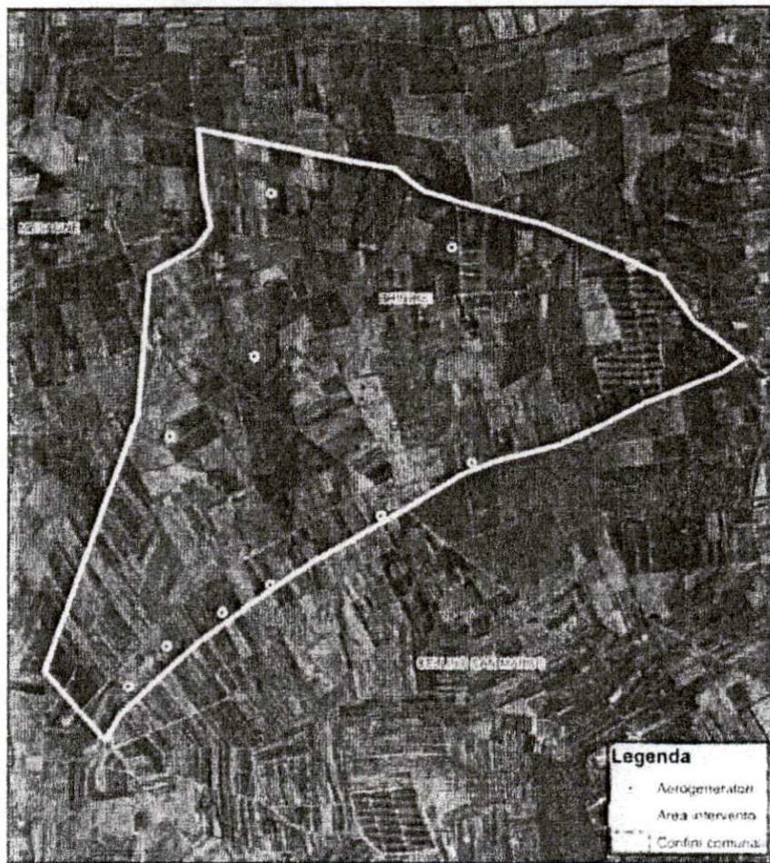
Fig. 2 - Individuazione aerogeneratori su ortofoto
