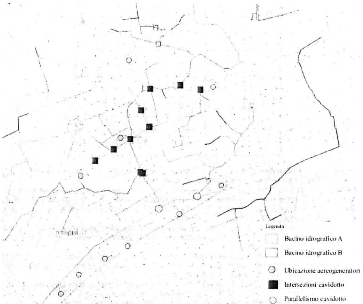
Fig. 7 – Interferenze rilevate tra il cavidotto MT in progetto e il reticolo idrografico rilevato
