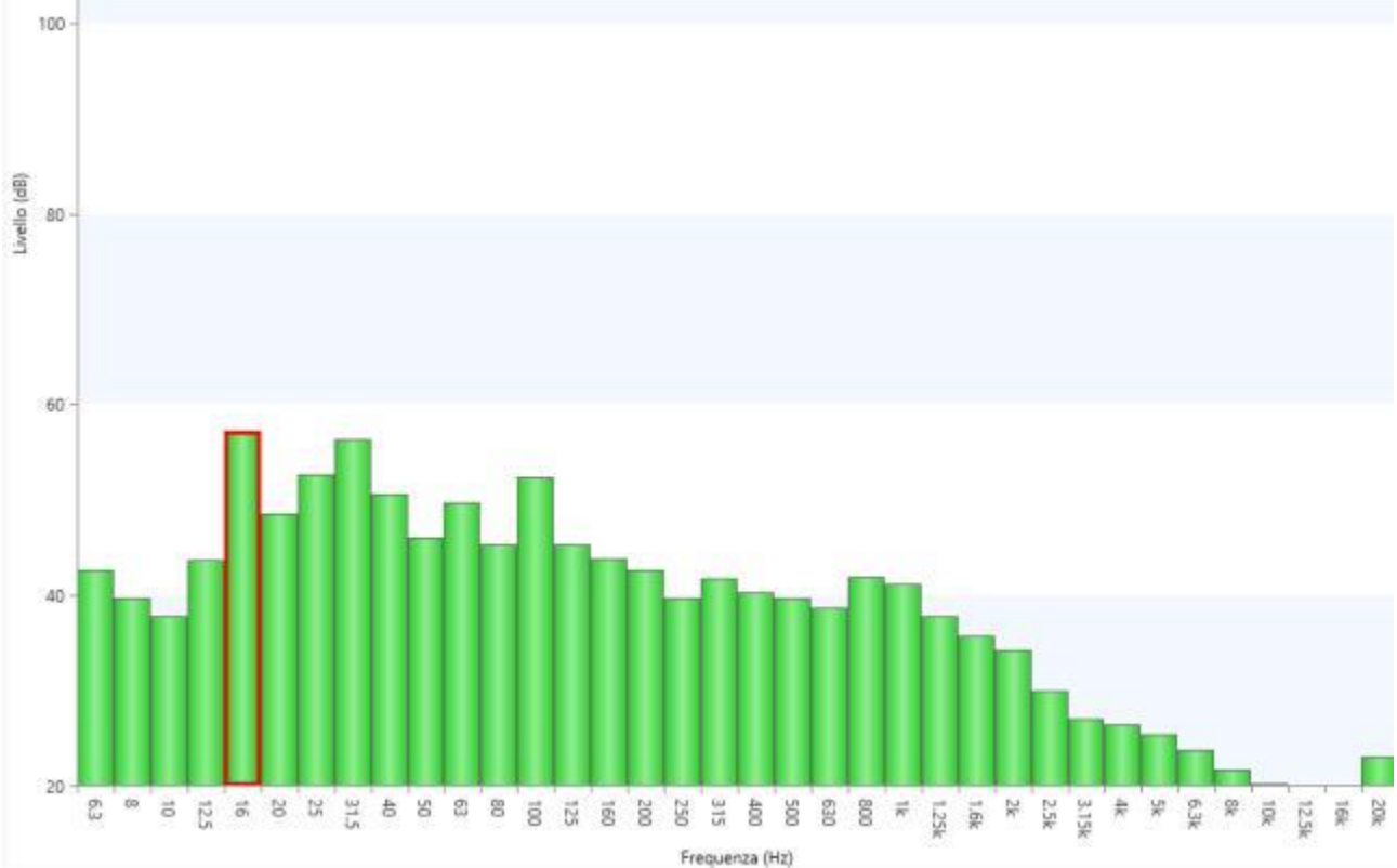
Figura 35 - Misura5: Spettro di frequenza in terzi d'ottave
