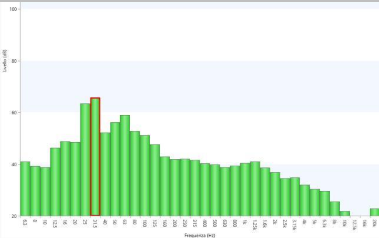
Figura 25 - Misura1: Spettro di frequenza in terzi d'ottave
