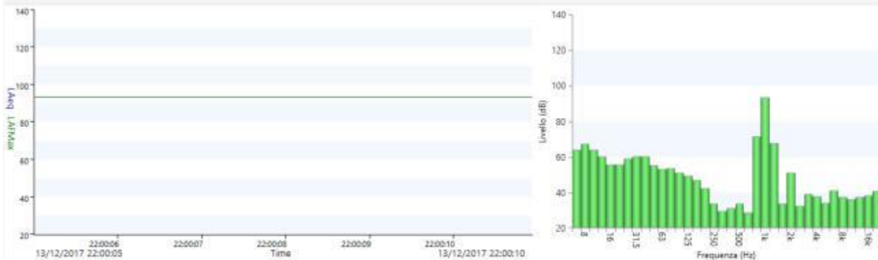
Figura 19 - Calibrazione INIZIALE del 13/12/2017
