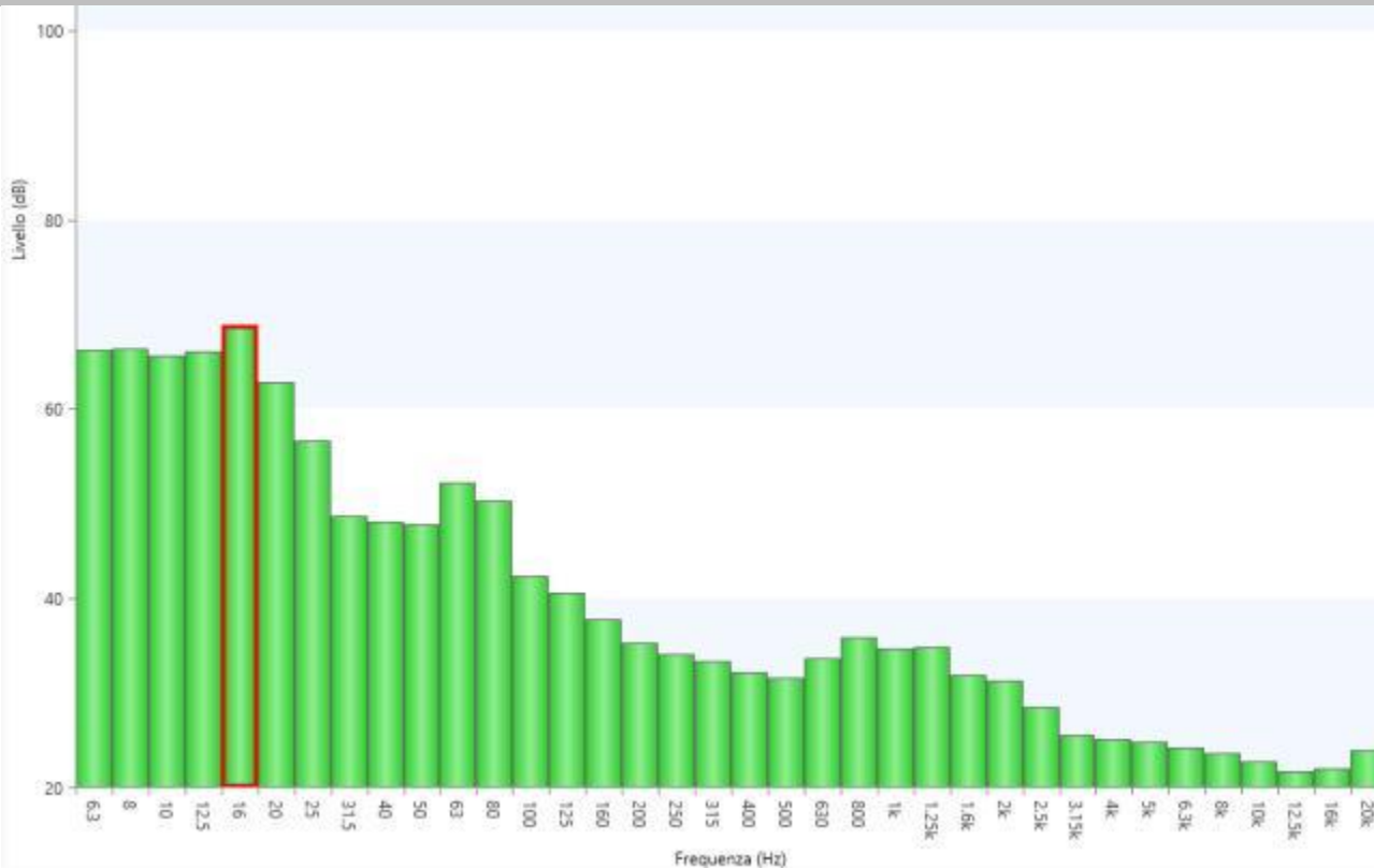
Figura 28 - Misura2: Spettro di frequenza in terzi d'ottave
