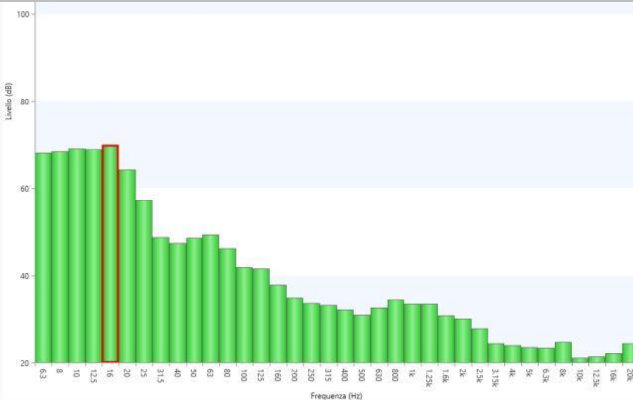
Figura 31 - Misura3: Spettro di frequenza in terzi d'ottave
