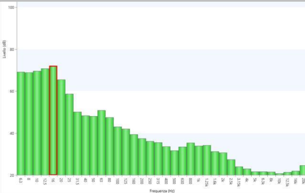
Figura 34 - Misura4: Spettro di frequenza in terzi d'ottave
