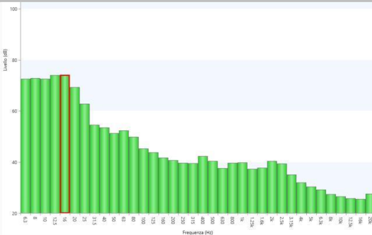
Figura 25 - Misura1: Spettro di frequenza in terzi d'ottave
