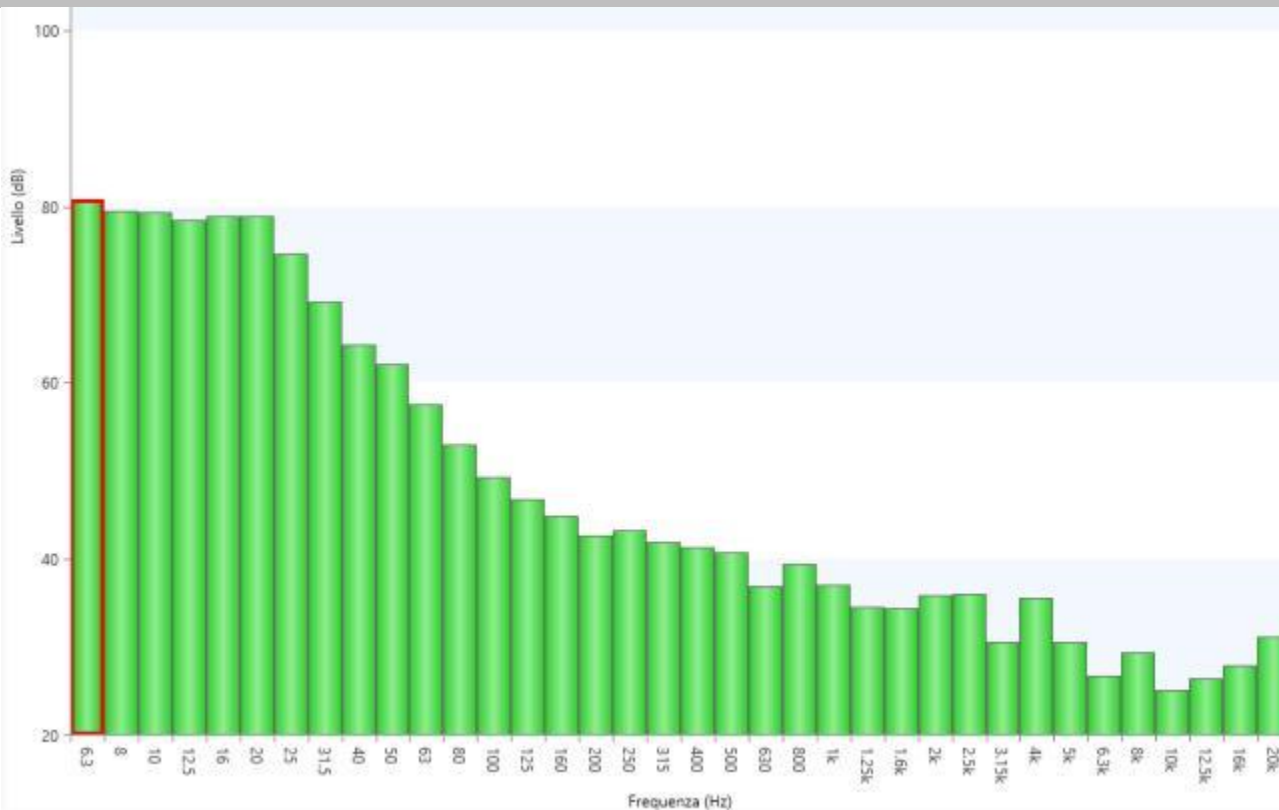
Figura 37 - Misura5: Spettro di frequenza in terzi d'ottave
