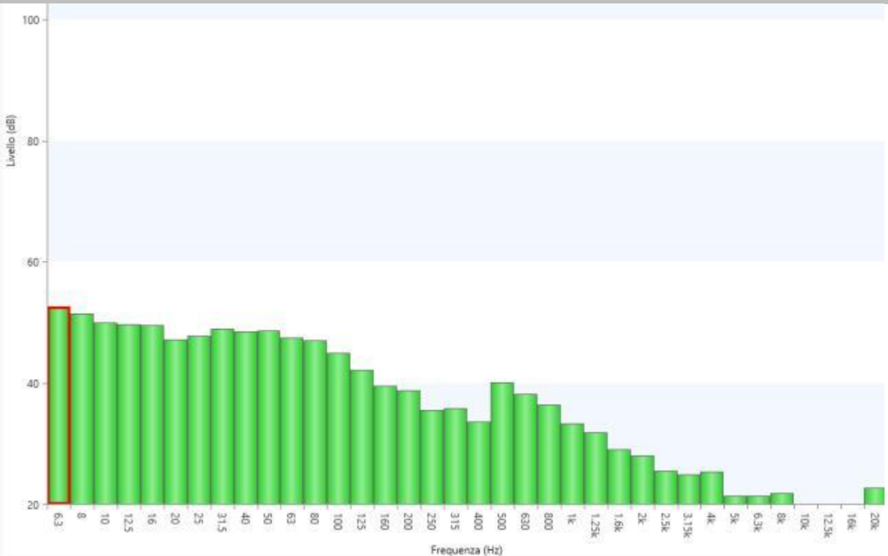
Figura 33 - Misura4: Spettro di frequenza in terzi d'ottave
