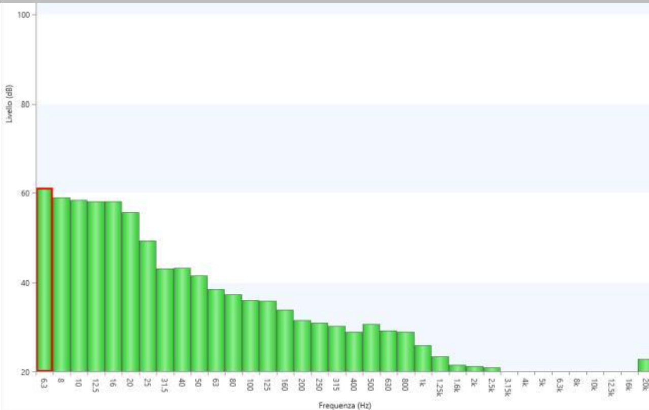
Figura 43 - Misura7: Spettro di frequenza in terzi d'ottave
