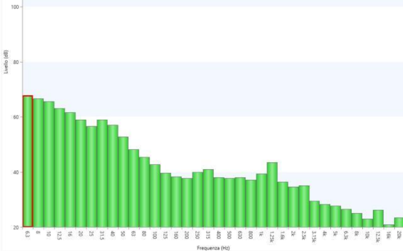
Figura 28 - Misura2: Spettro di frequenza in terzi d'ottave
