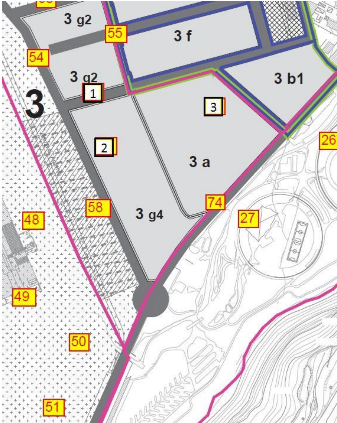
Figura 8 - Localizzazione delle postazioni di misura
