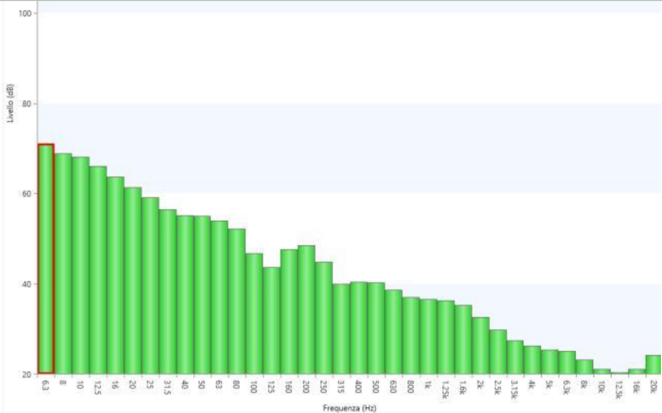
Figura 23 - Misura1: Spettro di frequenza in terzi d'ottave
