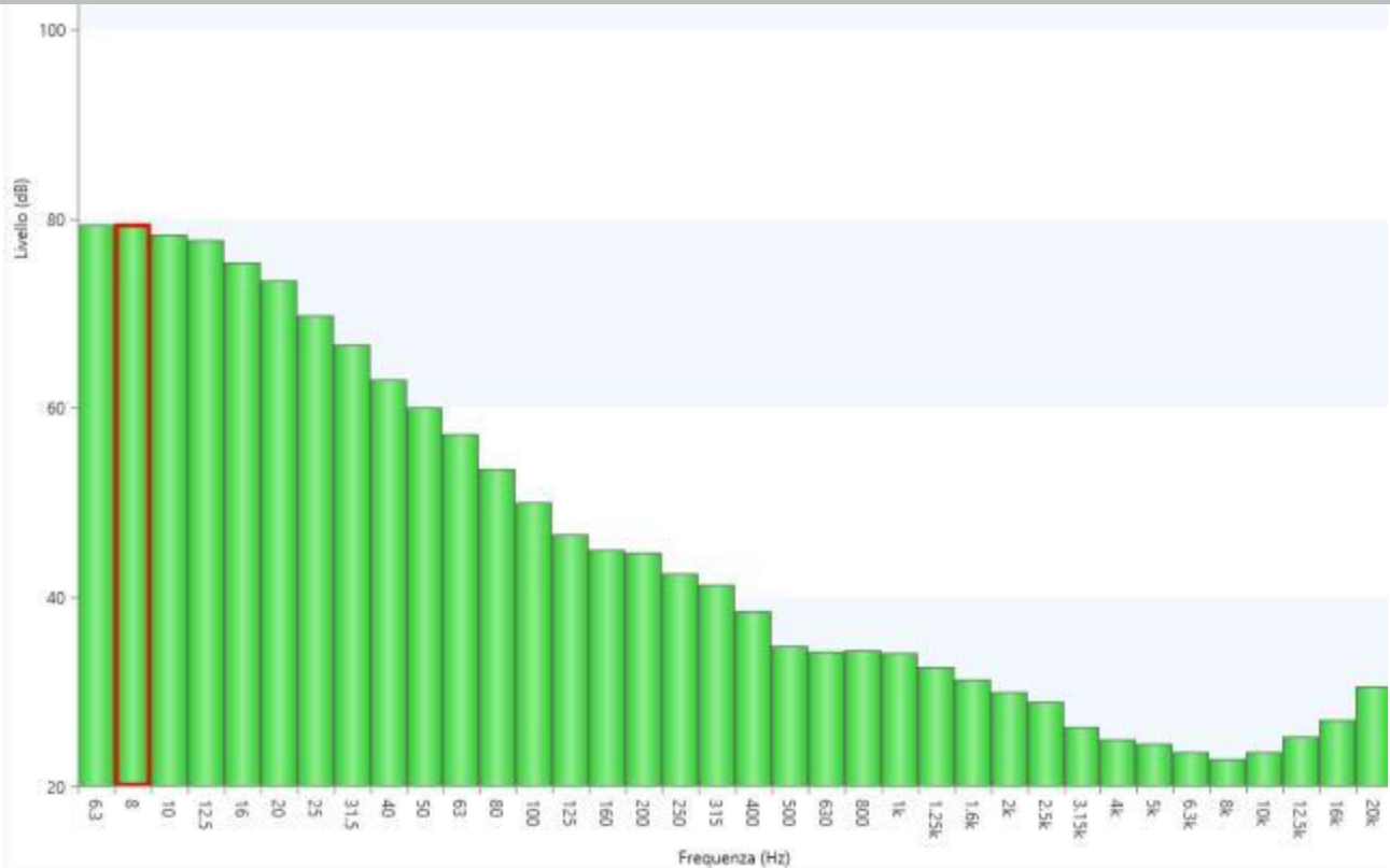
Figura 29 - Misura3: Spettro di frequenza in terzi d'ottave
