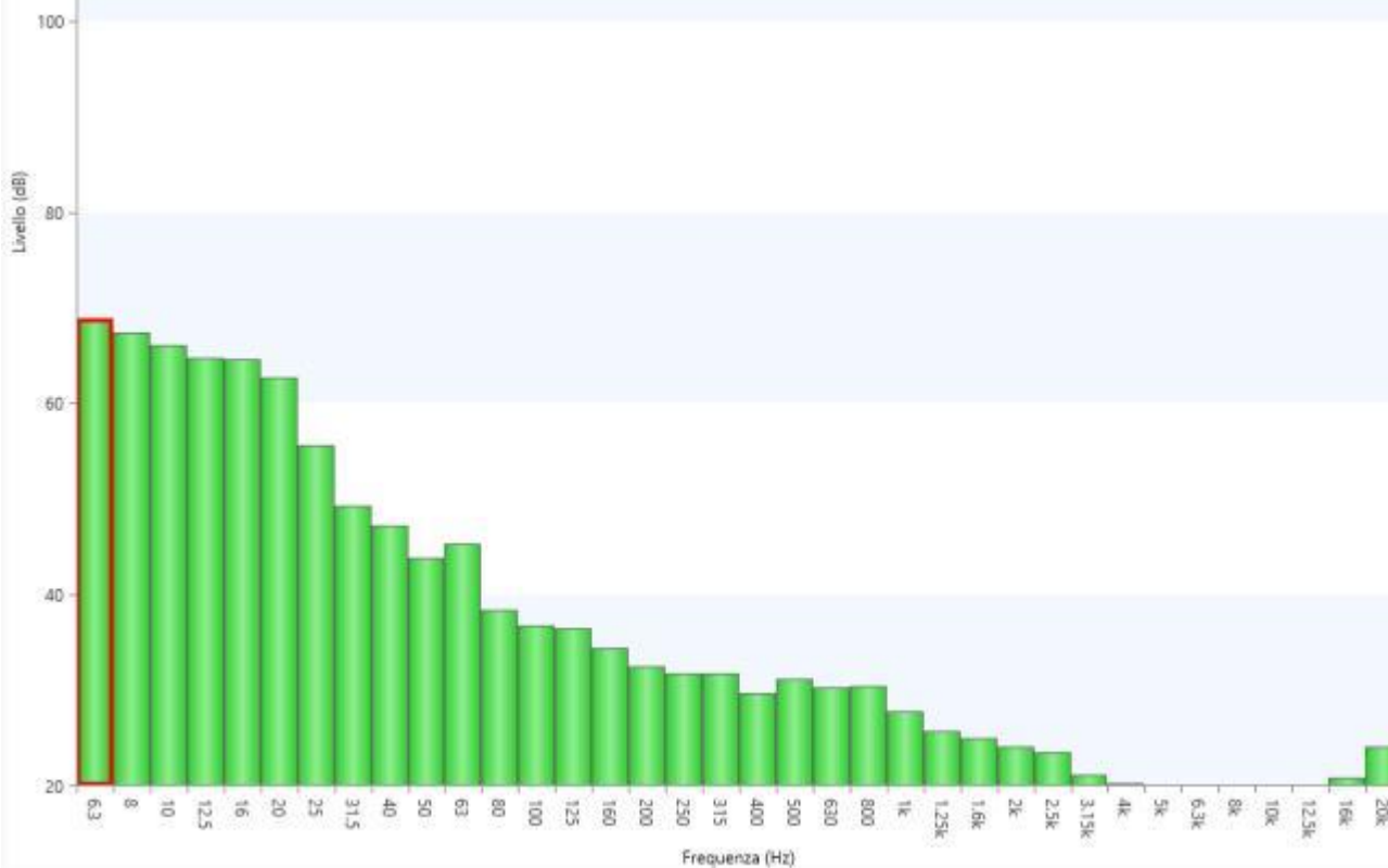
Figura 52 - Misura8: Spettro di frequenza in terzi d'ottave
