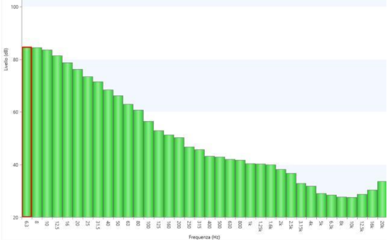
Figura 24 - Misura1: Spettro di frequenza in terzi d'ottave
