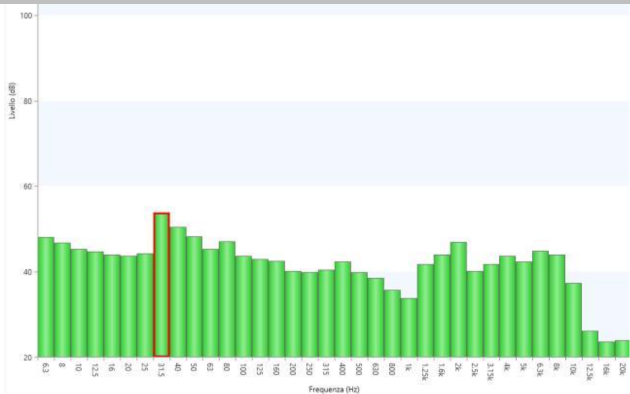
Figura 39 - Misura6: Spettro di frequenza in terzi d'ottave
