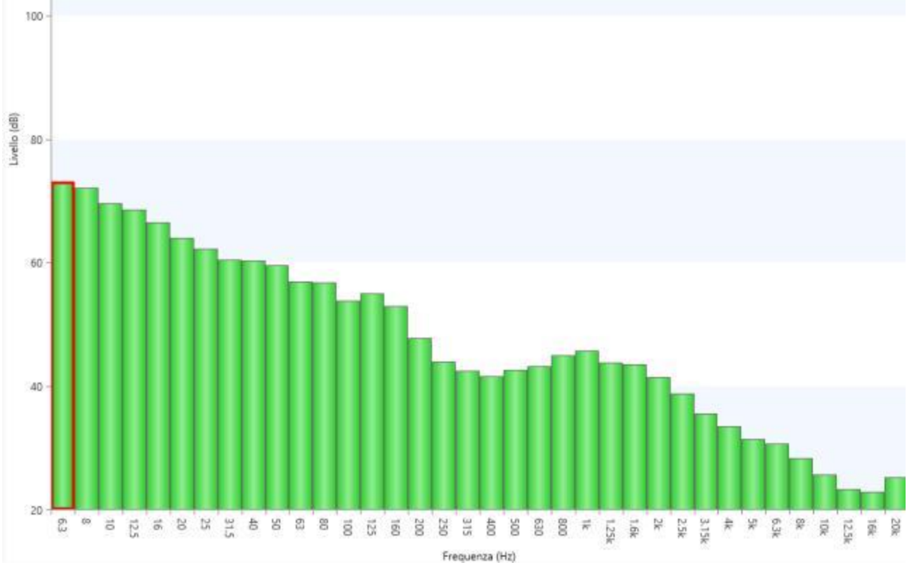
Figura 27 - Misura2: Spettro di frequenza in terzi d'ottave
