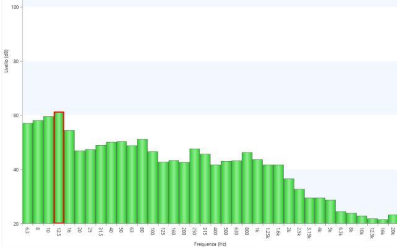
Figura 36 - Misura5: Spettro di frequenza in terzi d'ottave
