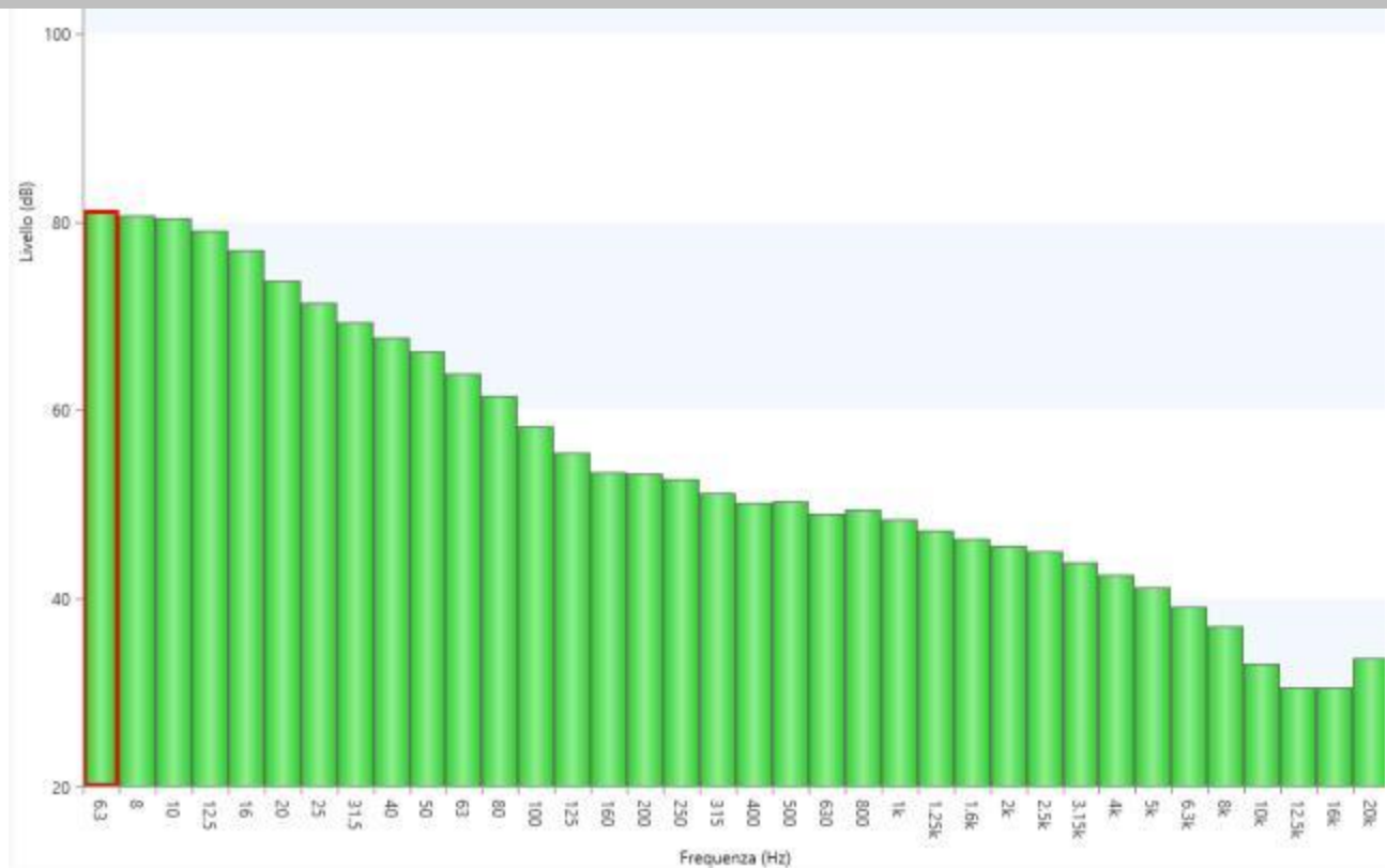
Figura 30 - Misura3: Spettro di frequenza in terzi d'ottave
