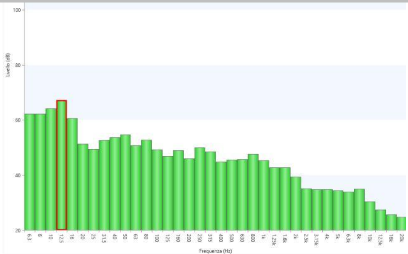
Figura 32 - Misura4: Spettro di frequenza in terzi d'ottave
