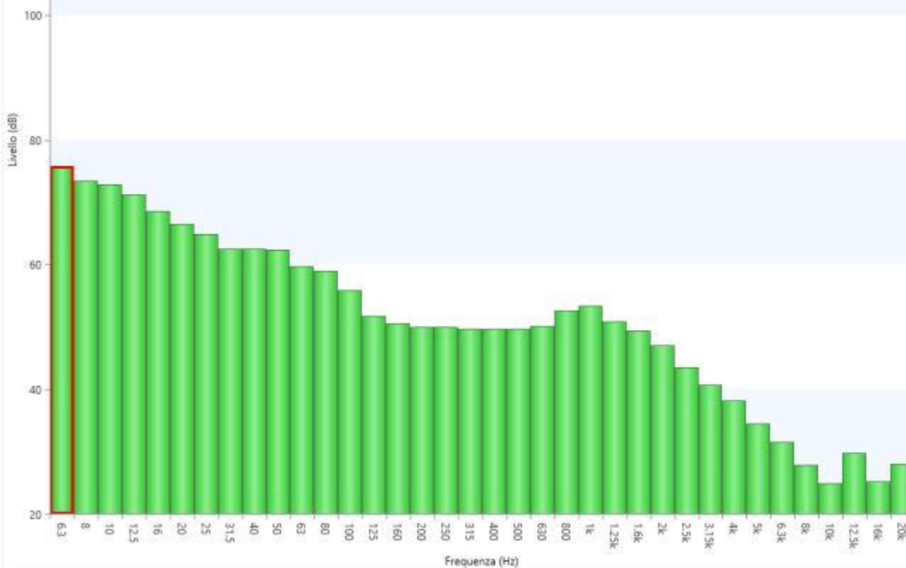
Figura 39 - Misura6: Spettro di frequenza in terzi d'ottave
