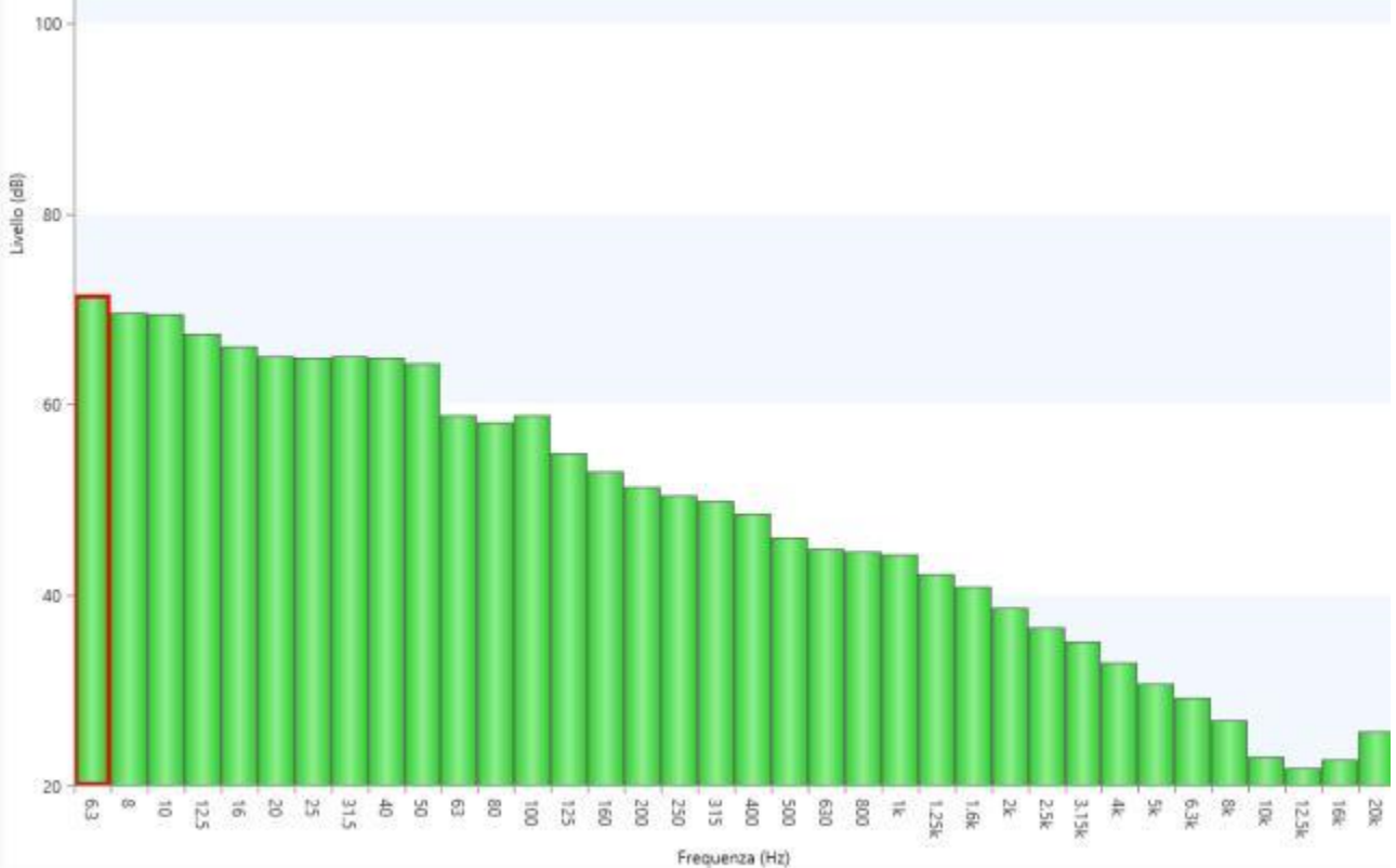
Figura 26 - Misura2: Spettro di frequenza in terzi d'ottave
