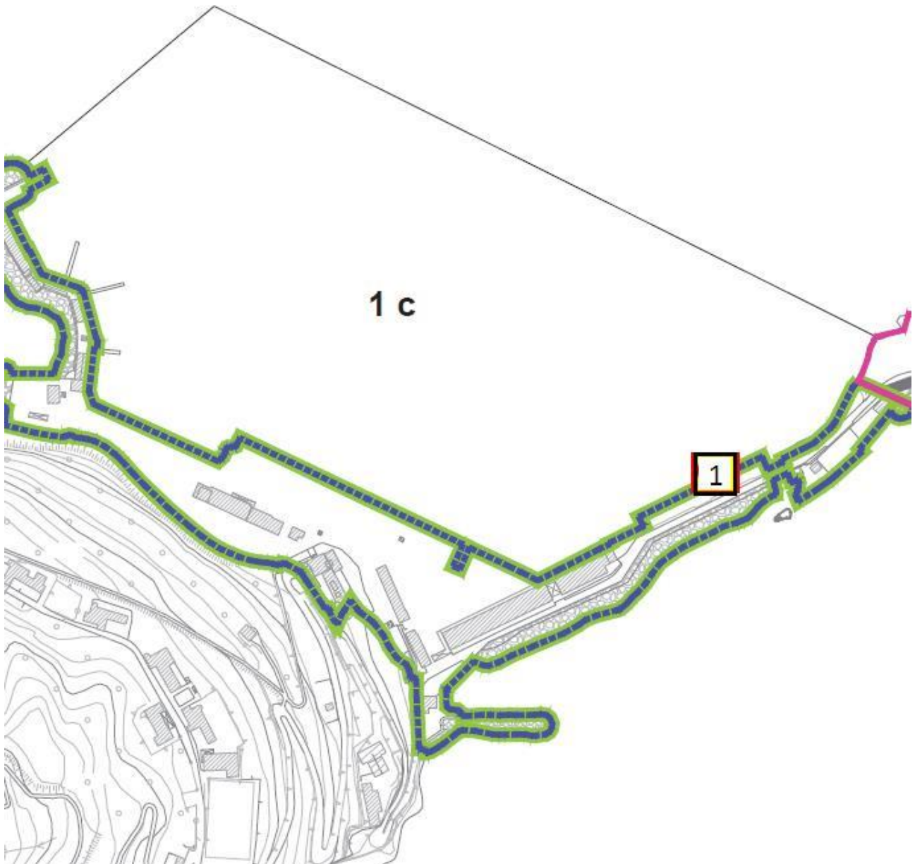
Figura 8 - Localizzazione delle postazioni di misura
