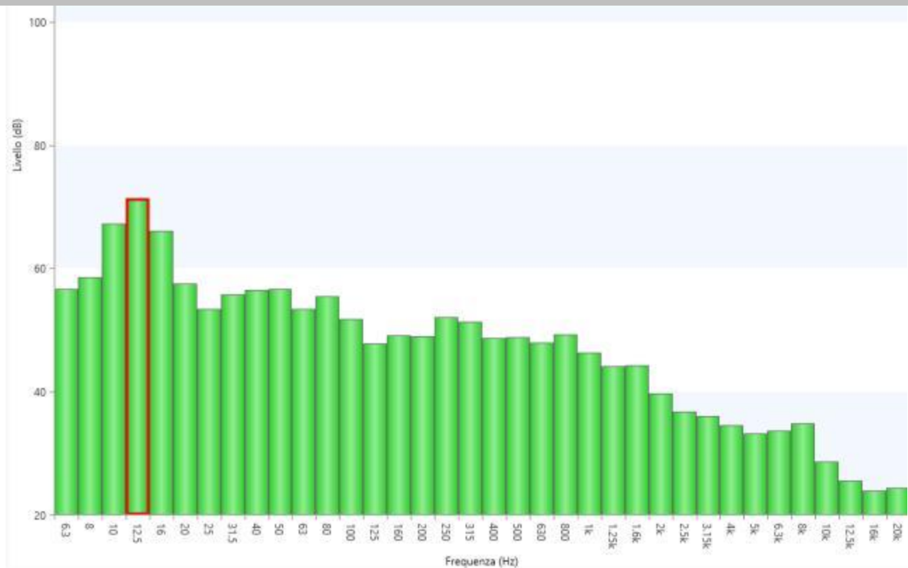
Figura 40 - Misura3: Spettro di frequenza in terzi d'ottave
