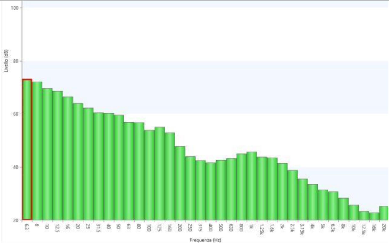
Figura 34 - Misura3: Spettro di frequenza in terzi d'ottave
