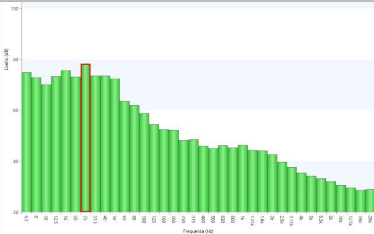
Figura 28 - Misura1: Spettro di frequenza in terzi d'ottave
