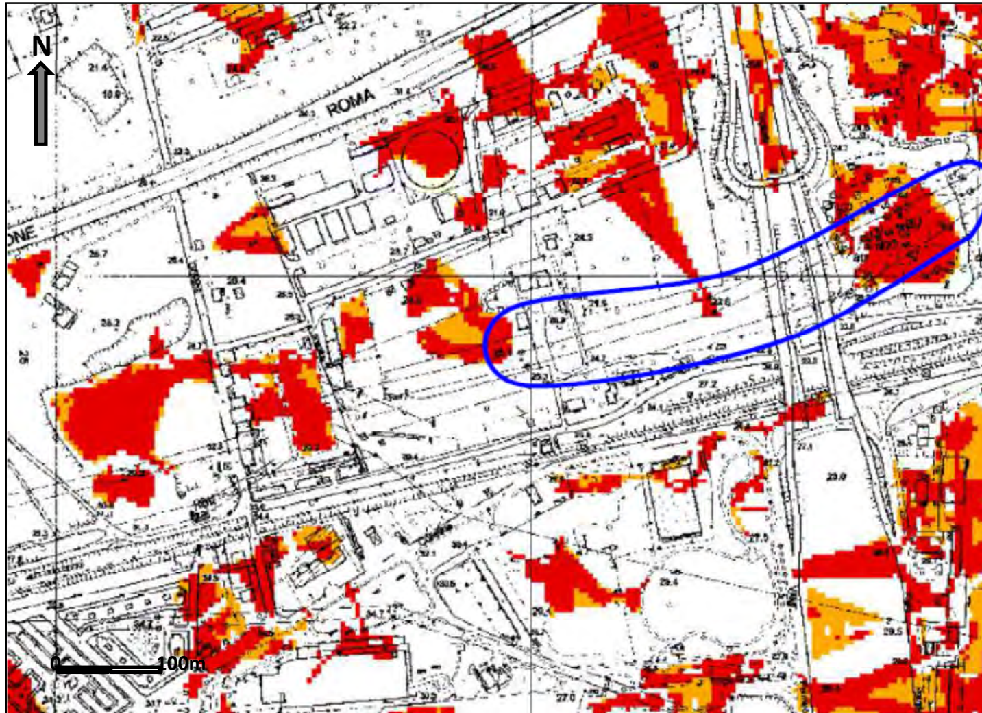
Localizzazione del progetto in riferimento tavola 18 della P3 del PS5 - aree a pericolosità idraulica potenziale. Fonte: Piano di Bacino -Piano di Stralcio PS5 Scala 1:5000 - Formato A4.
