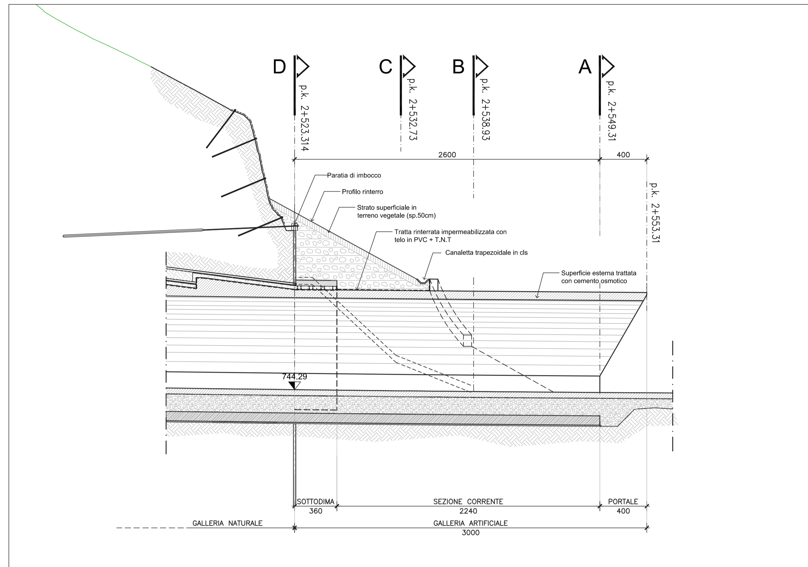
IMBOCCO EST - PROFILO OPERE DEFINITIVE
