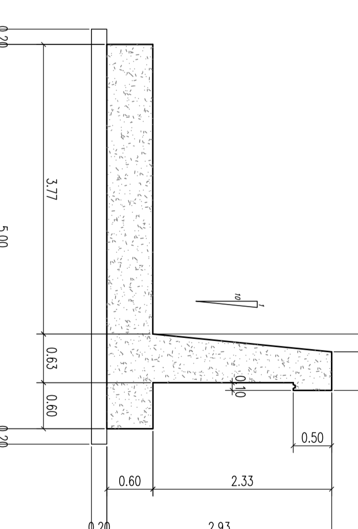
SEZIONE F-F SCALA 1:50
