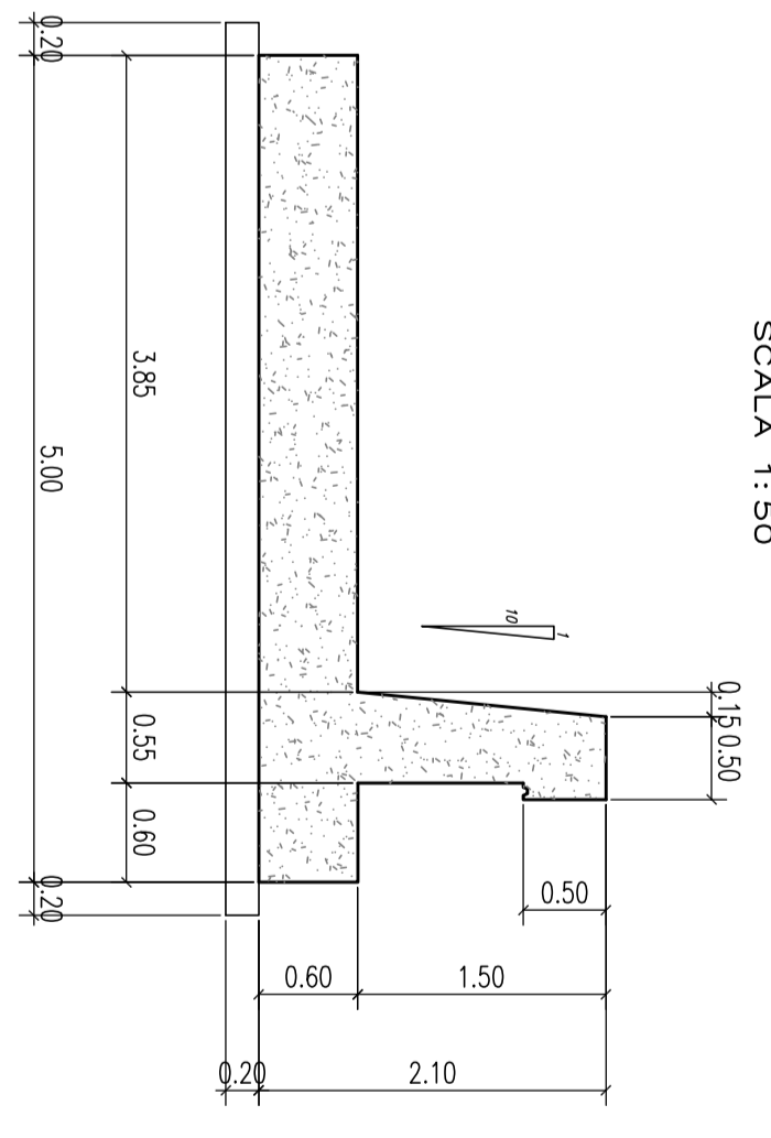
SEZIONE D-D SCALA 1:50
