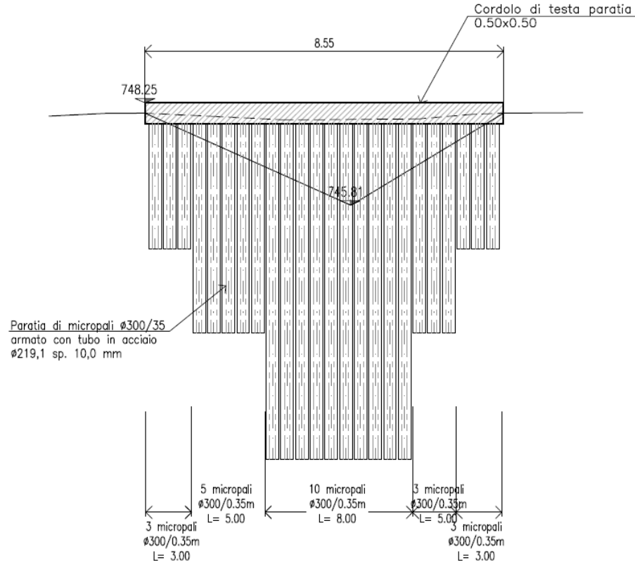
Figura 2.1 – Sviluppata paratia Spalla A – Viadotto Cant
