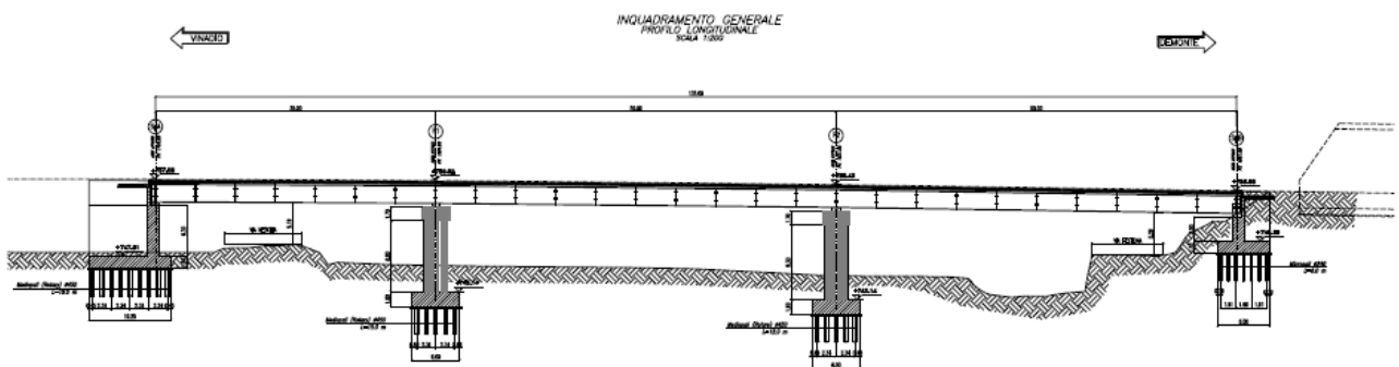
Prospetto Viadotto Cant
