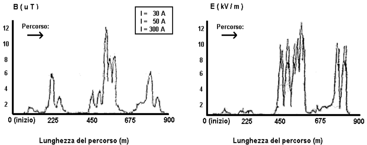
Figure 2: Risultati della misura dei campi elettrici e magnetici effettuate lungo le vie interne della sezione a 380 kV della stazione riportata in fig. 1
