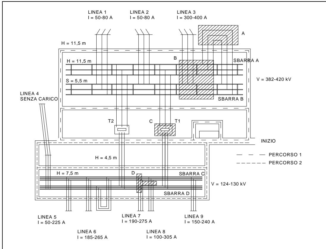
Figure 1: Pianta di una tipica stazione 380/132 kV con l'indicazione delle principali distanze fase-fase (S) e fase-terra (H) e delle variazioni delle tensioni e delle correnti durante la fasi di misurazioni di campo elettrico e magnetico
