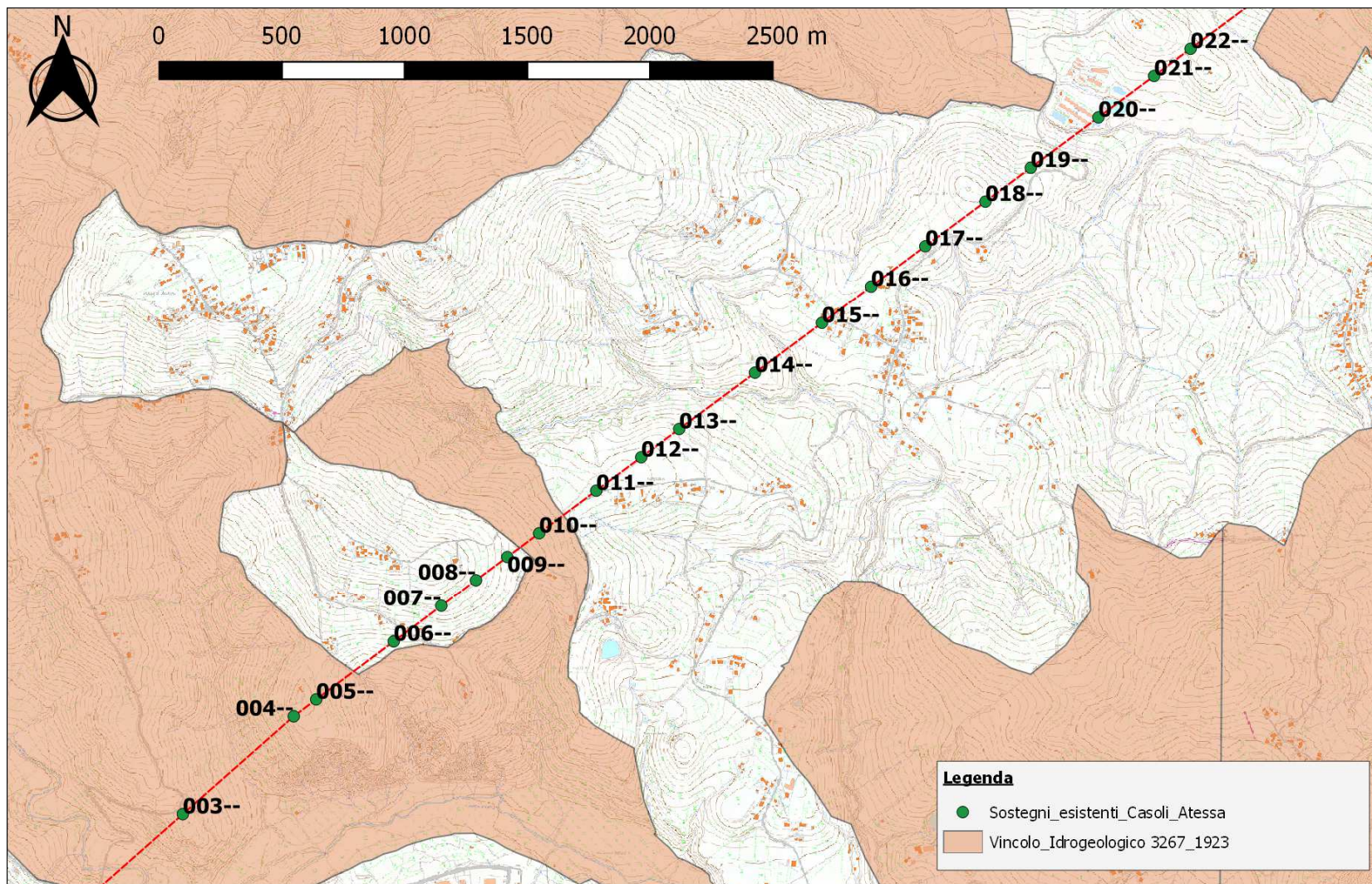
Carta di localizzazione delle opere di progetto e vincolo idrogeologico R.D. 3267/1923. Scala 1:25000
