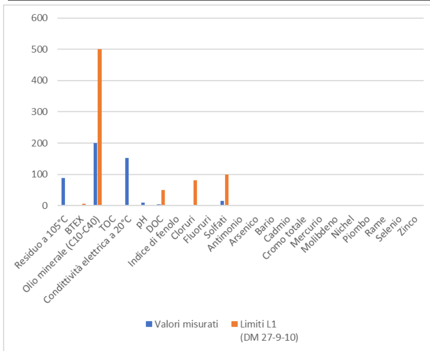
Figura 19 - Risultati test eluato secondo il DM 05-02-1998 campione SI-2.
