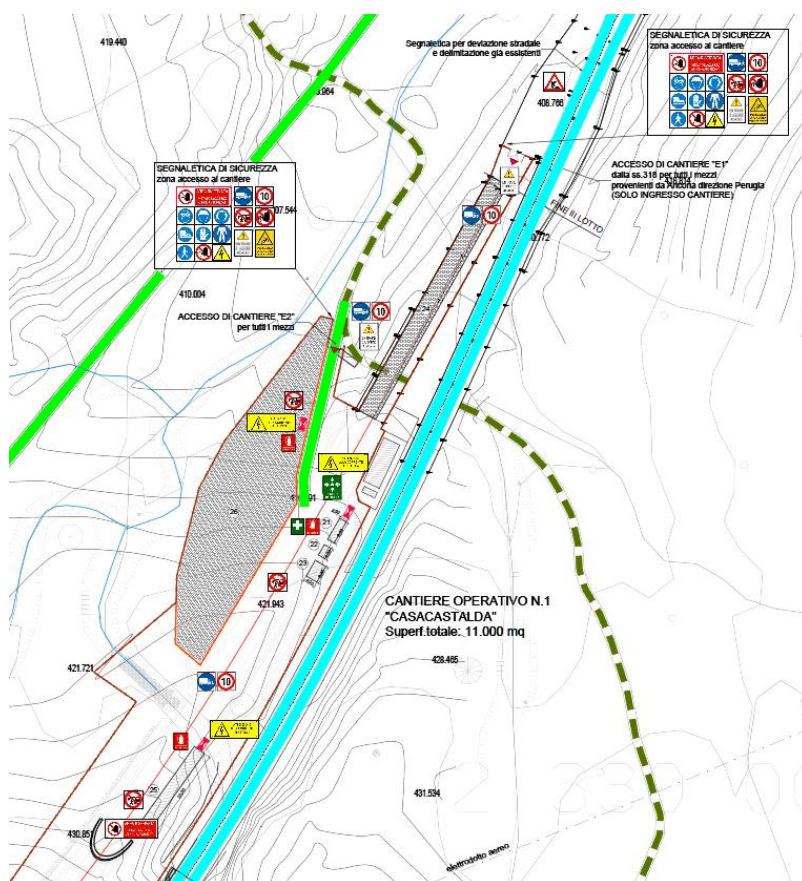
Figura 29 – Planimetria cantiere "Casacastalda"
