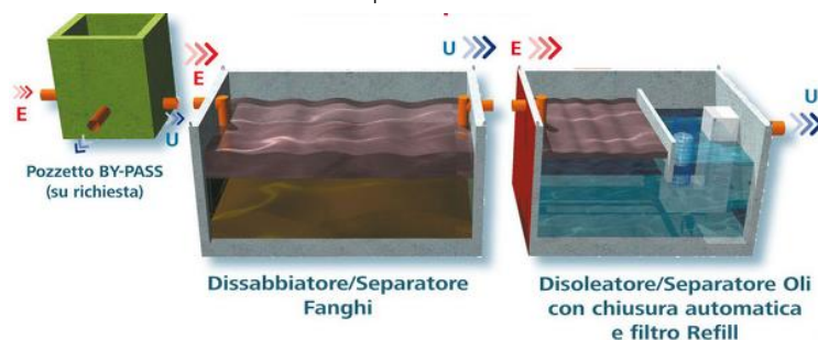
Figura 31 - Schema impianto in continuo.
