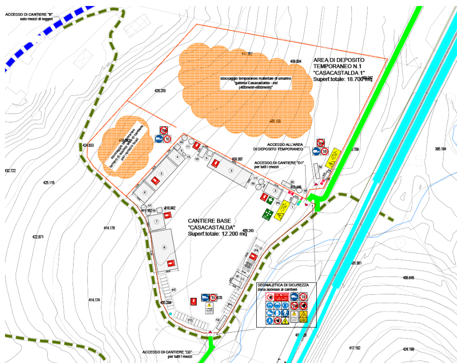
Figura 28 - Planimetria cantiere base "Casacastalda".
