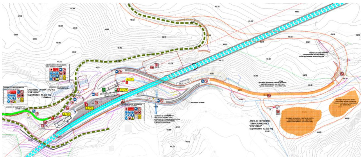
Figura 5 - Planimetria cantiere operativo "Calvario".
