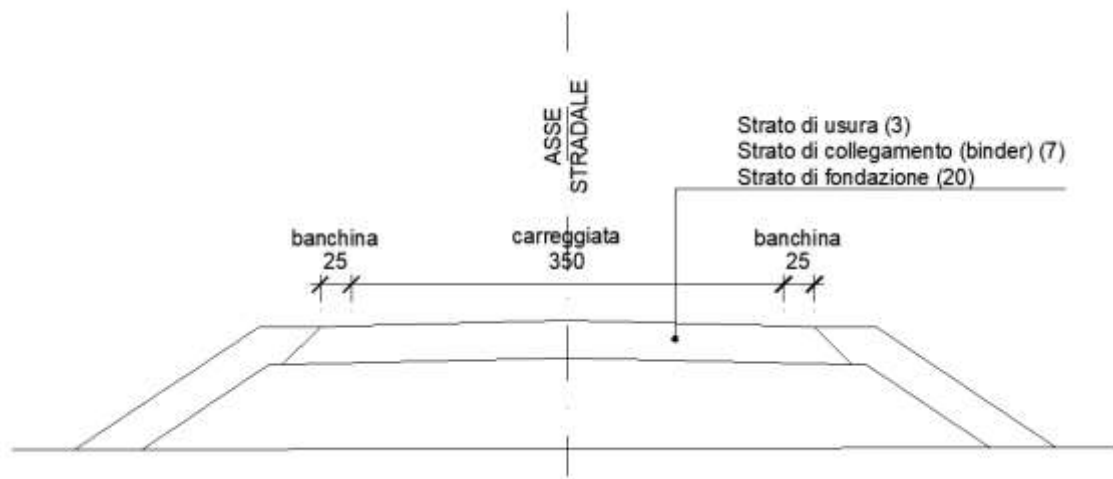
Figura 1: Sezione tipologica
