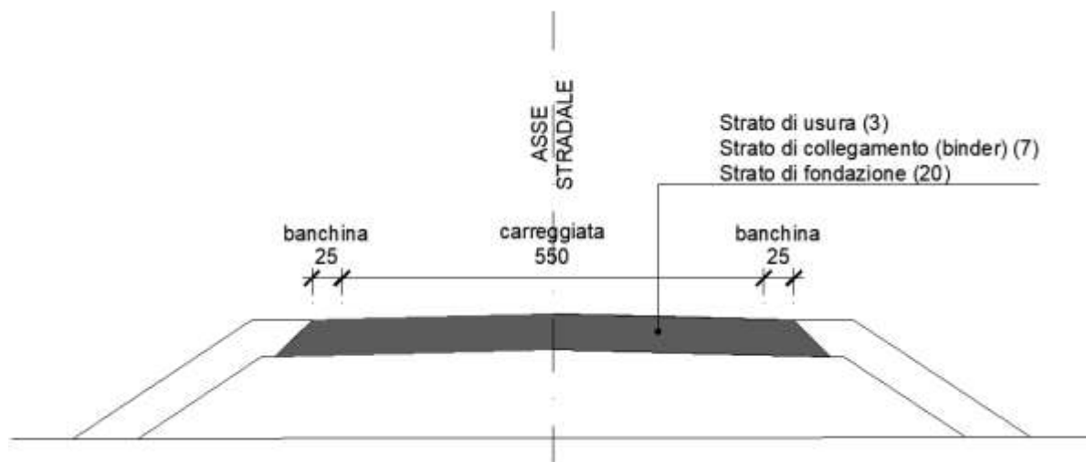
Figura 1: Sezione tipologica
