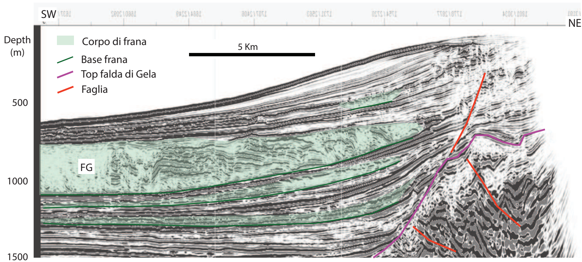
ALLEGATO 5 Sezione geologica dell'AREA-3 sulla sea-line
