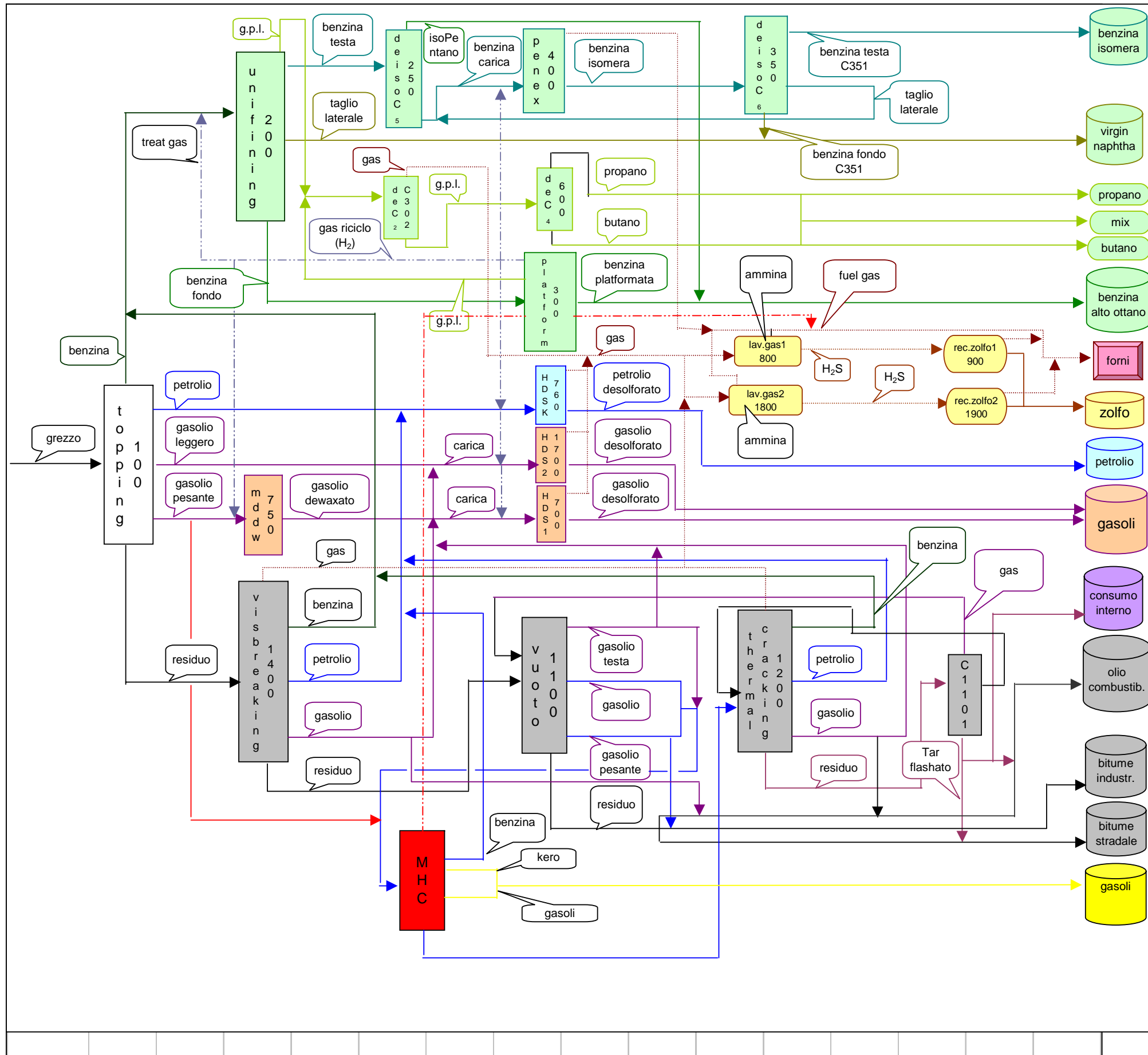
A.25 - SCHEMA GENERALE DELLA RAFFINERIA A BLOCCHI
