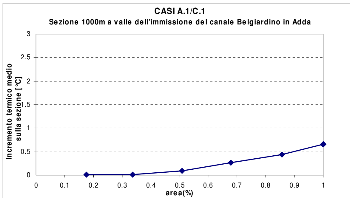
fig. 6.27 – Casi A.1 e C.1. Andamento dell’incremento termico medio nella sezione a 1000 m in funzione della percentuale di area
