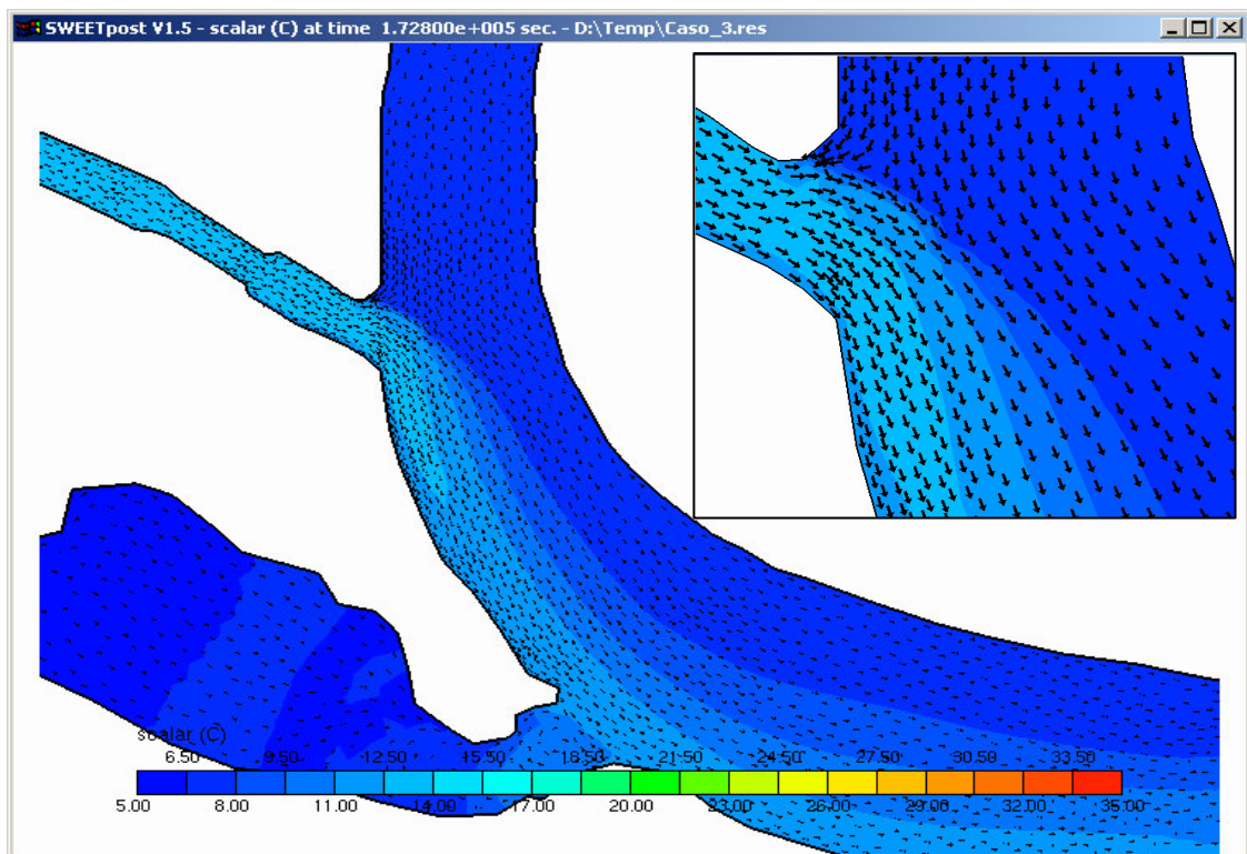
fig. 6.14 – Caso B.3. Campo termico e campo di moto nella zona della confluenza del Belgiardino in Adda
