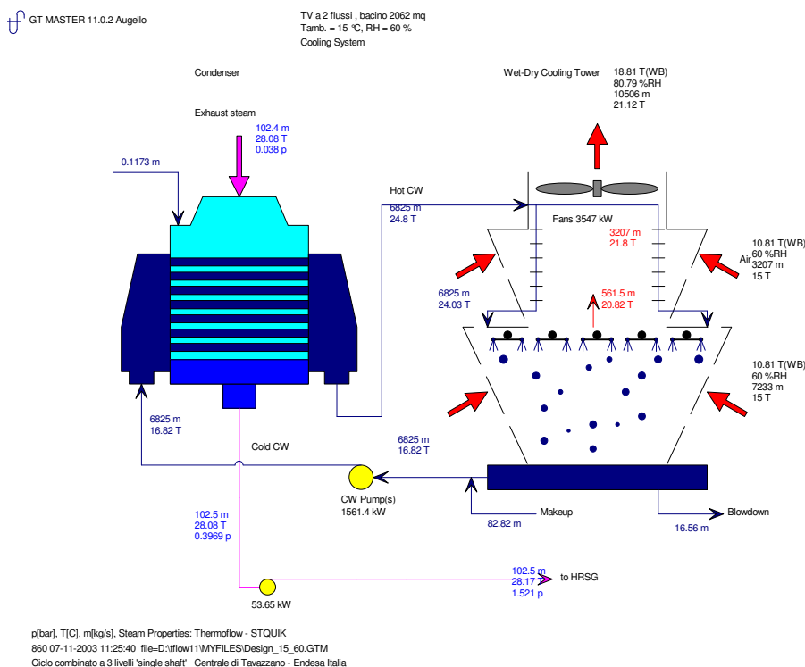
fig. 3.2 – Schema funzionale della torre di raffreddamento wet-dry per il modulo 9
