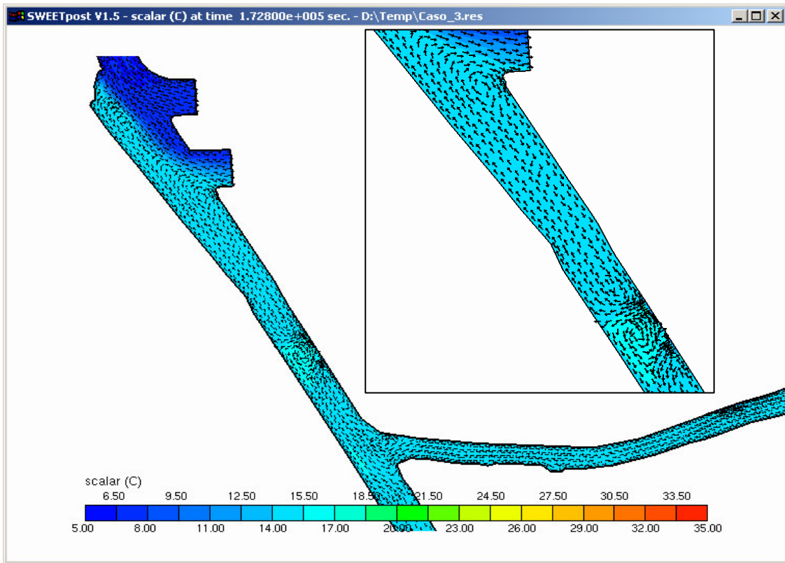
fig. 6.13 – Caso B.3. Campo termico e campo di moto nella zona delle opere di scarico e presa
