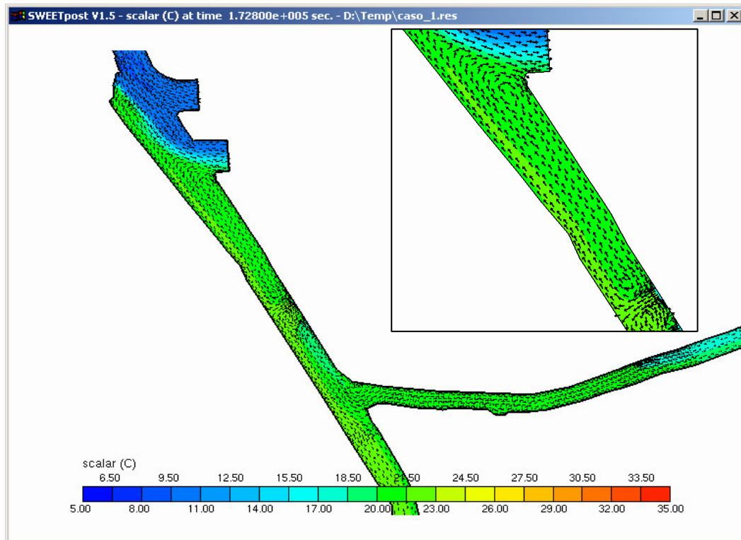
fig. 6.1 – Caso B.1. Campo termico e campo di moto nella zona delle opere di scarico e presa
