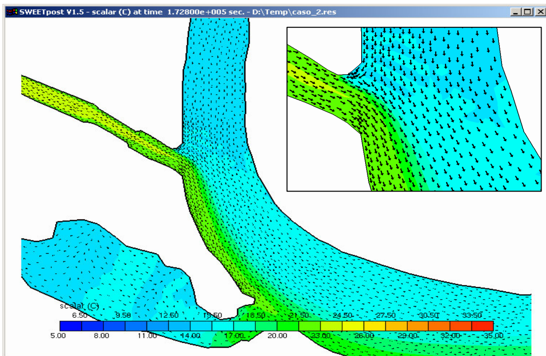
fig. 6.8 – Caso B.2. Campo termico e campo di moto nella zona della confluenza del Belgiardino in Adda
