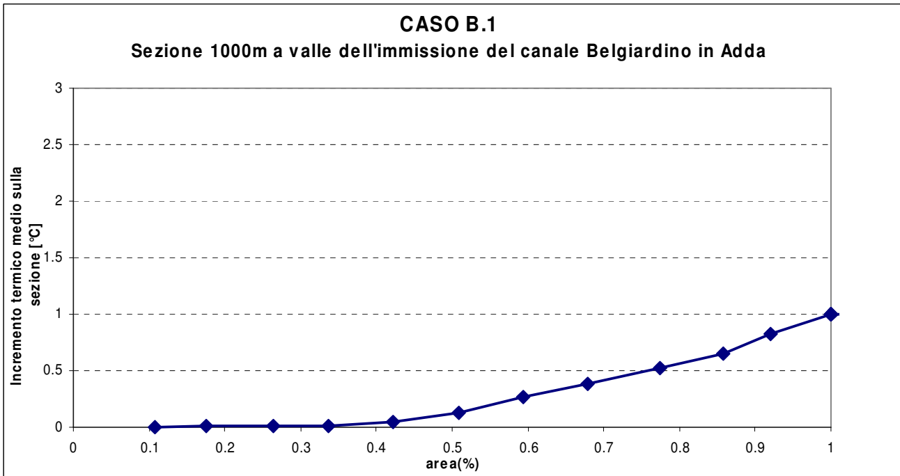
fig. 6.5 – Caso B.1. Andamento dell'incremento termico medio nella sezione a 1000 m in funzione della percentuale di area
