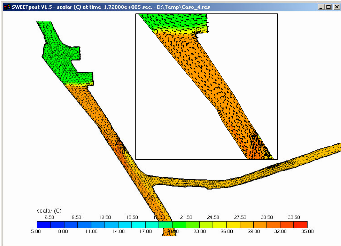
fig. 6.19 – Caso B.4. Campo termico e campo di moto nella zona delle opere di scarico e presa
