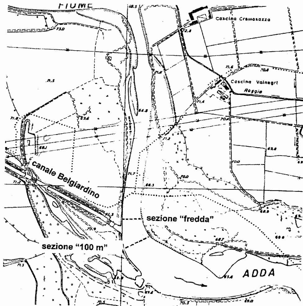
fig. 4.1- Collocazione delle sezioni di valutazione della perturbazione termica
