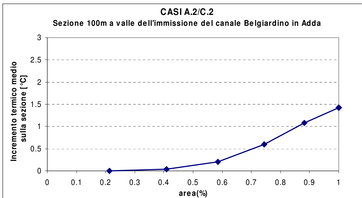
fig. 6.29 – Casi A.2 e C.2. Andamento dell'incremento termico medio nella sezione a 100 m in funzione della percentuale di area
