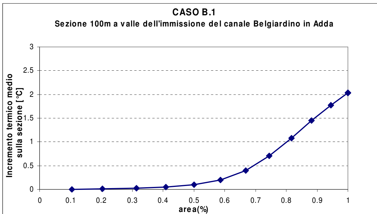
fig. 6.3 – Caso B.1. Andamento dell'incremento termico medio nella sezione a 100 m in funzione della percentuale di area
