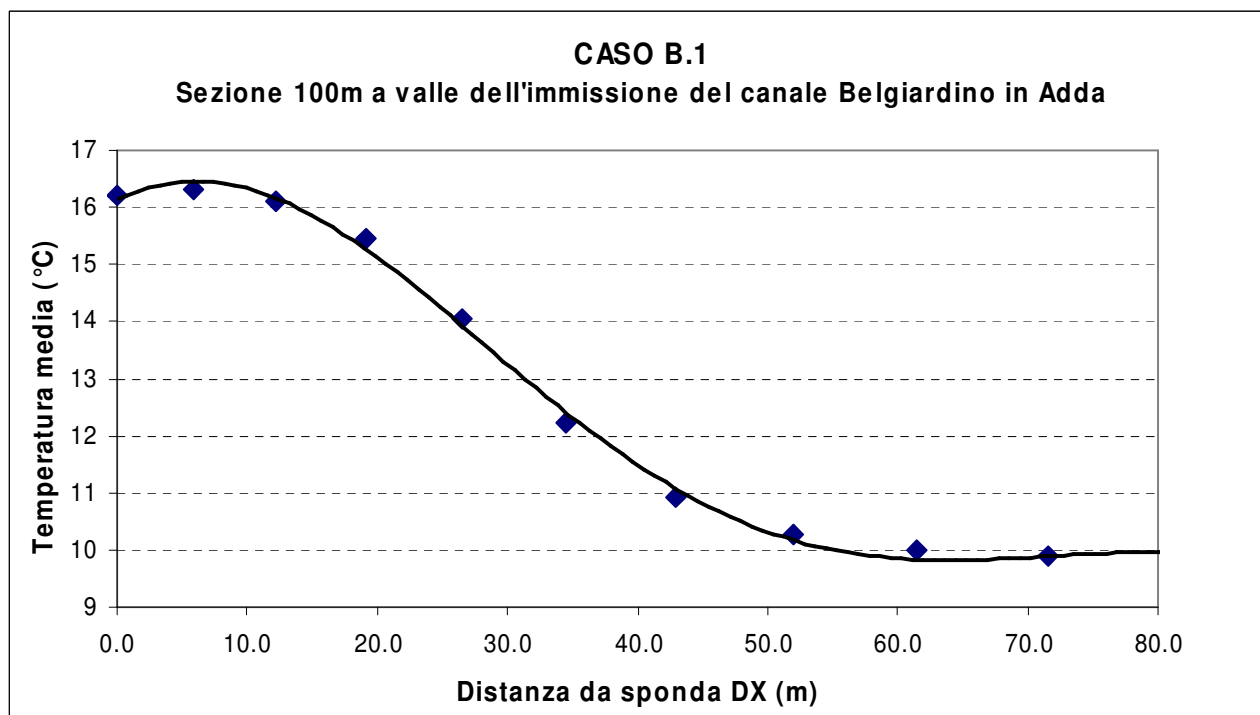
fig. 6.4 – caso B.1. Andamento della temperatura media nella sezione a 100 m
