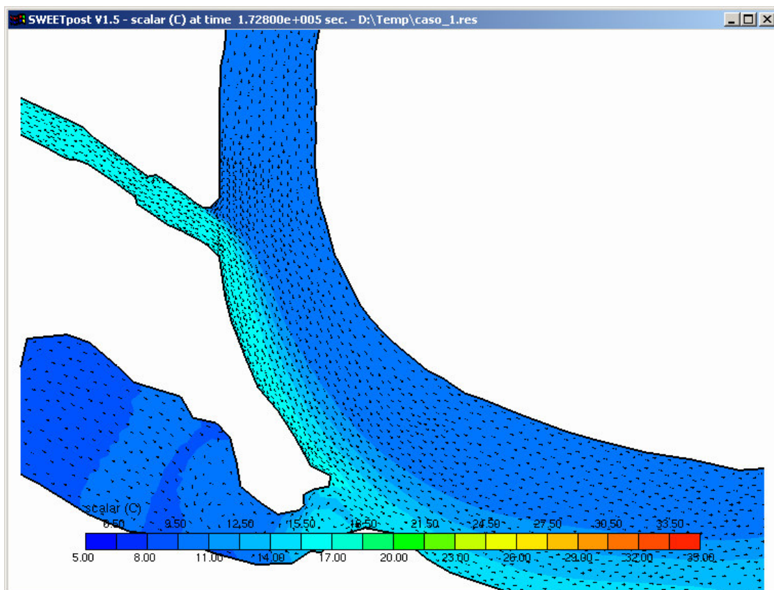
fig. 6.2 – Caso B.1. Campo termico e campo di moto nella zona della confluenza del Belgiardino in Adda
