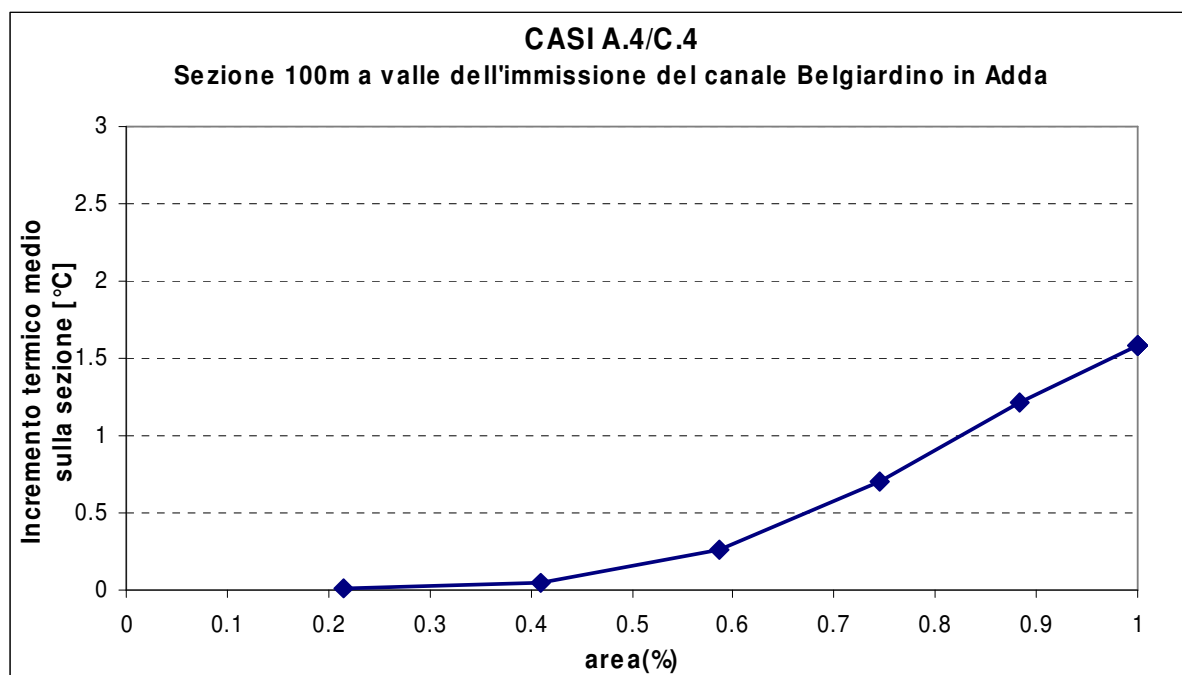
fig. 6.37 – Casi A.4 e C.4. Andamento dell'incremento termico medio nella sezione a 100 m in funzione della percentuale di area
