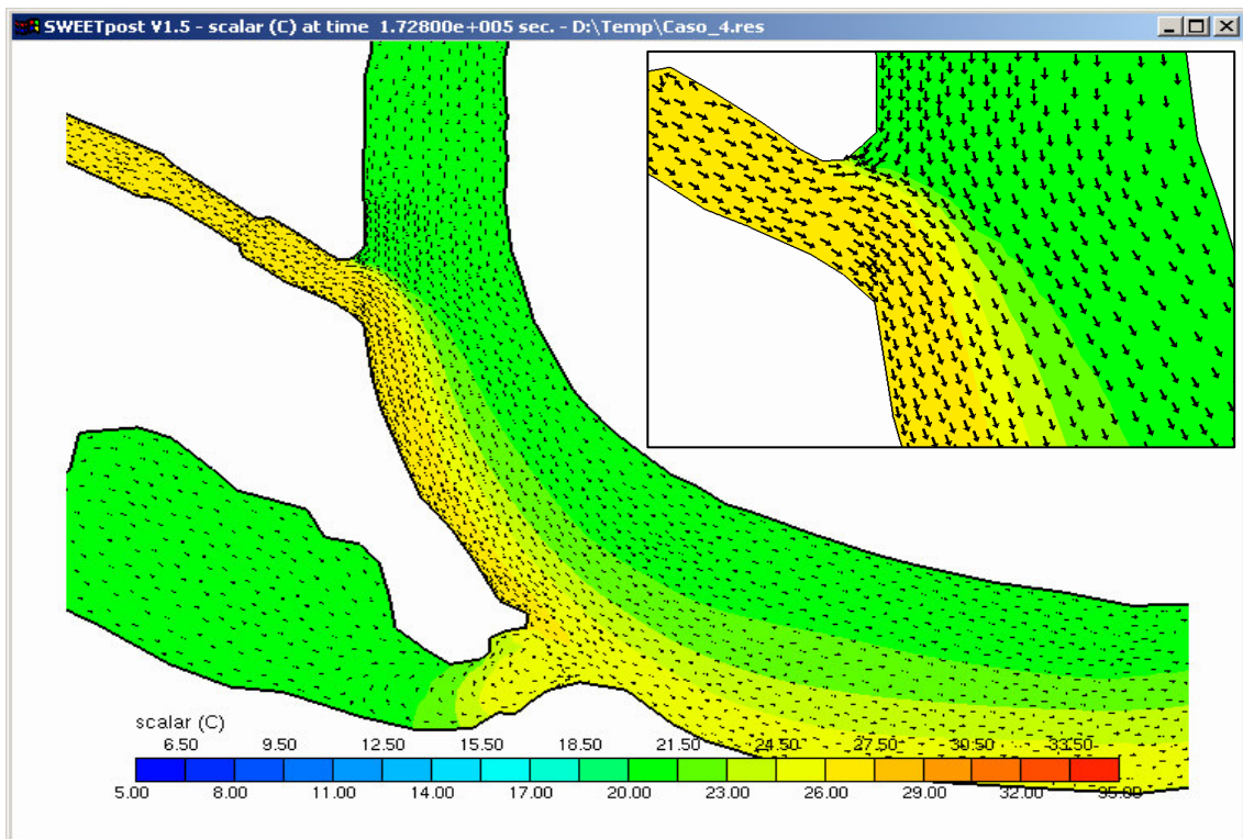
fig. 6.20 – Caso B.4. Campo termico e campo di moto nella zona della confluenza del Belgiardino in Adda
