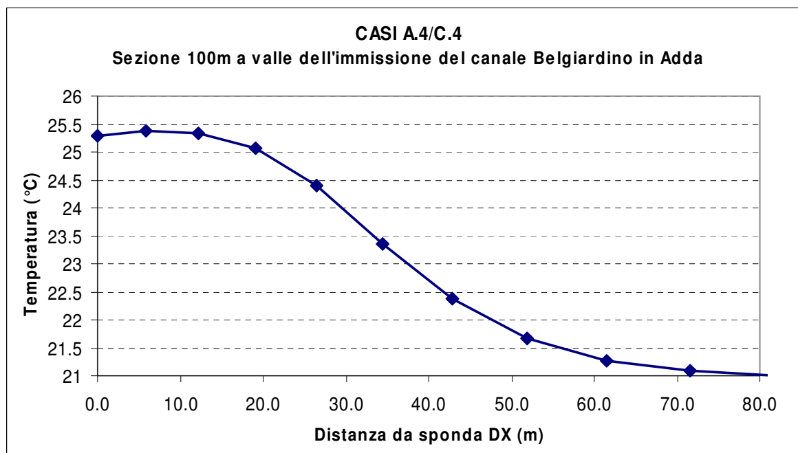
fig. 6.38 – Casi A.4 e C.4. Andamento della temperatura media nella sezione a 100 m
