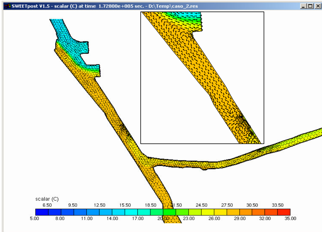
fig. 6.7 – Caso B.2. Campo termico e campo di moto nella zona delle opere di scarico e presa
