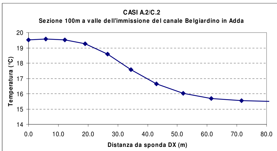
fig. 6.30 – Casi A.2 e C.2. Andamento della temperatura media nella sezione a 100 m
