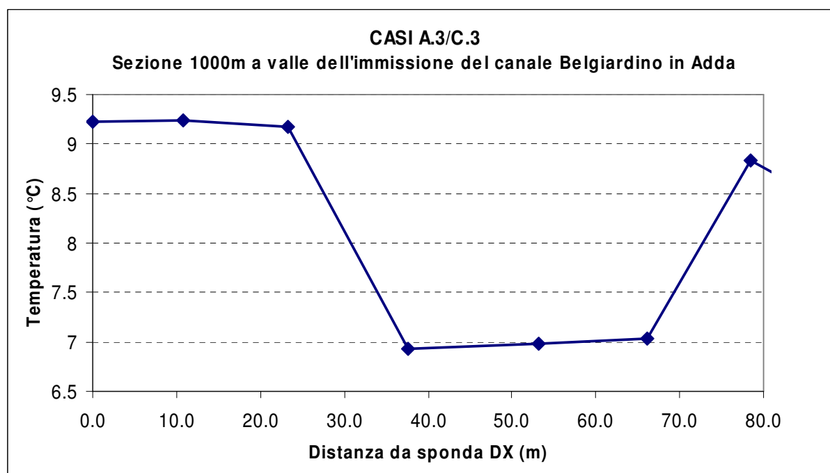
fig. 6.36 – Casi A.3 e C.3. Andamento della temperatura media nella sezione a 1000 m
