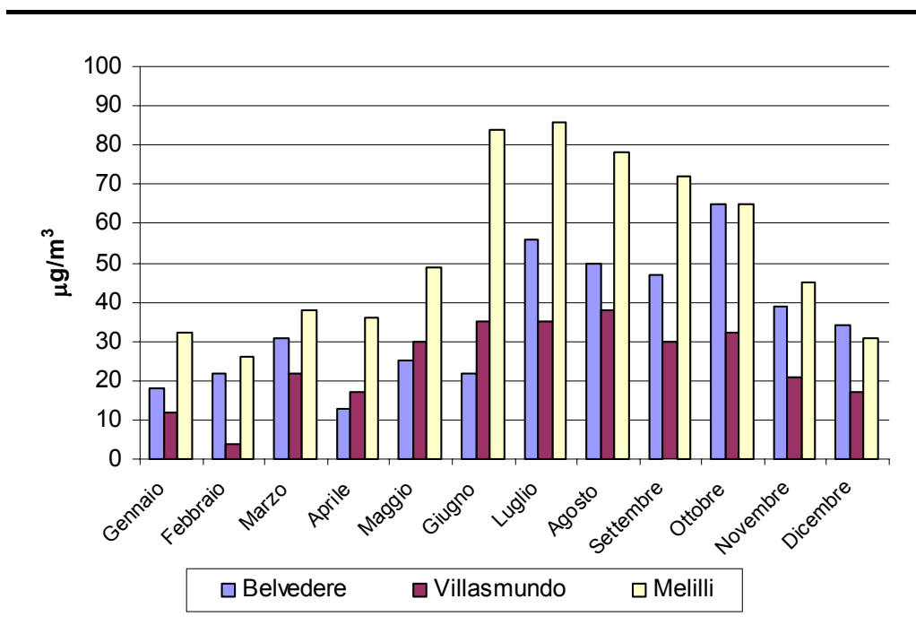
Figura 2.2.2.5a Concentrazioni Medie Mensili di NMHC ( \mu\text{g}/\text{m}^3 ) Rilevate nel 2005 alle Stazioni di Belvedere, Villasmundo, Melilli
