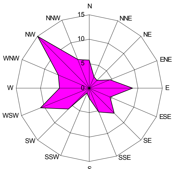
Rosa dei Venti della Stazione Melilli - Anno 2005
