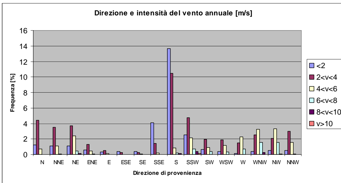
Figura 4: Distribuzione annuale di frequenza delle classi di intensità e direzione del vento (Porto Torres - anno 1998)
