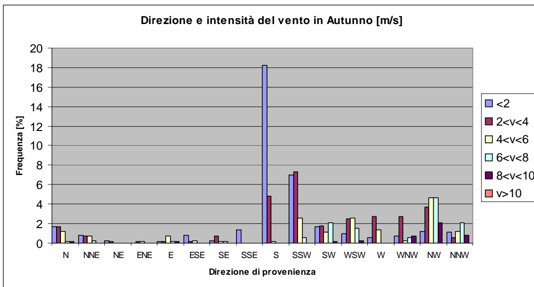
Figura 10: Distribuzione in autunno di frequenza delle classi di intensità e direzione del vento (Porto Torres - anno 1998)
