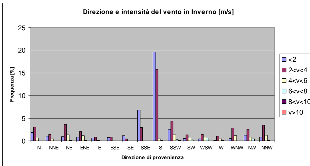
Figura 12: Distribuzione in inverno di frequenza delle classi di intensità e direzione del vento (Porto Torres - anno 1998)
