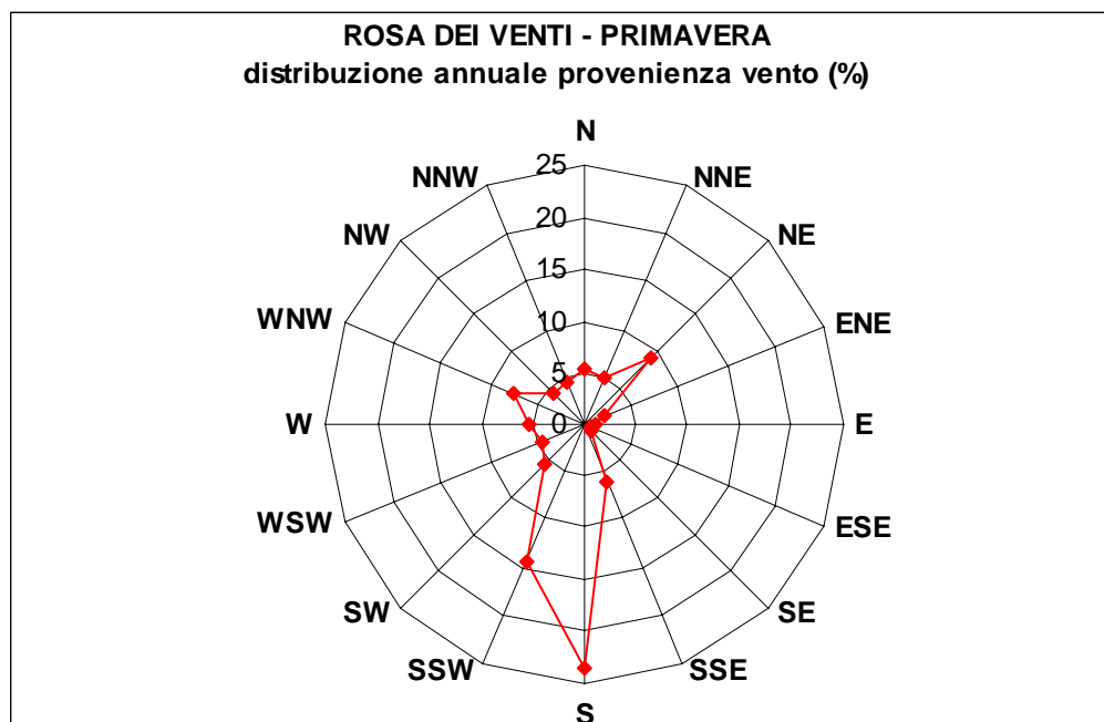
Figura 5: Rosa venti in primavera (Porto Torres - anno 1998)
