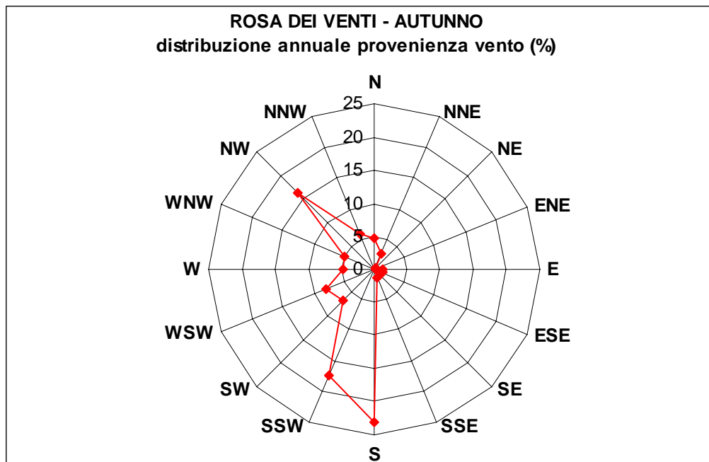
Figura 9: Rosa venti in autunno (Porto Torres - anno 1998)
