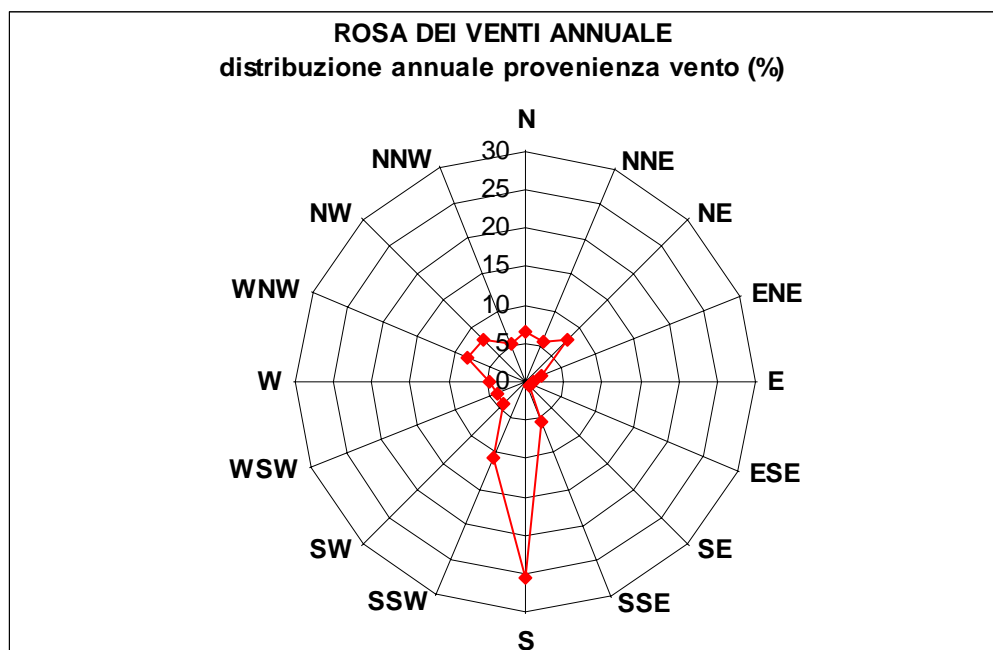
Figura 3: Rosa venti annuale (Porto Torres - anno 1998)
