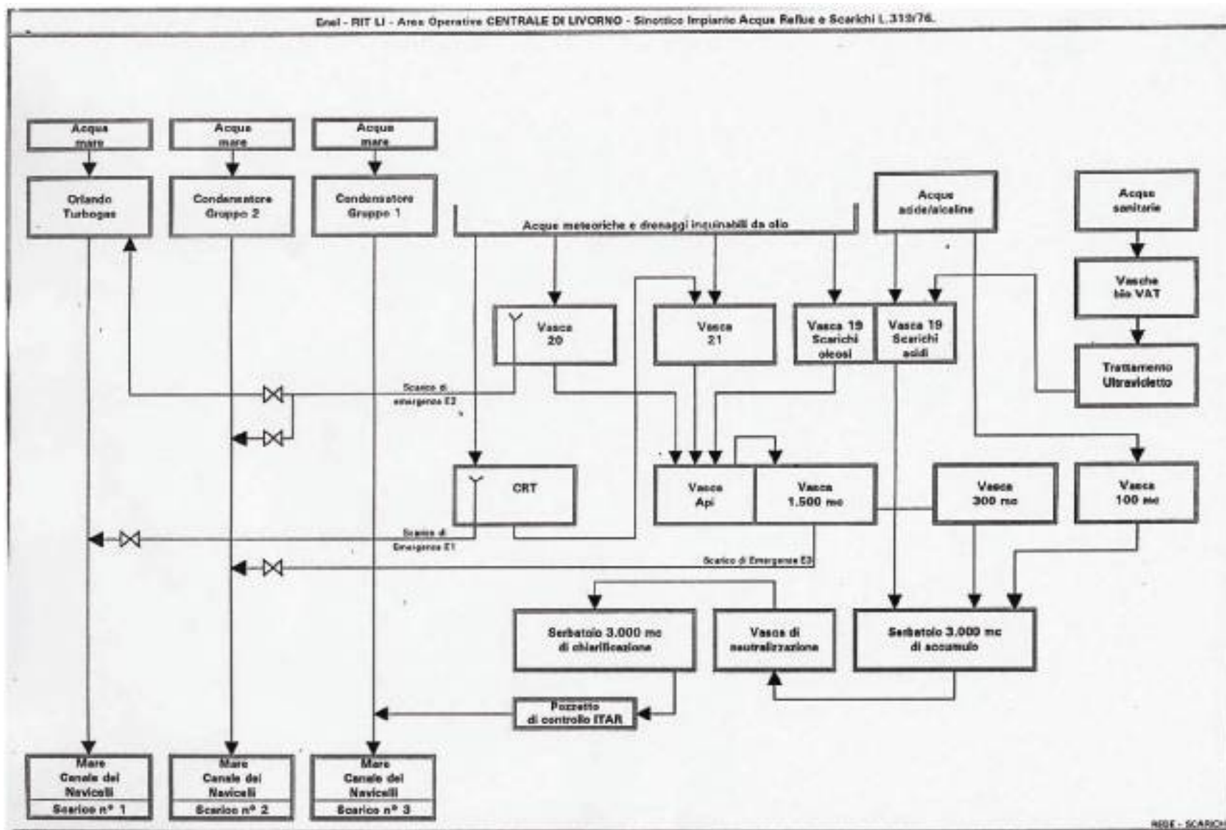
B.18 – Figura 1 - schema di flusso impianto trattamento acque reflue
