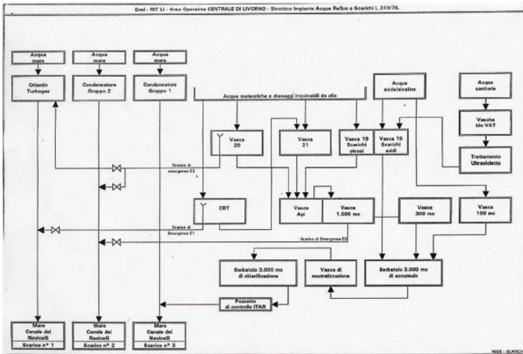
B.21 – schema di flusso impianto trattamento acque reflue
