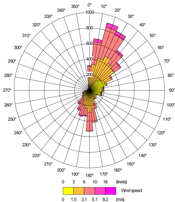
Figura 4-3: rosa dei venti per l'anno 2005
