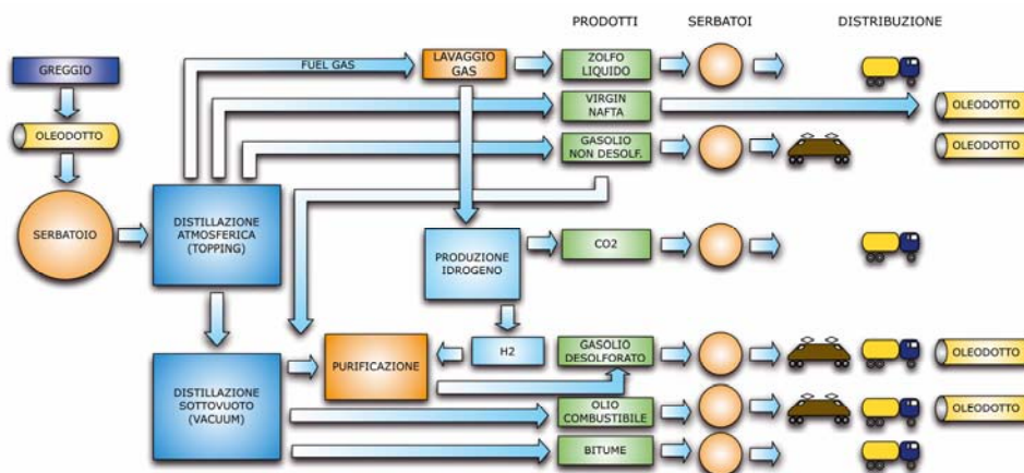
Figura 5 – Schema di flusso del ciclo di lavorazione
