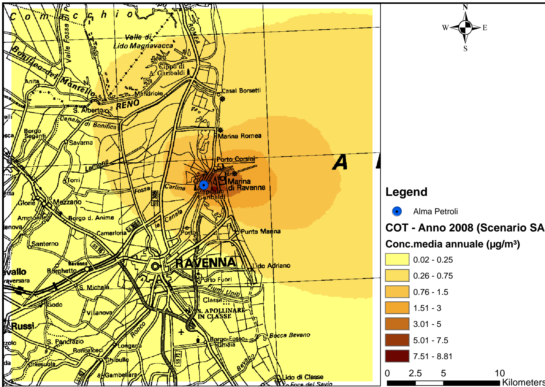
Mappa 5- Concentrazione massima su media annua – CALPUFF – COT- SCENARIO AUTORIZZATO – Anno 2008
