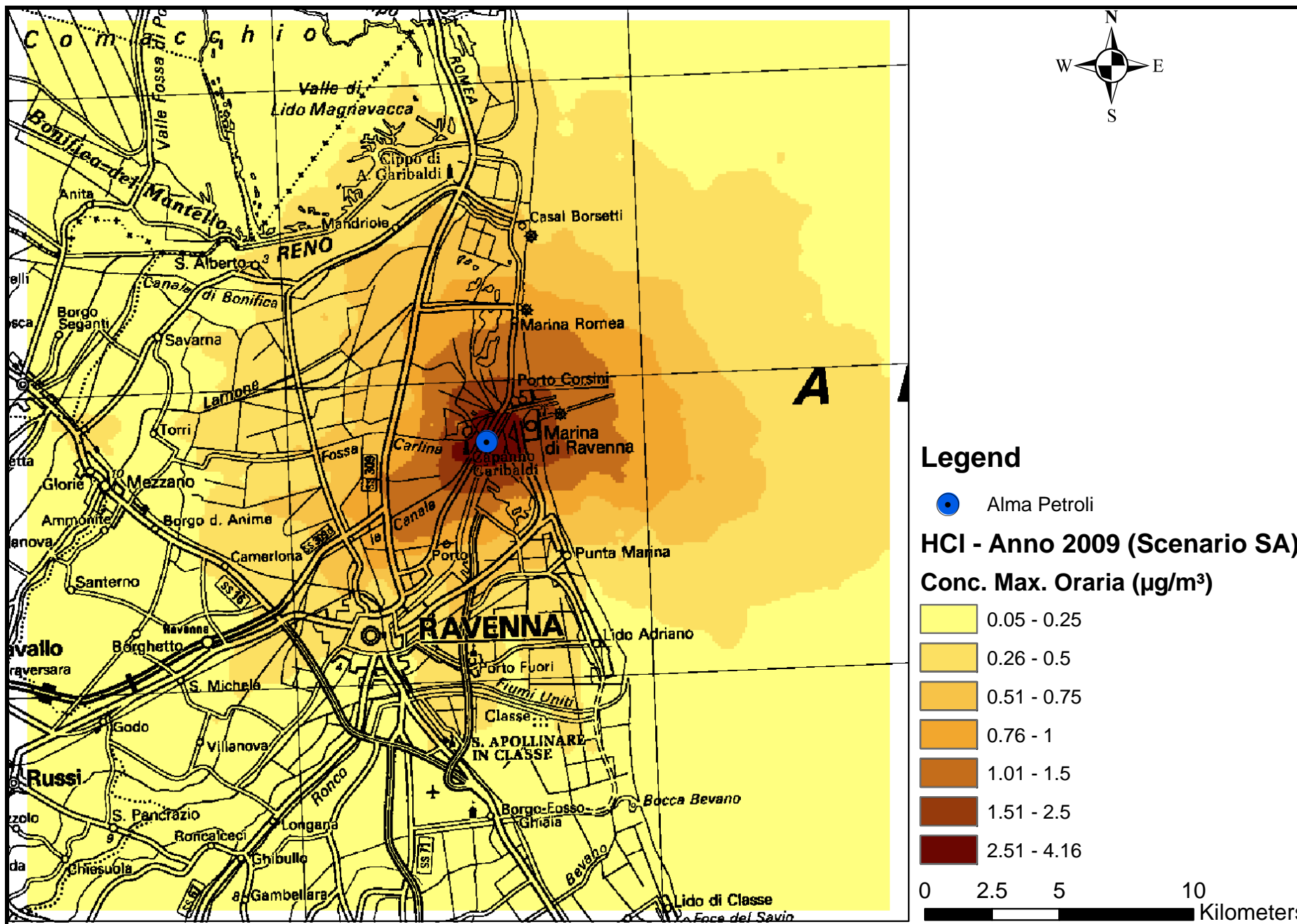
Mappa 8- Concentrazione massima su media oraria – CALPUFF – HCL- SCENARIO AUTORIZZATO – Anno 2009
