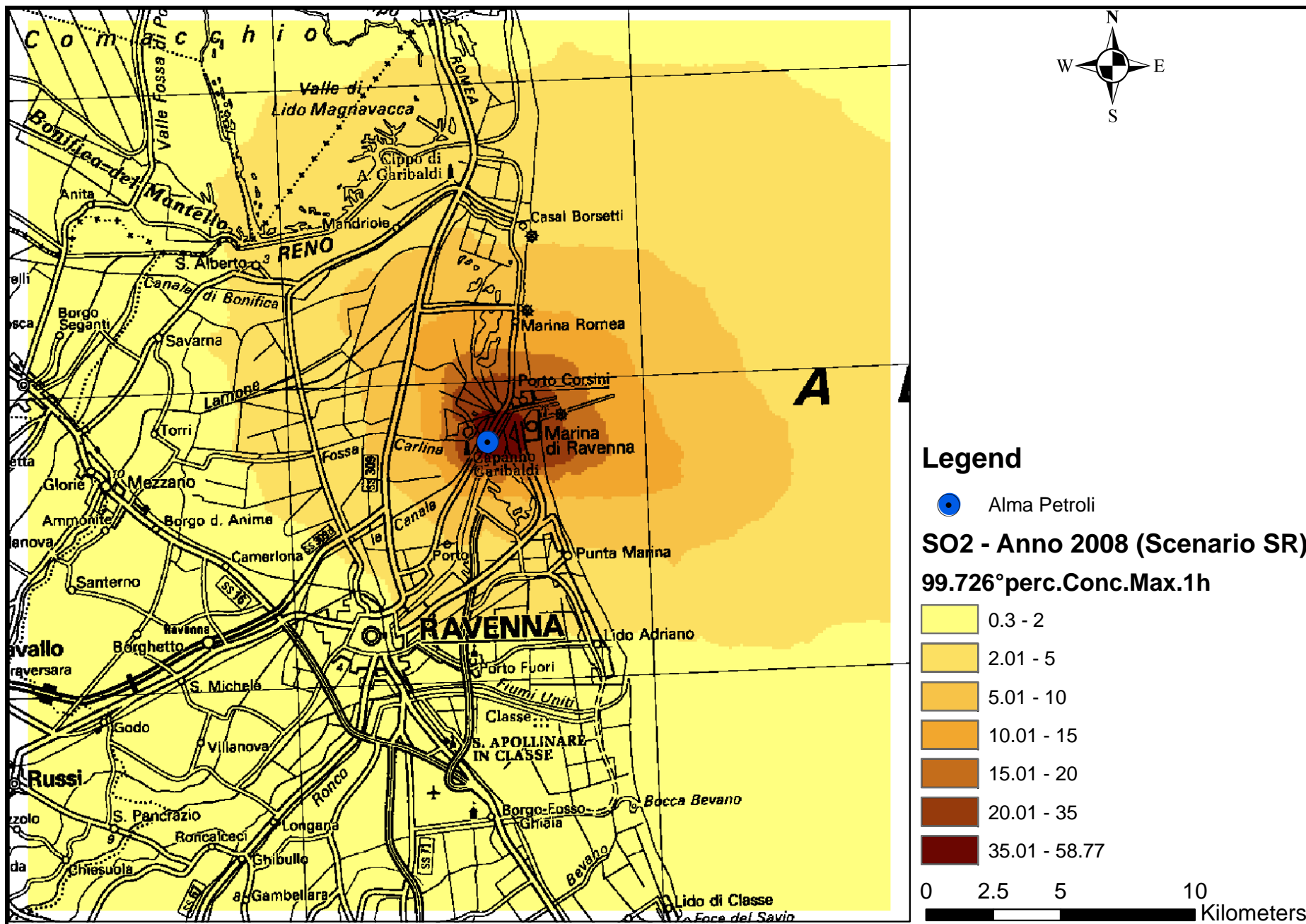
Mapa 43 - 99,726° percentile Concentrazione massima su media oraria – CALPUFF – SO x - SCENARIO REALE – Anno 2008
