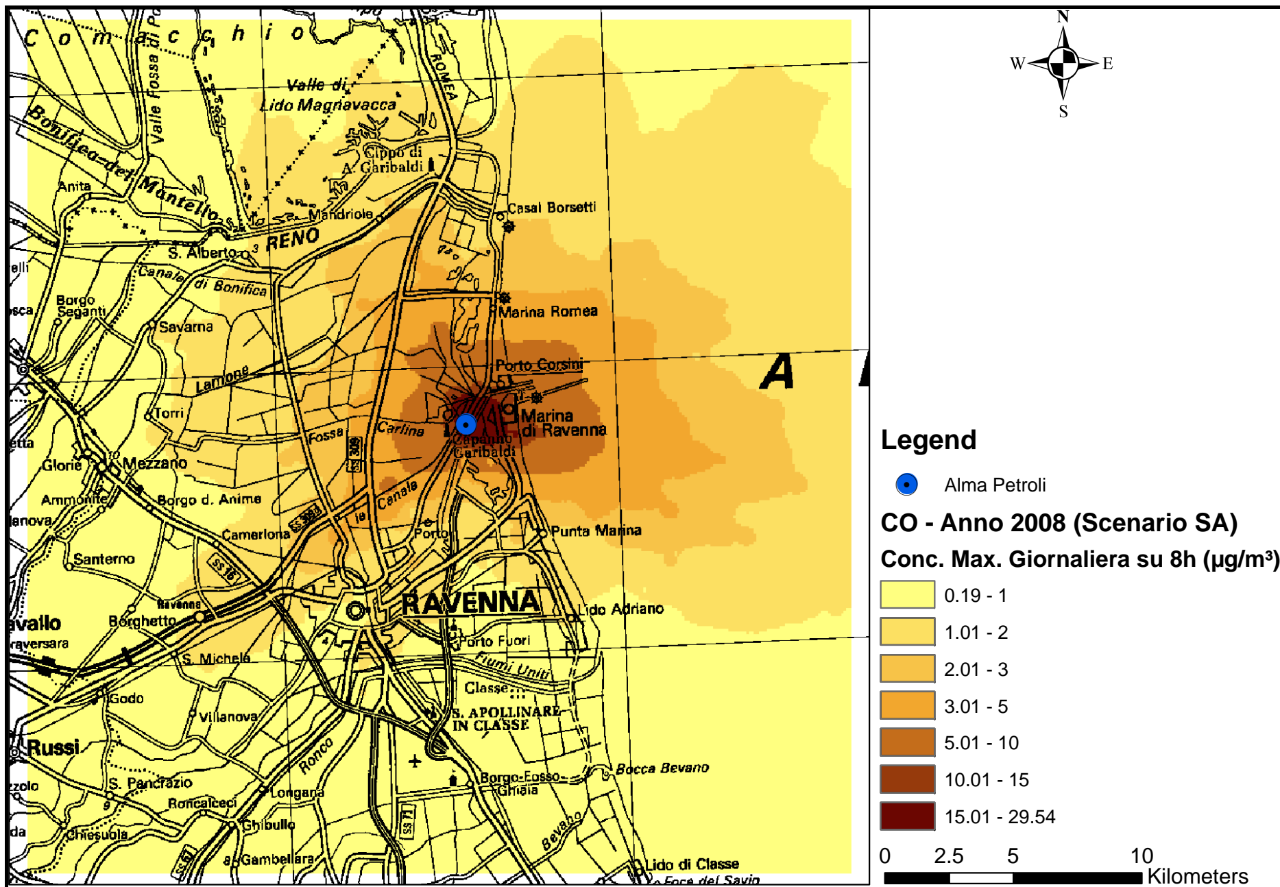
Mappa 1- Concentrazione massima giornaliera su media di 8 ore – CALPUFF – CO- SCENARIO AUTORIZZATO – Anno 2008
