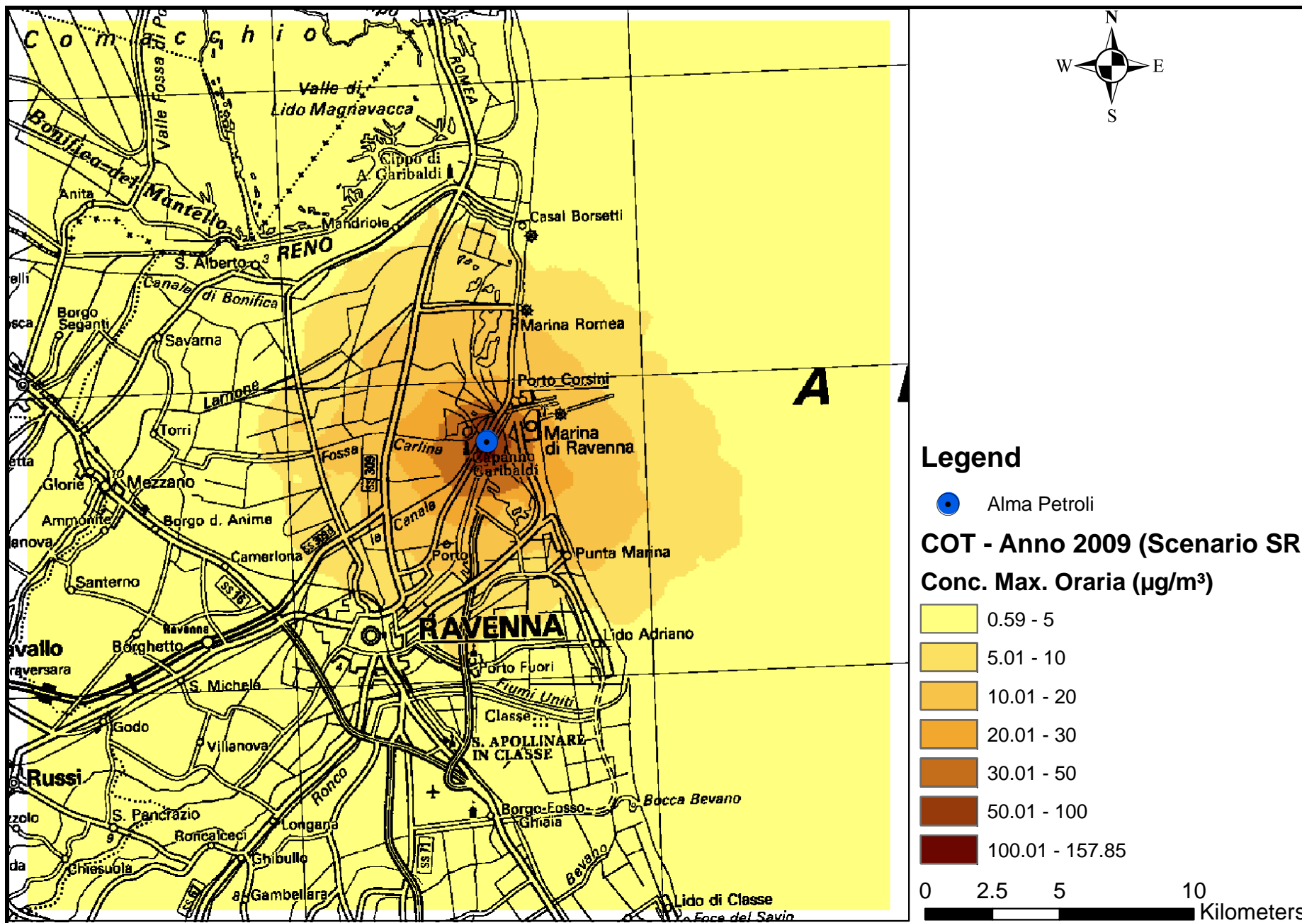
Mappa 28 - Concentrazione massima su media oraria – CALPUFF – COT- SCENARIO REALE – Anno 2009
