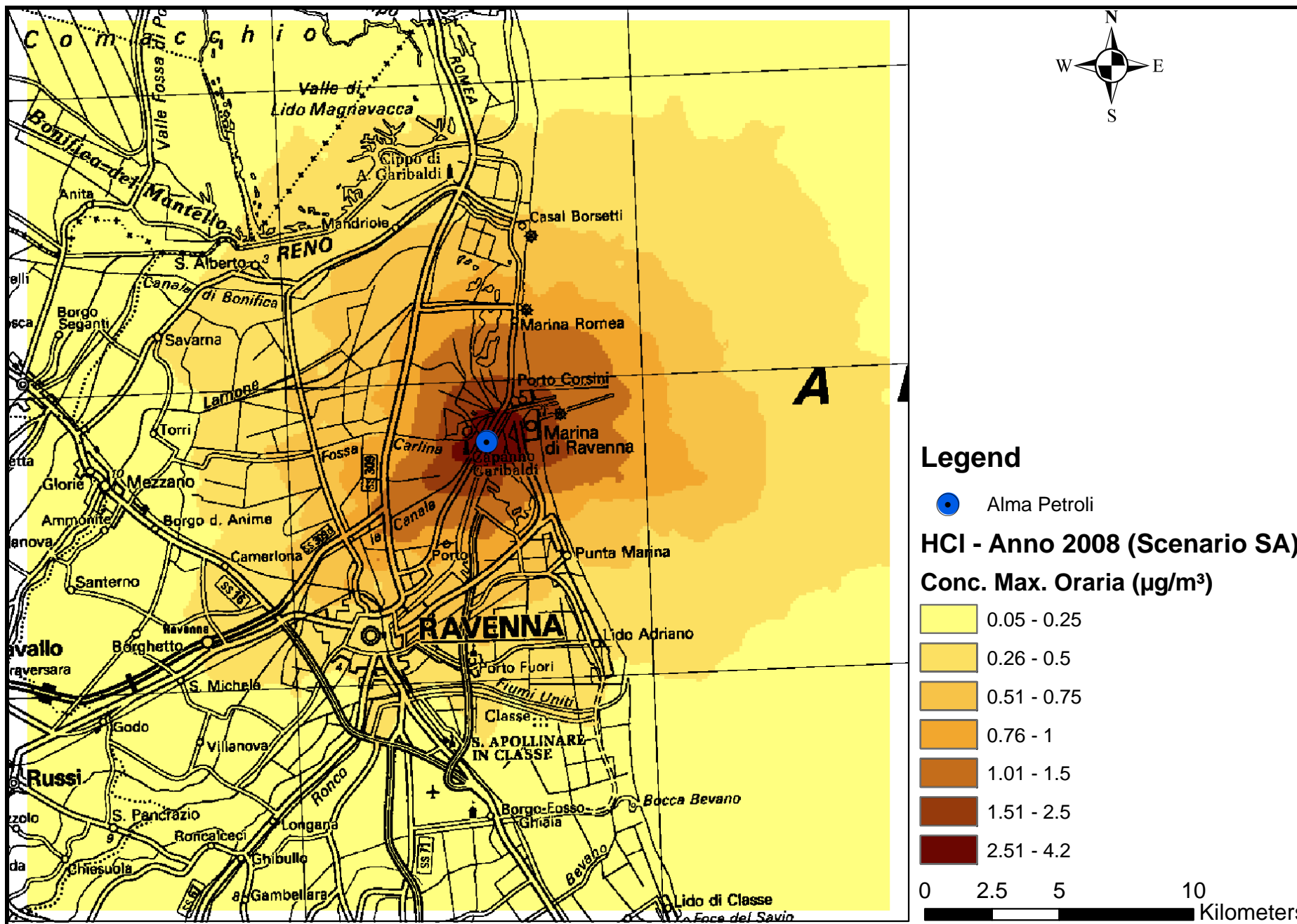
Mapa 7- Concentrazione massima su media oraria – CALPUFF – HCL- SCENARIO AUTORIZZATO – Anno 2008
