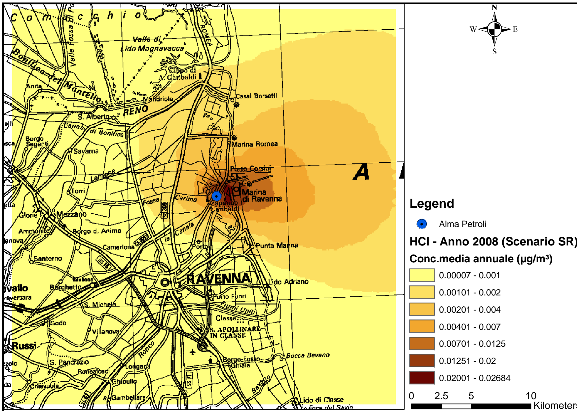
Mapa 33 - Concentrazione massima su media annua – CALPUFF – HCL- SCENARIO REALE – Anno 2008
