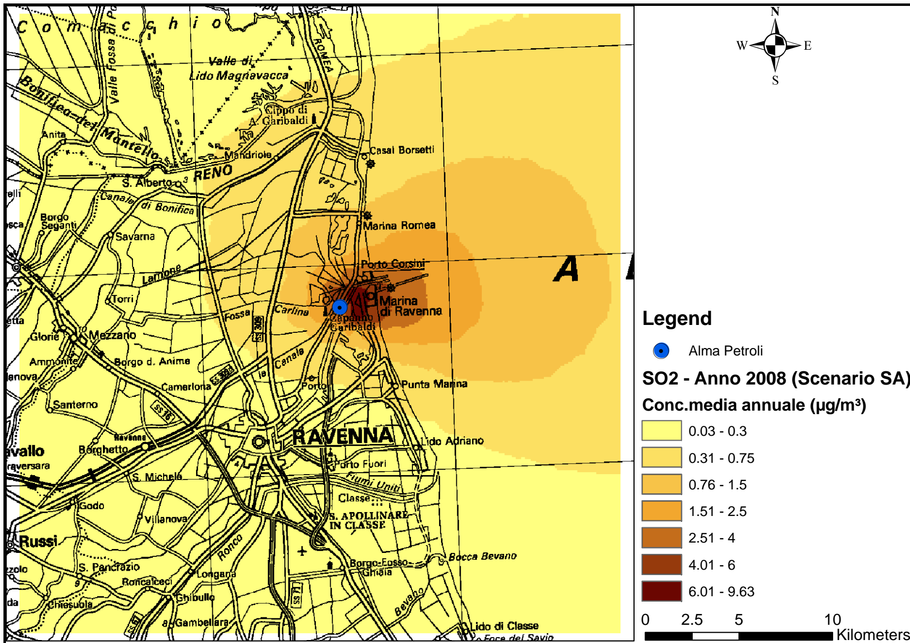
Mappa 23 - Concentrazione massima su media annua – CALPUFF – SO x - SCENARIO AUTORIZZATO – Anno 2008
