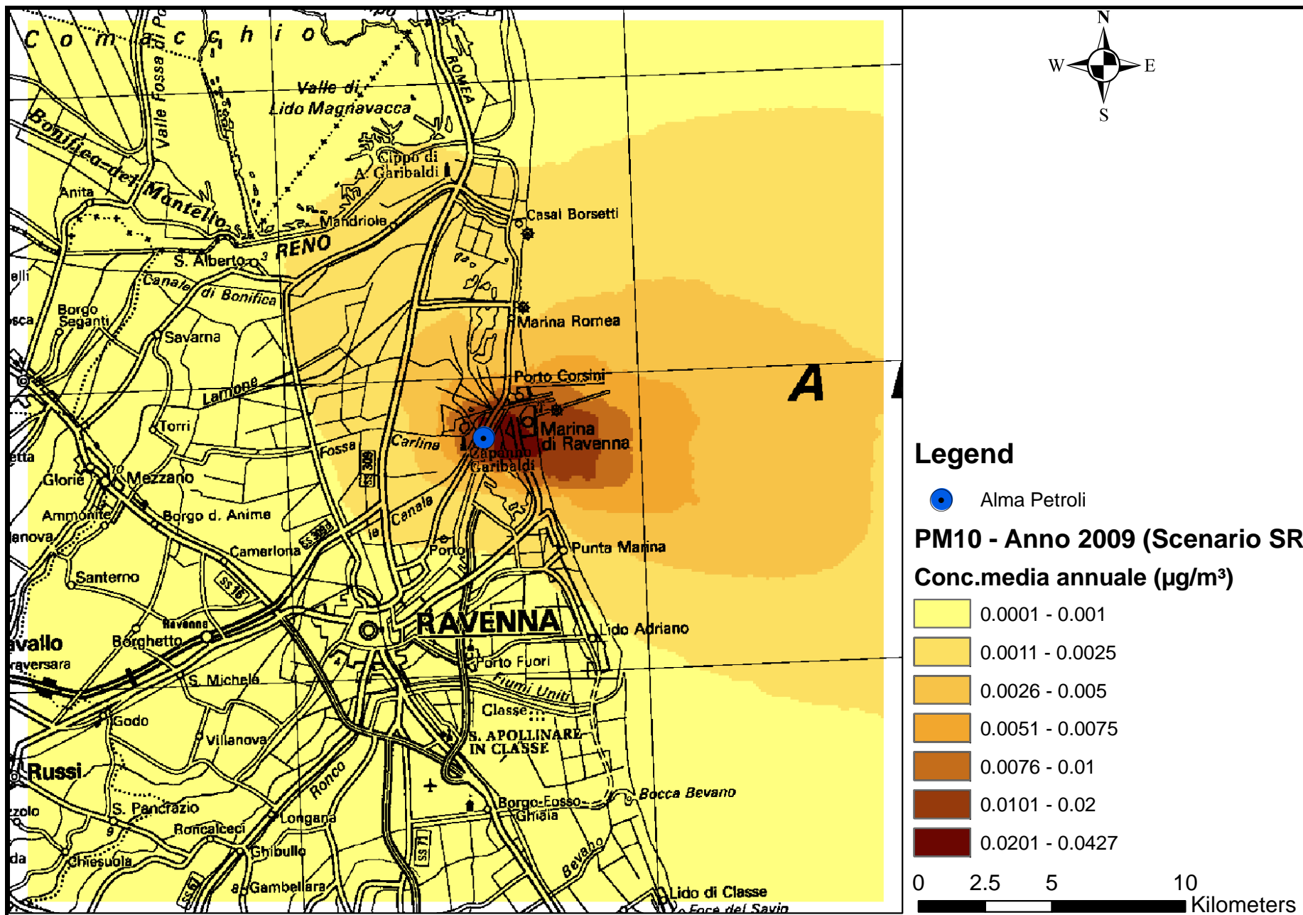
Mappa 42 - Concentrazione massima su media annua – CALPUFF – PM10- SCENARIO REALE – Anno 2009
