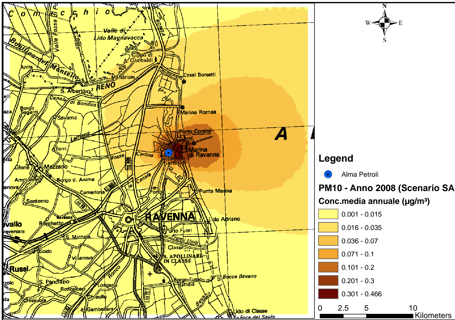
Mapa 17 - Concentrazione massima su media - annua - CALPUFF - PM10- SCENARIO AUTORIZZATO - Anno 2008
