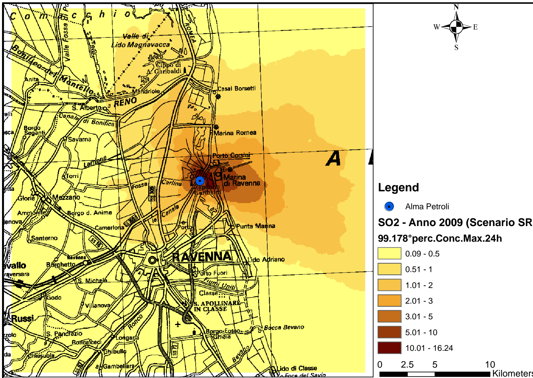
Mappa 46 - 99.178° Concentrazione massima su media giornaliera – CALPUFF – SO x - SCENARIO REALE – Anno 2009
