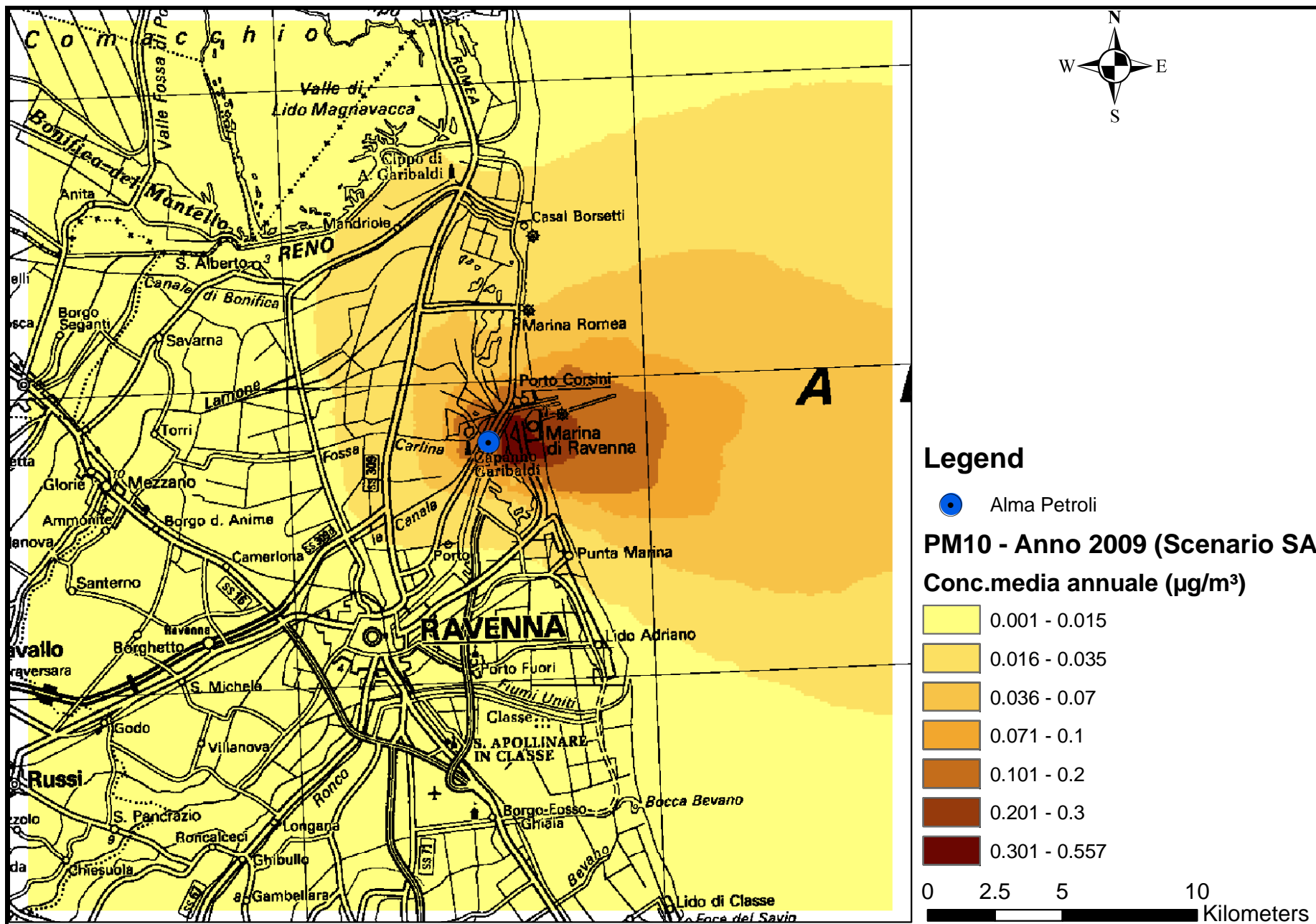
Mappa 18 - Concentrazione massima su media - annua - CALPUFF - PM10- SCENARIO AUTORIZZATO - Anno 2009
