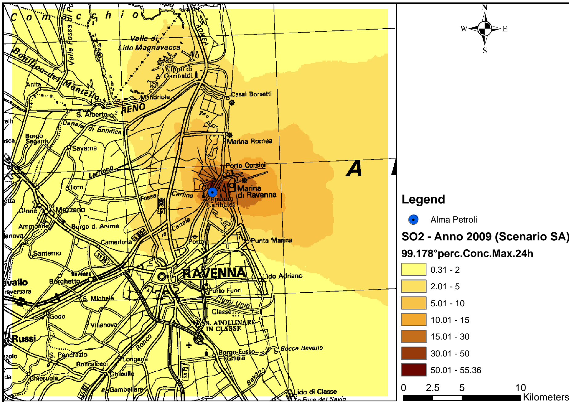
Mappa 22 - 99.178° Concentrazione massima su media giornaliera – CALPUFF – SO x - SCENARIO AUTORIZZATO – Anno 2009
