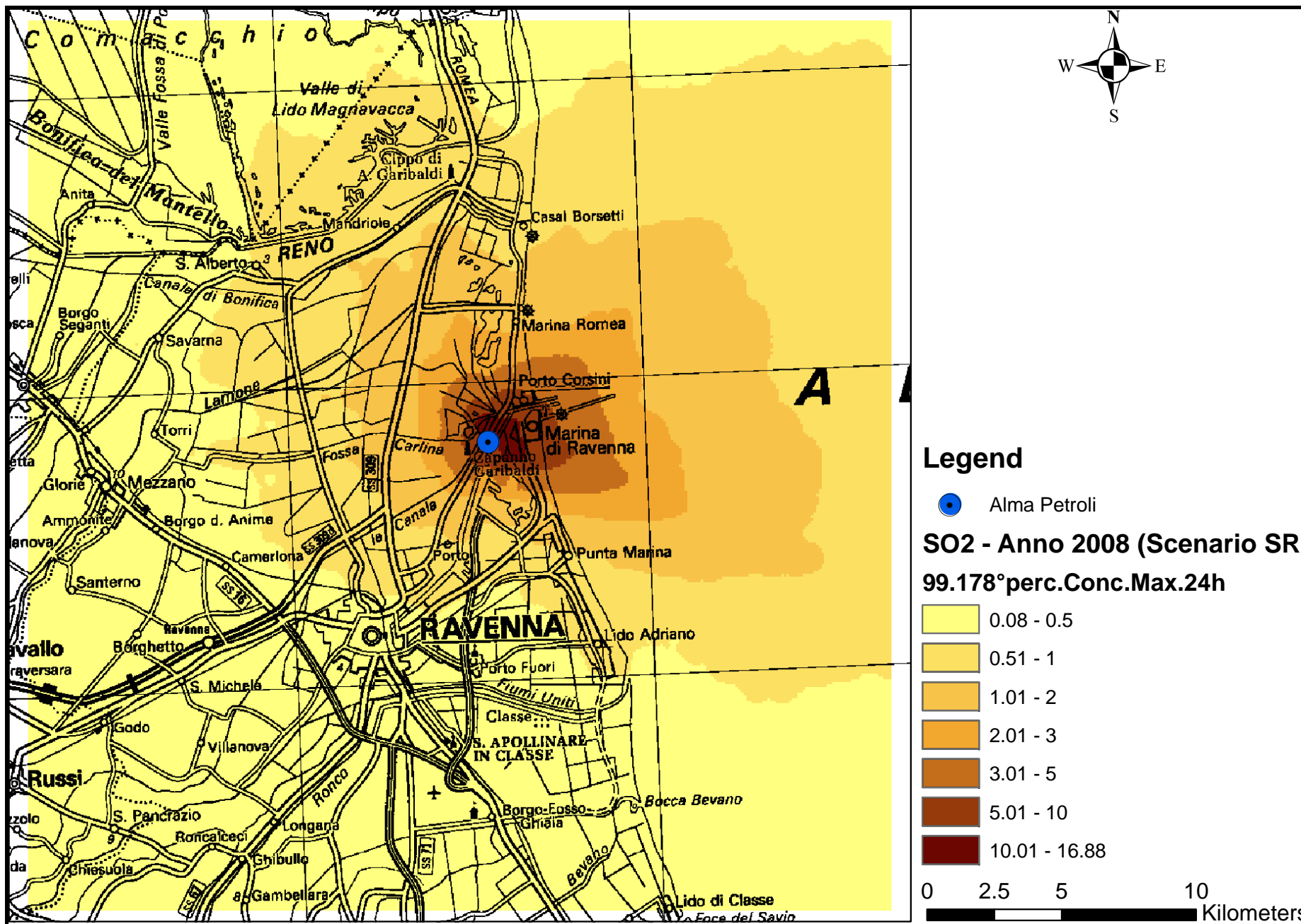
Mappa 45 - 99.178° Concentrazione massima su media giornaliera – CALPUFF – SO x - SCENARIO REALE – Anno 2008
