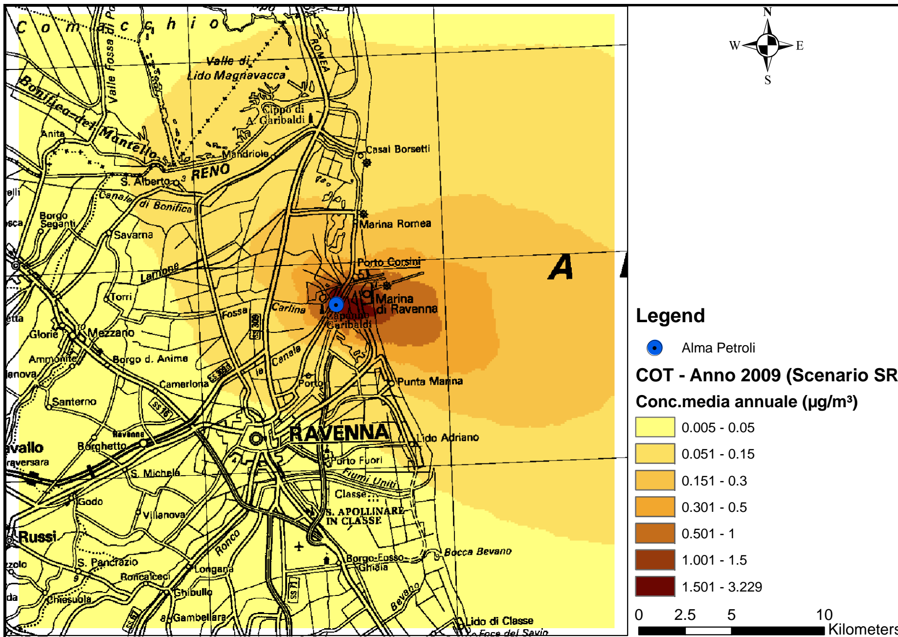
Mappa 30 - Concentrazione massima su media annua – CALPUFF – COT- SCENARIO REALE – Anno 2009
