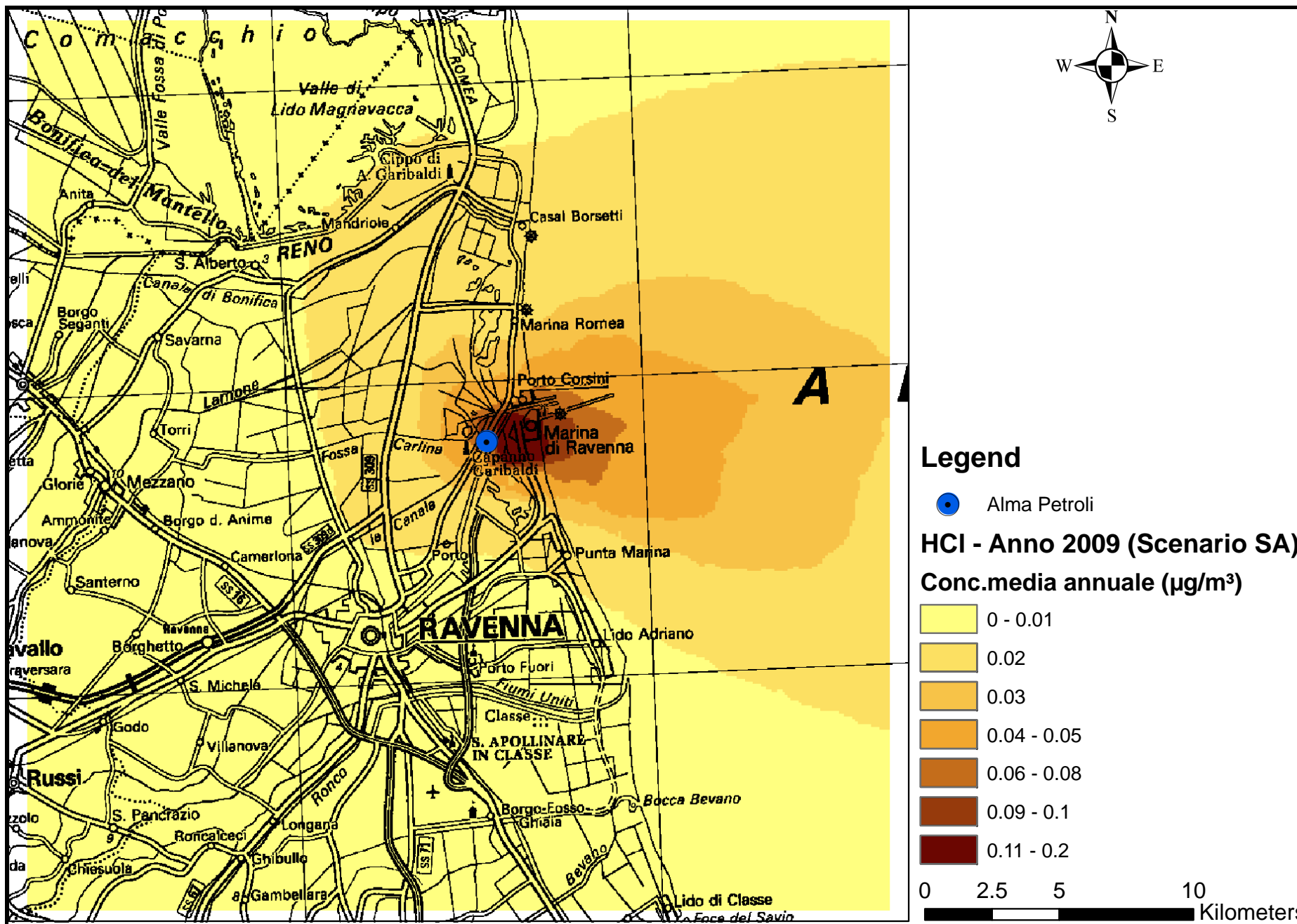
Mappa 10 - Concentrazione massima su media annua – CALPUFF – HCL- SCENARIO AUTORIZZATO – Anno 2009
