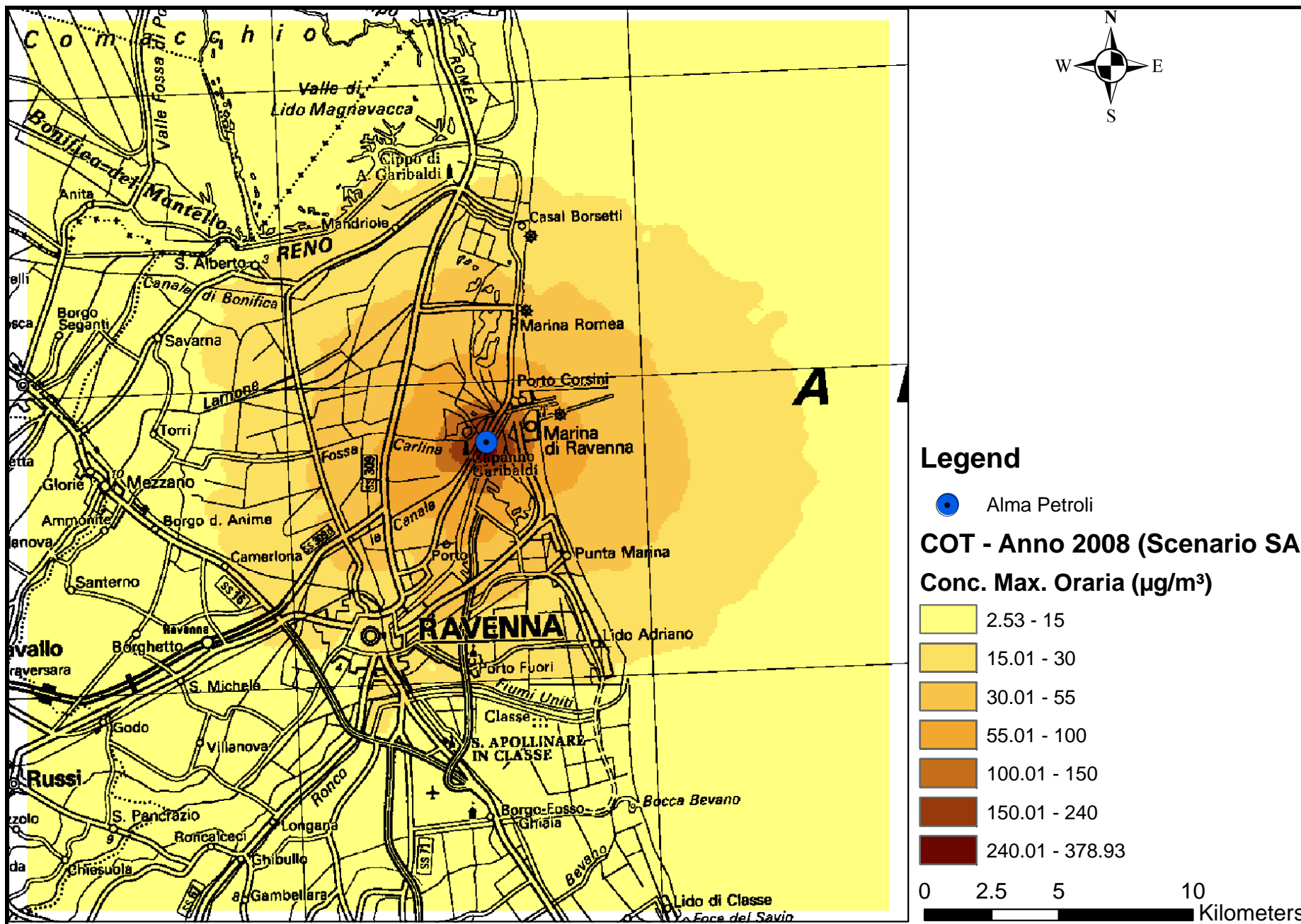
Mapa 3- Concentrazione massima su media oraria – CALPUFF – COT- SCENARIO AUTORIZZATO – Anno 2008
