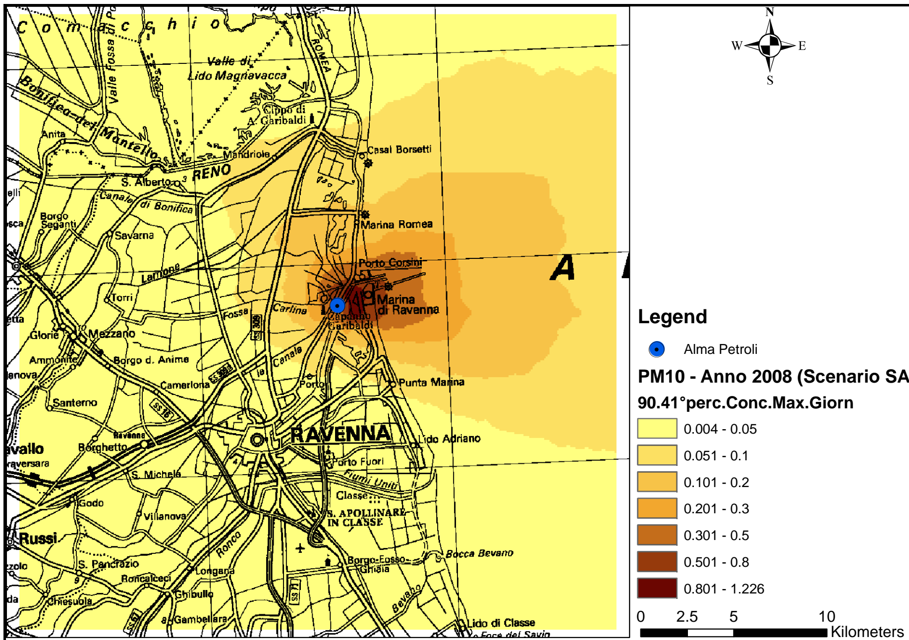
Mappa 15 - 90,41° percentile Concentrazione massima su media giornaliera – CALPUFF – PM10- SCENARIO AUTORIZZATO – Anno 2008
