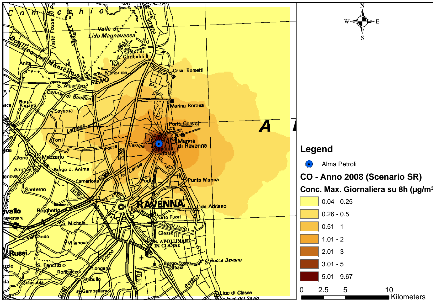
Mappa 25 - Concentrazione massima giornaliera su media di 8 ore – CALPUFF – CO - SCENARIO REALE – Anno 2008
