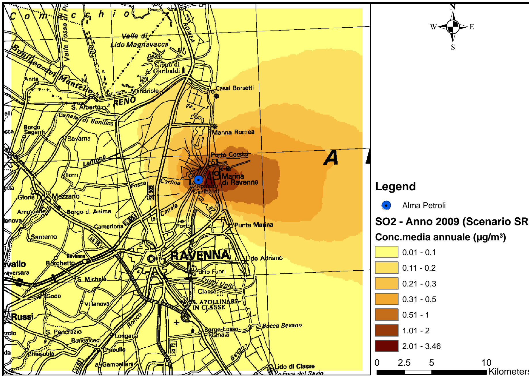
Mappa 48 - Concentrazione massima su media annua – CALPUFF – SO x - SCENARIO REALE – Anno 2009
