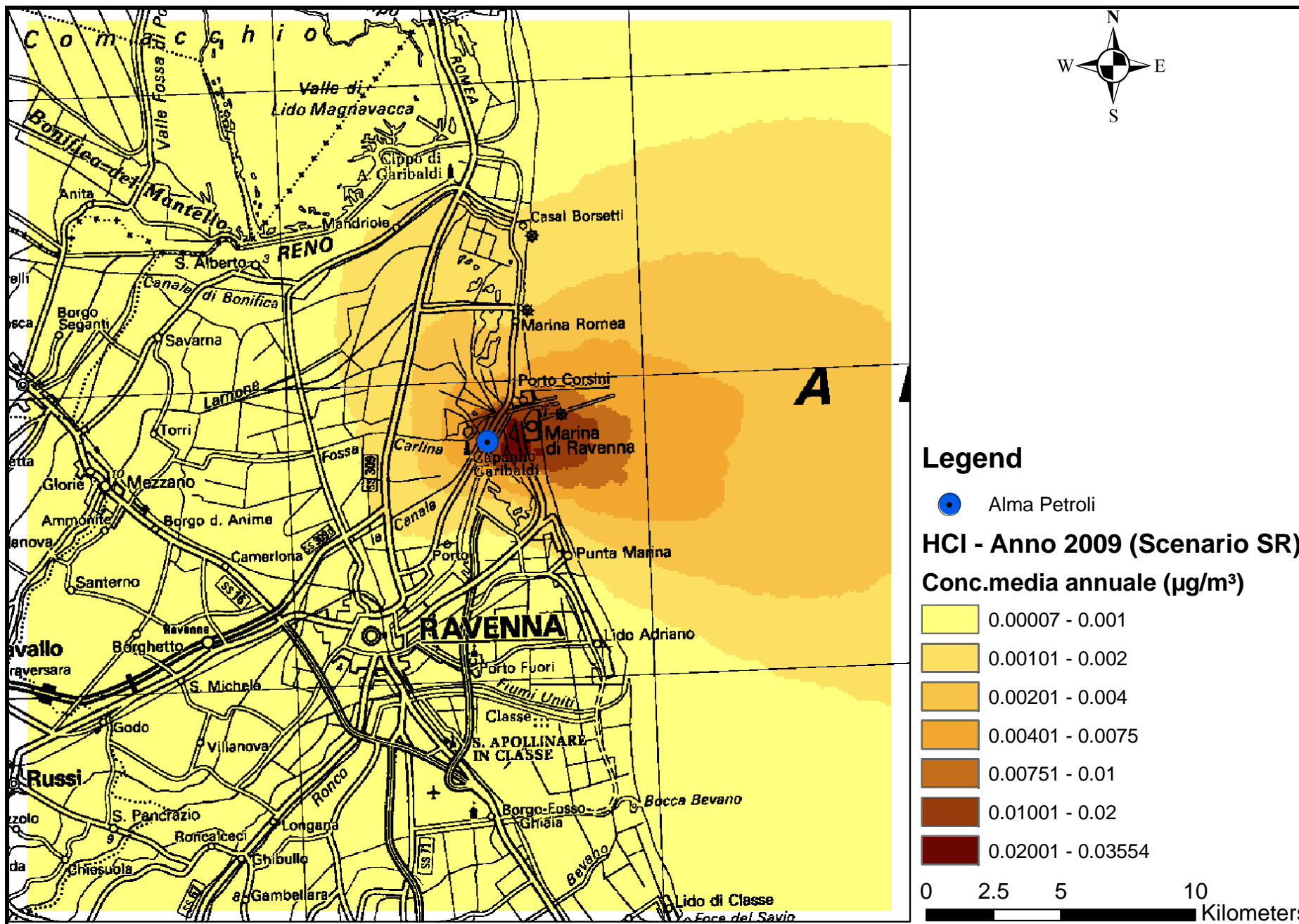
Mapa 34 - Concentrazione massima su media annua – CALPUFF – HCL- SCENARIO REALE – Anno 2009
