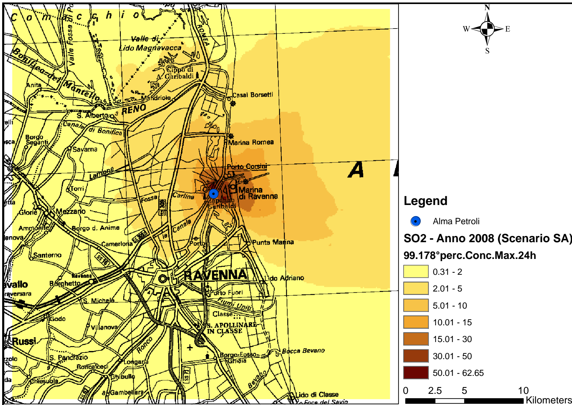
Mappa 21 - 99.178° Concentrazione massima su media giornaliera – CALPUFF – SO x - SCENARIO AUTORIZZATO – Anno 2008
