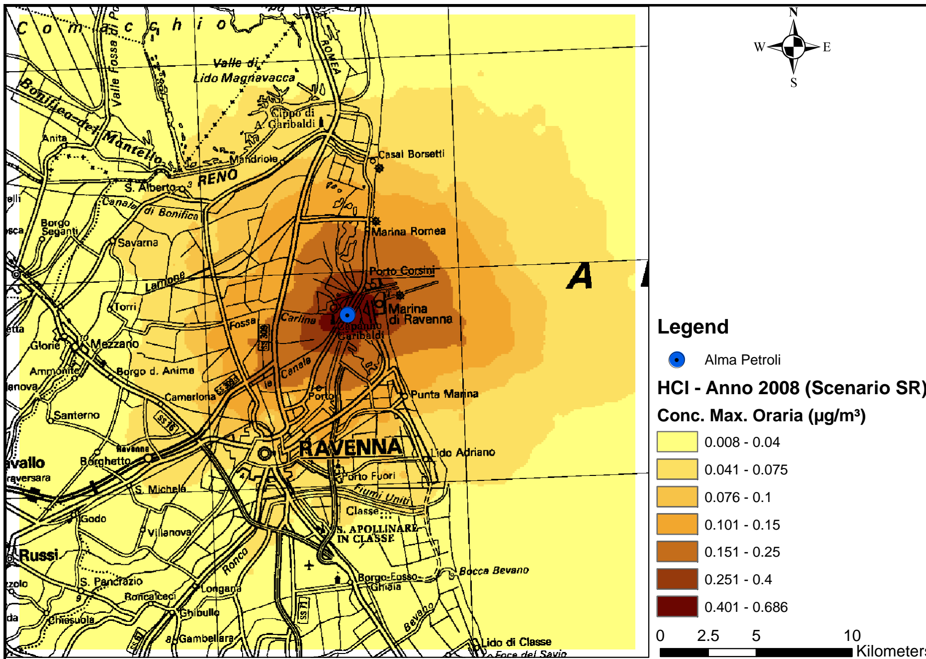
Mappa 31 - Concentrazione massima su media oraria – CALPUFF – HCL- SCENARIO REALE – Anno 2008
