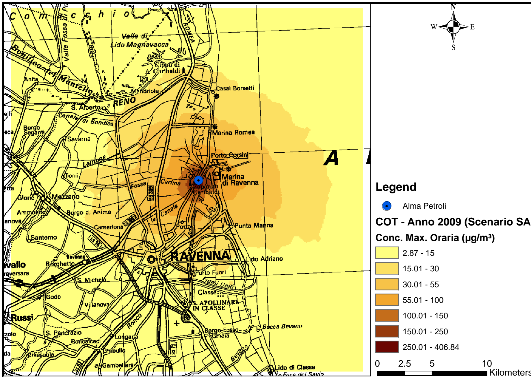
Mapa 4- Concentrazione massima su media oraria – CALPUFF – COT- SCENARIO AUTORIZZATO – Anno 2009
