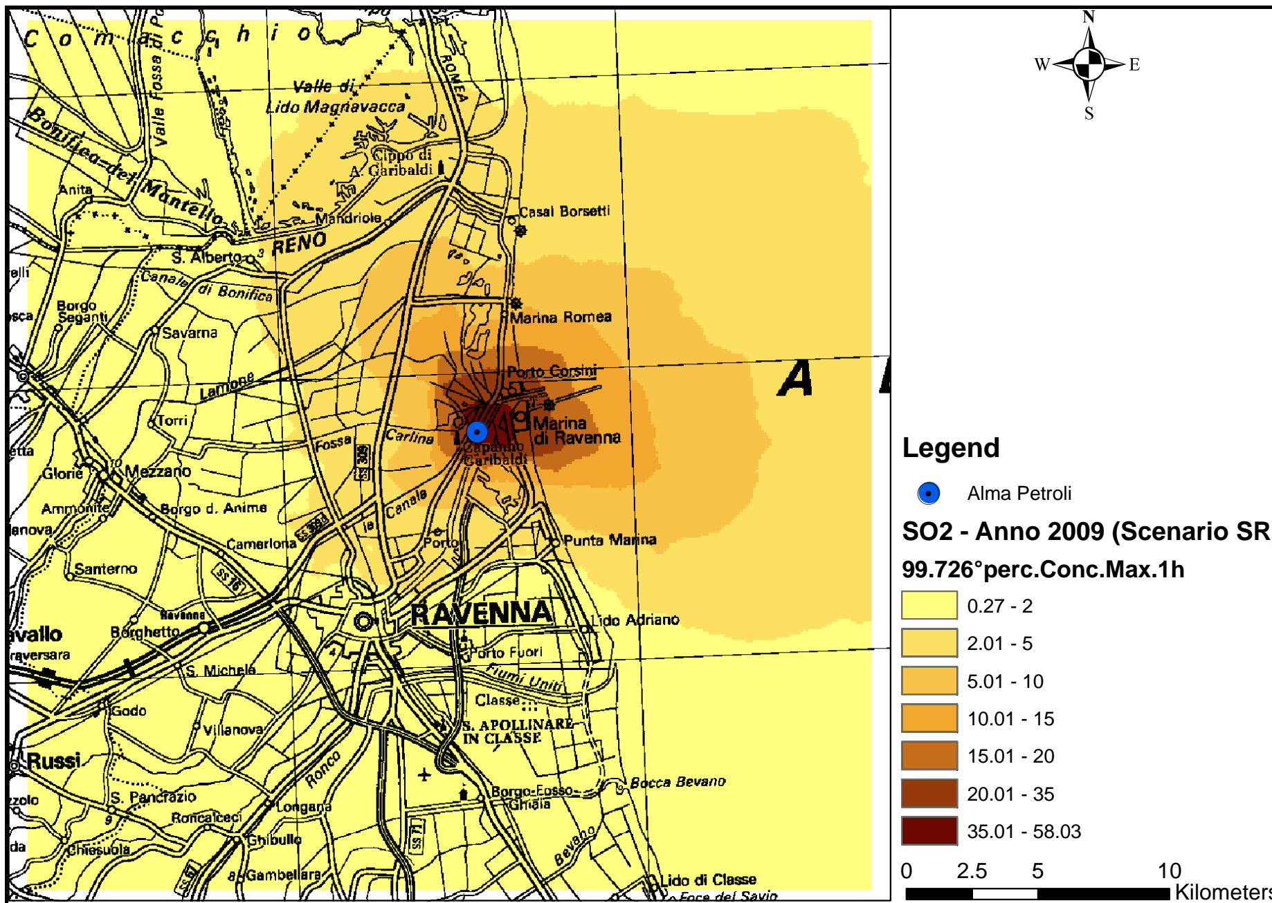
Mappa 44 - 99,726° percentile Concentrazione massima su media oraria – CALPUFF – SOx- SCENARIO REALE – Anno 2009
