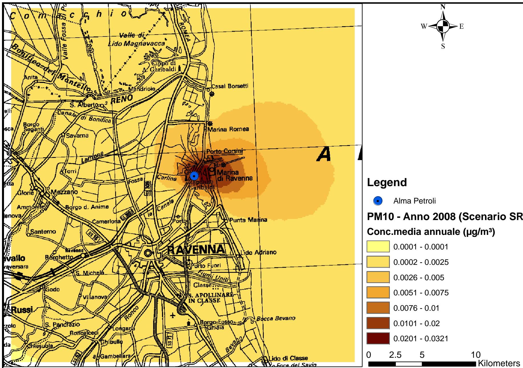
Mappa 41 - Concentrazione massima su media annua – CALPUFF – PM10- SCENARIO REALE – Anno 2008
