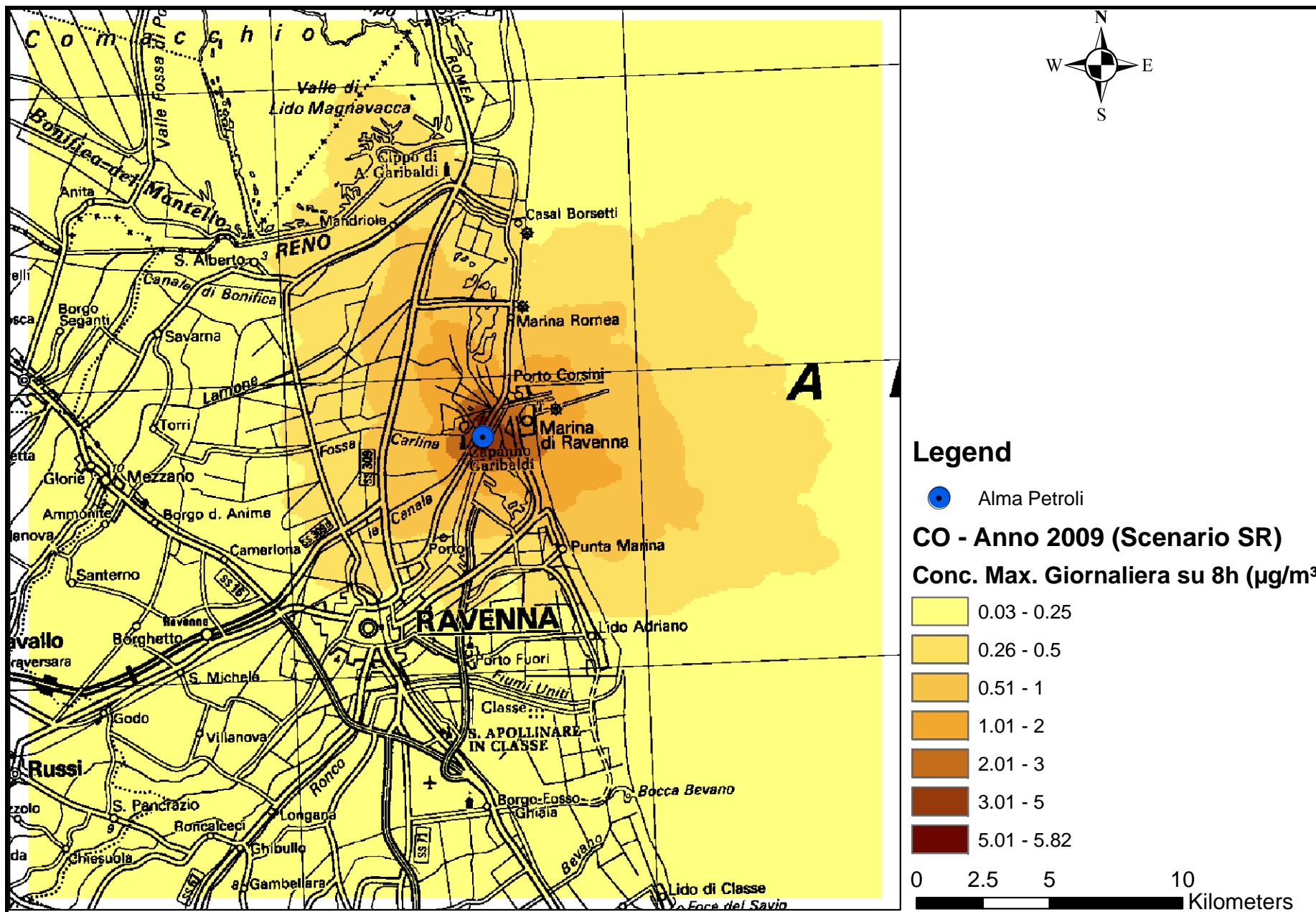
Mappa 26 - Concentrazione massima giornaliera su media di 8 ore – CALPUFF – CO - SCENARIO REALE – Anno 2009
