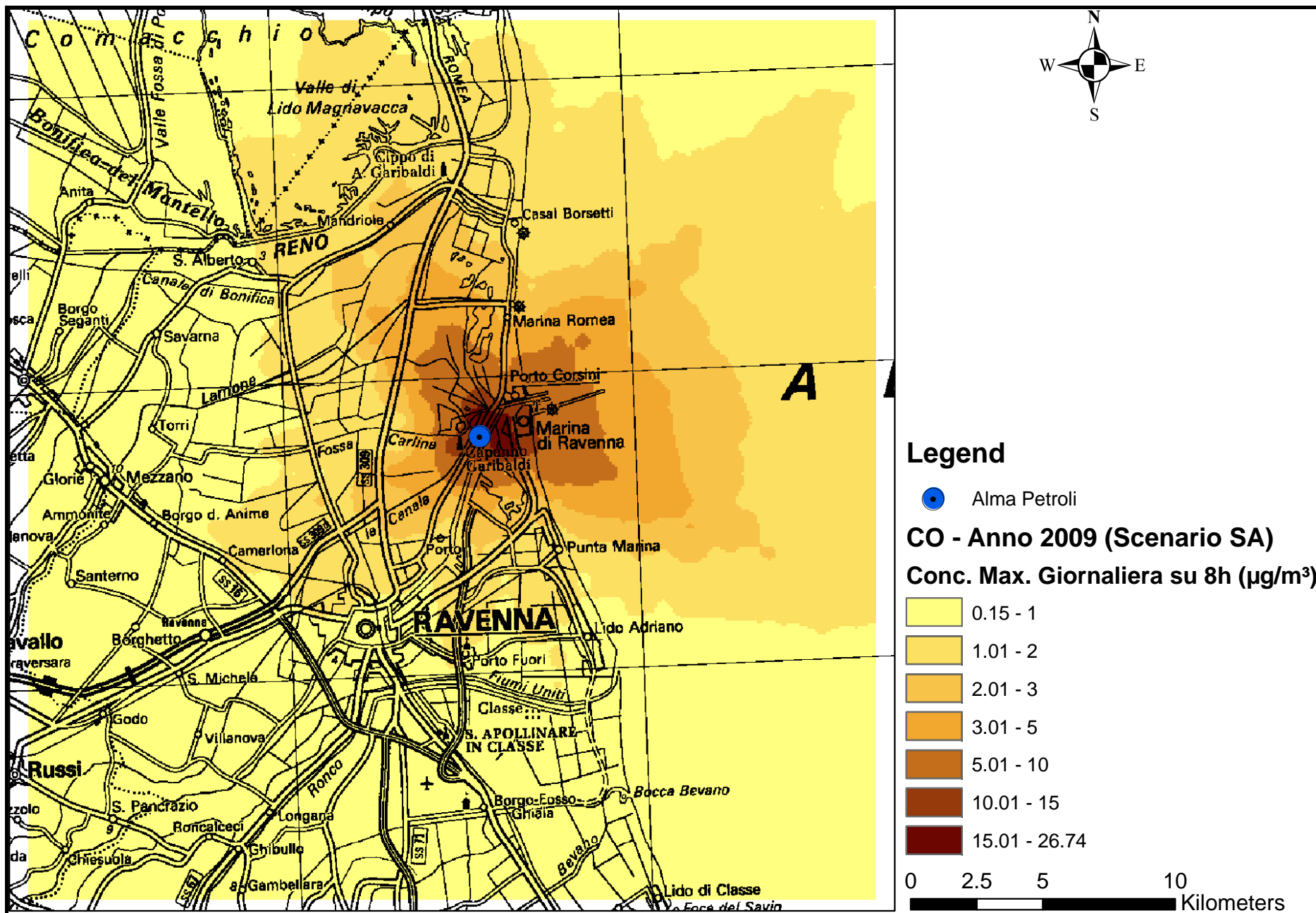
Mappa 2- Concentrazione massima giornaliera su media di 8 ore – CALPUFF – CO- SCENARIO AUTORIZZATO – Anno 2009
