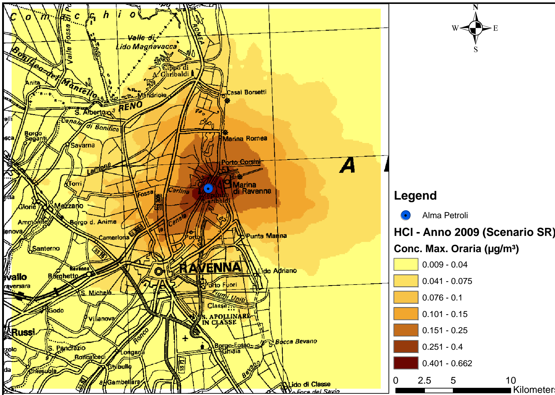
Mappa 32 - Concentrazione massima su media oraria – CALPUFF – HCL- SCENARIO REALE – Anno 2009
