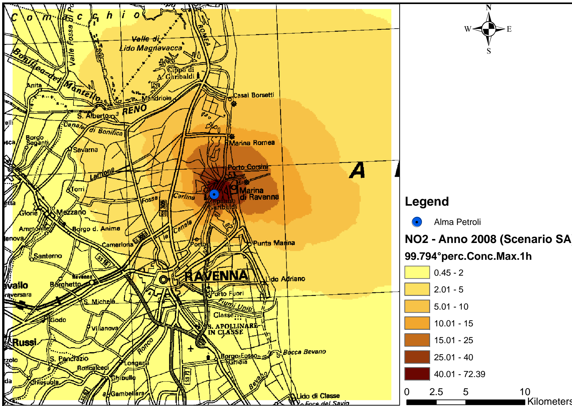
Mappa 11 - 99,794° percentile Concentrazione massima su media oraria – CALPUFF – NOx- SCENARIO AUTORIZZATO – Anno 2008
