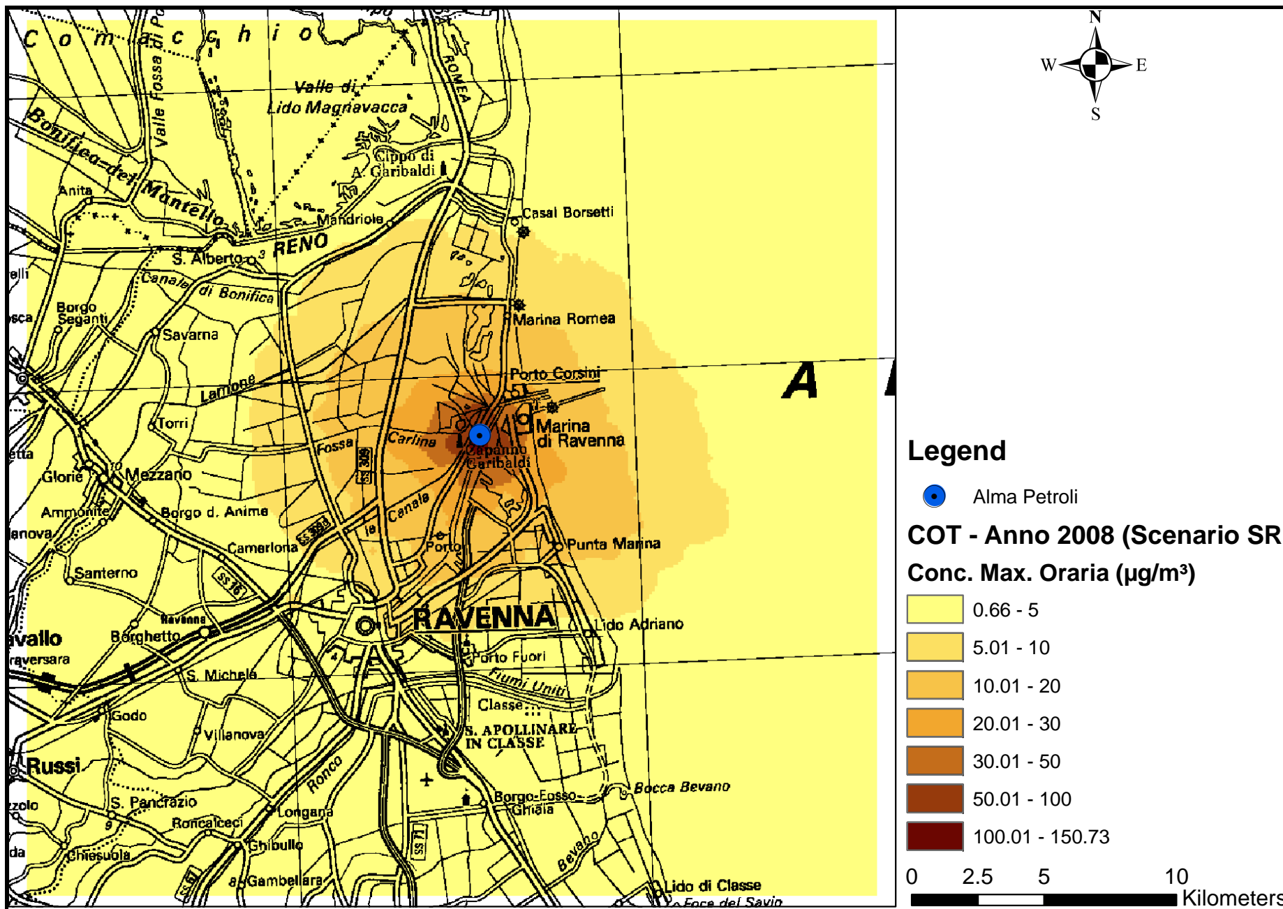
Mappa 27 - Concentrazione massima su media oraria – CALPUFF – COT- SCENARIO REALE – Anno 2008
