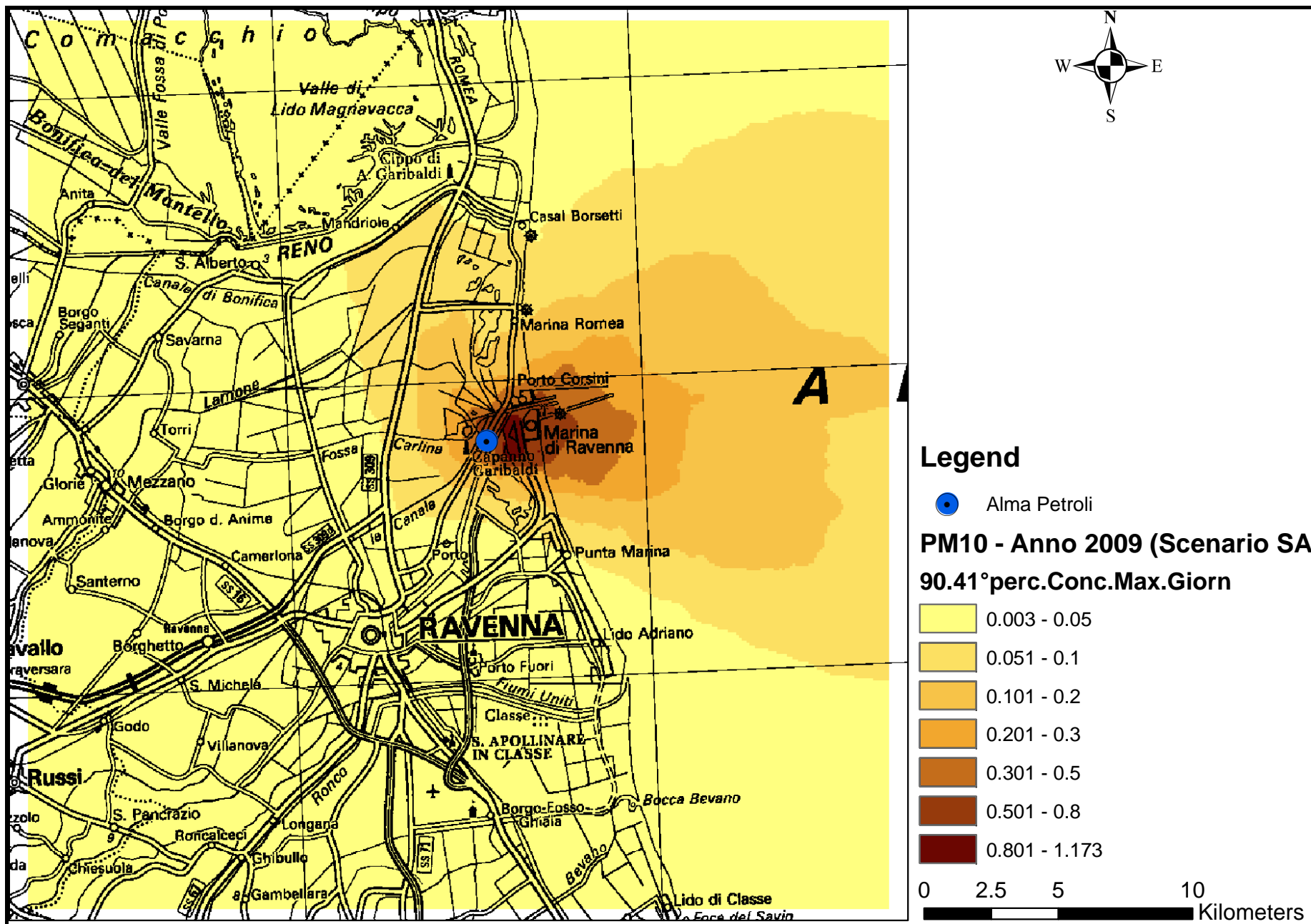
Mappa 16 - 90,41° percentile Concentrazione massima su media giornaliera – CALPUFF – PM10- SCENARIO AUTORIZZATO – Anno 2009
