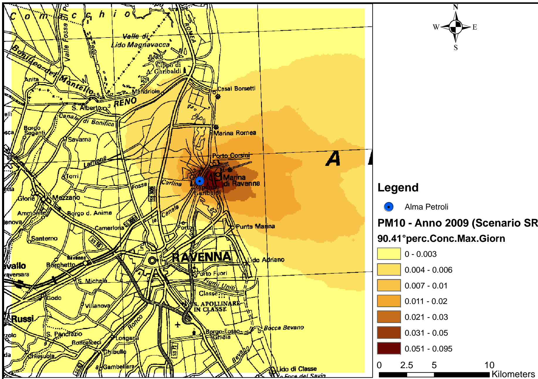
Mappa 40 - 90,41° percentile Concentrazione massima su media giornaliera – CALPUFF – PM10- SCENARIO REALE – Anno 2009
