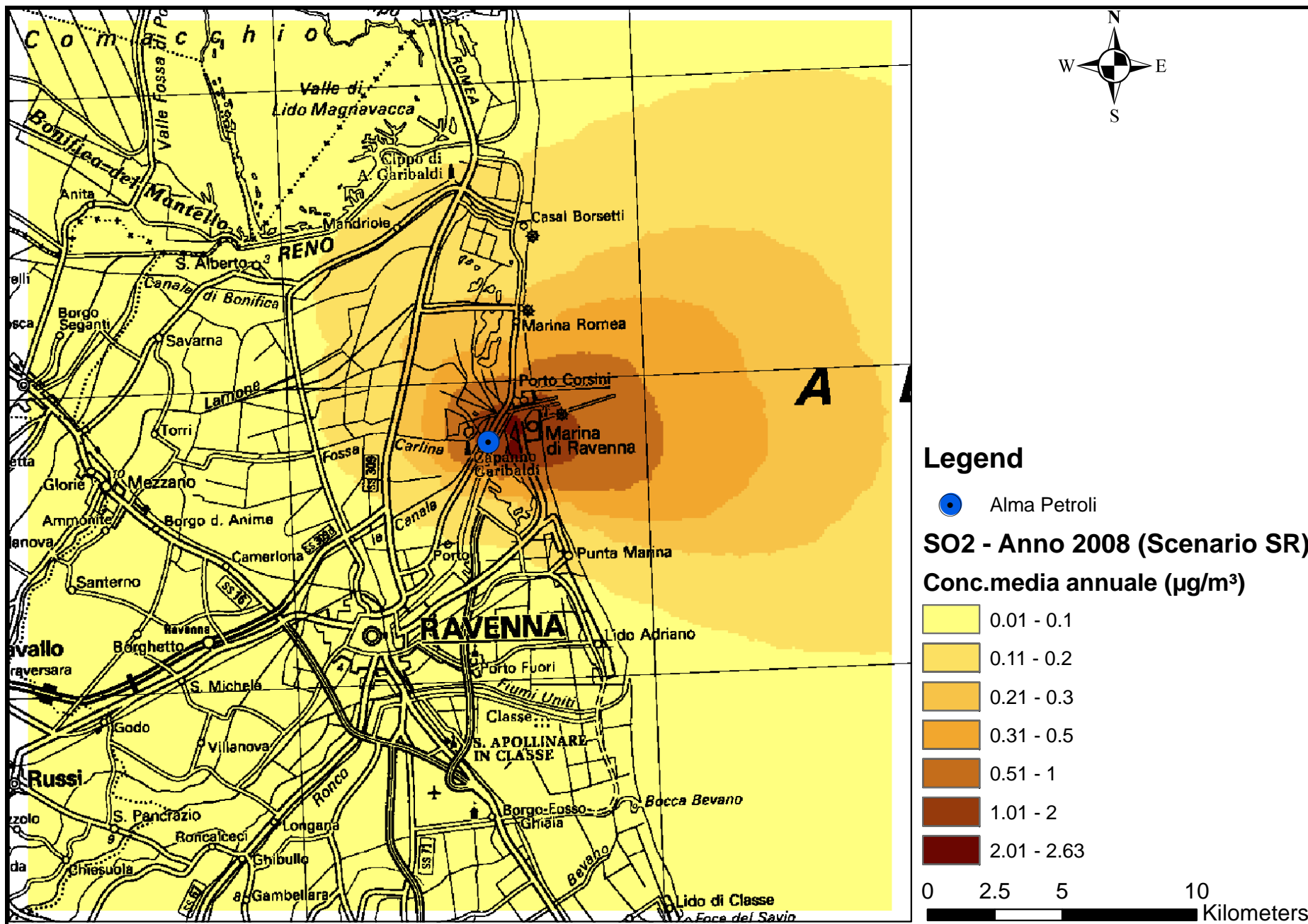
Mappa 47 - Concentrazione massima su media annua – CALPUFF – SO x - SCENARIO REALE – Anno 2008
