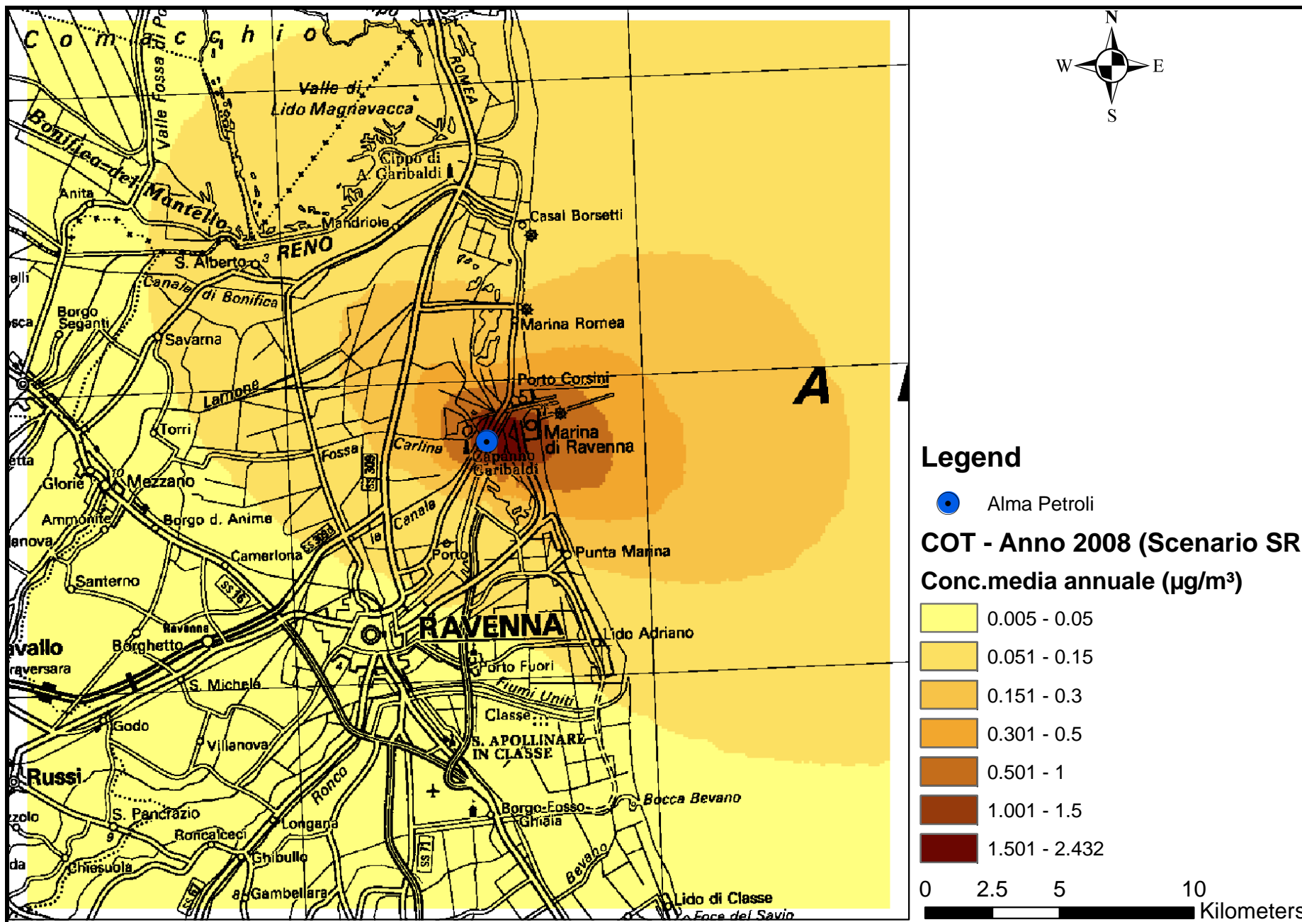
Mappa 29 - Concentrazione massima su media annua – CALPUFF – COT- SCENARIO REALE – Anno 2008
