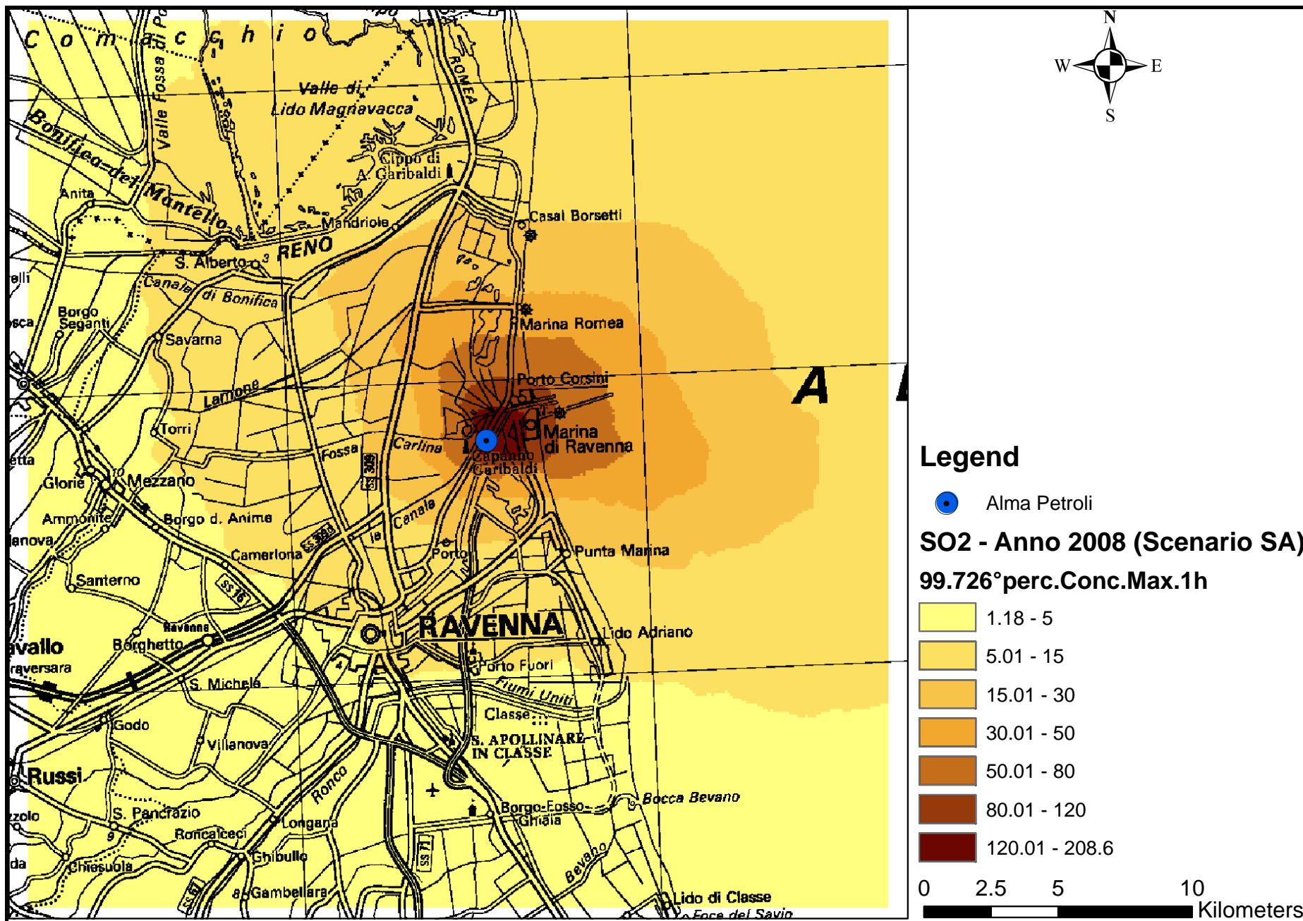
Mapa 19 - 99,726° percentile Concentrazione massima su media oraria – CALPUFF – SO x - SCENARIO AUTORIZZATO – Anno 2008
