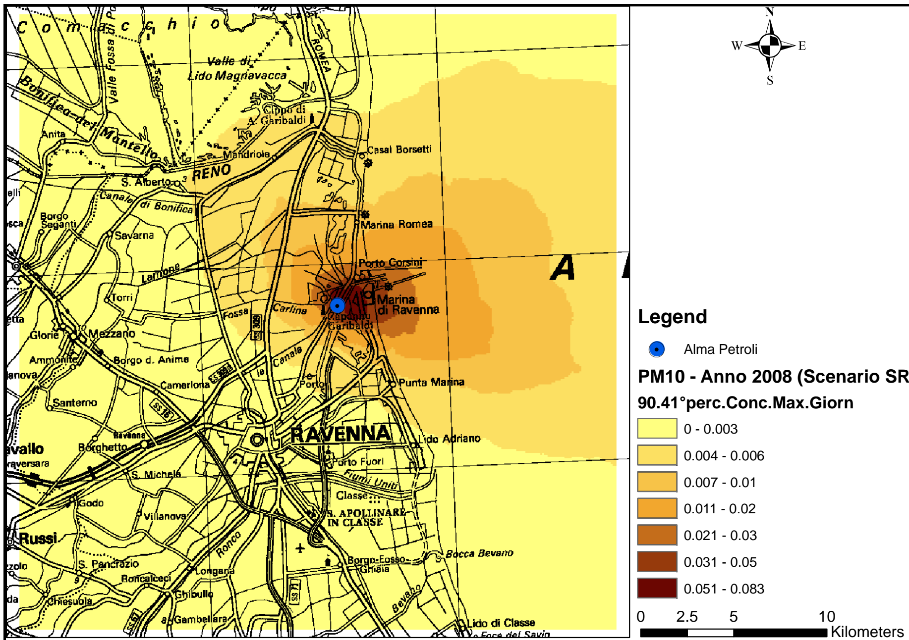
Mapa 39 - 90,41° percentile Concentrazione massima su media giornaliera – CALPUFF – PM10- SCENARIO REALE – Anno 2008
