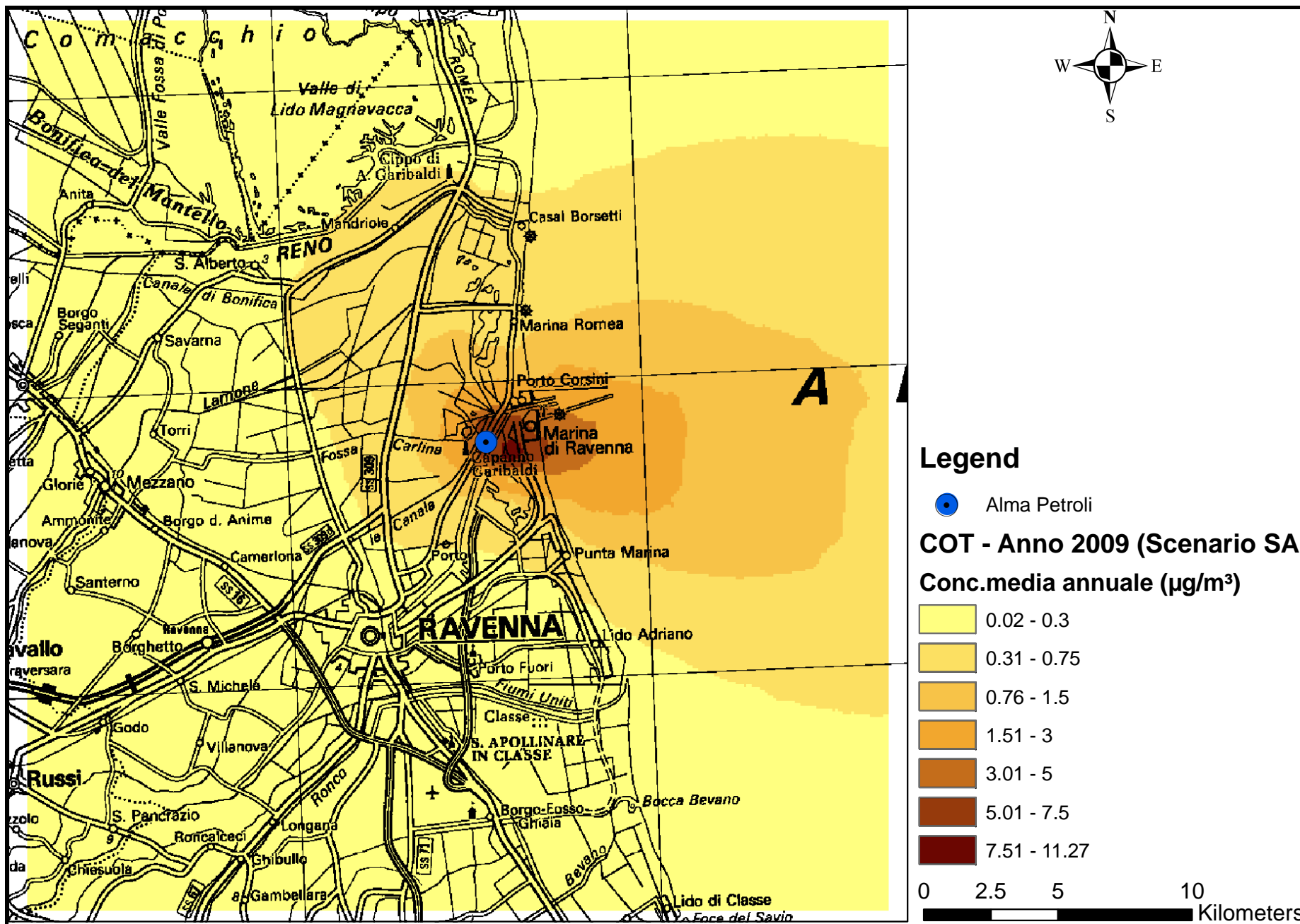
Mappa 6- Concentrazione massima su media annua – CALPUFF – COT- SCENARIO AUTORIZZATO – Anno 2009
