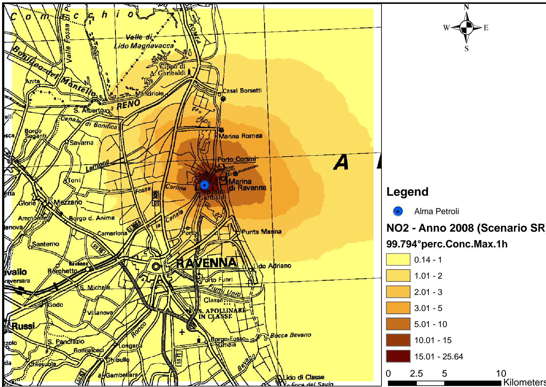
Mapa 35 - 99,794° percentile Concentrazione massima su media oraria – CALPUFF – NOx- SCENARIO REALE – Anno 2008
