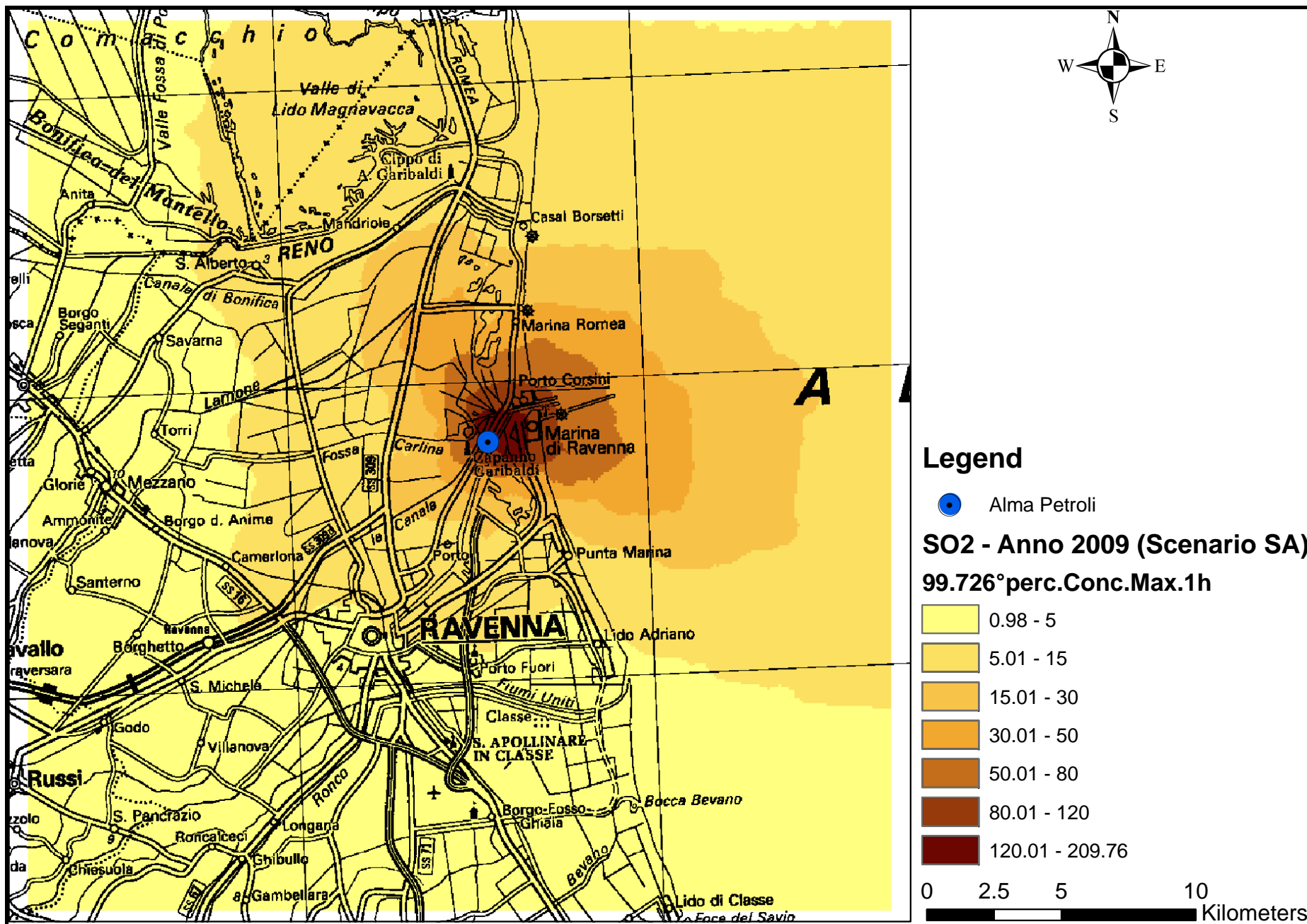
Mappa 20 - 99,726° percentile Concentrazione massima su media oraria – CALPUFF – SO x - SCENARIO AUTORIZZATO – Anno 2009
