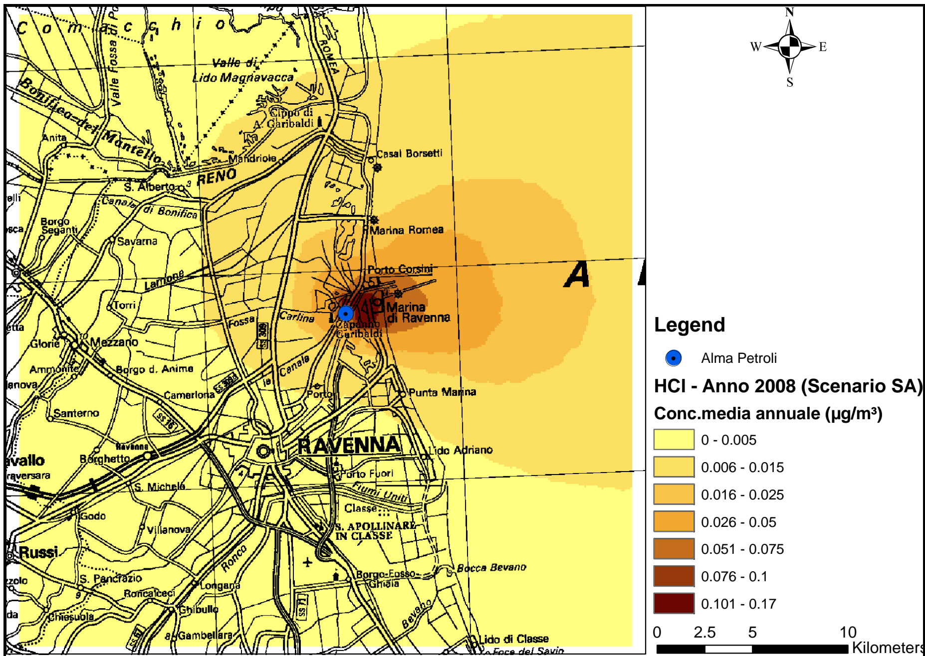
Mappa 9- Concentrazione massima su media annua – CALPUFF – HCL- SCENARIO AUTORIZZATO – Anno 2008
