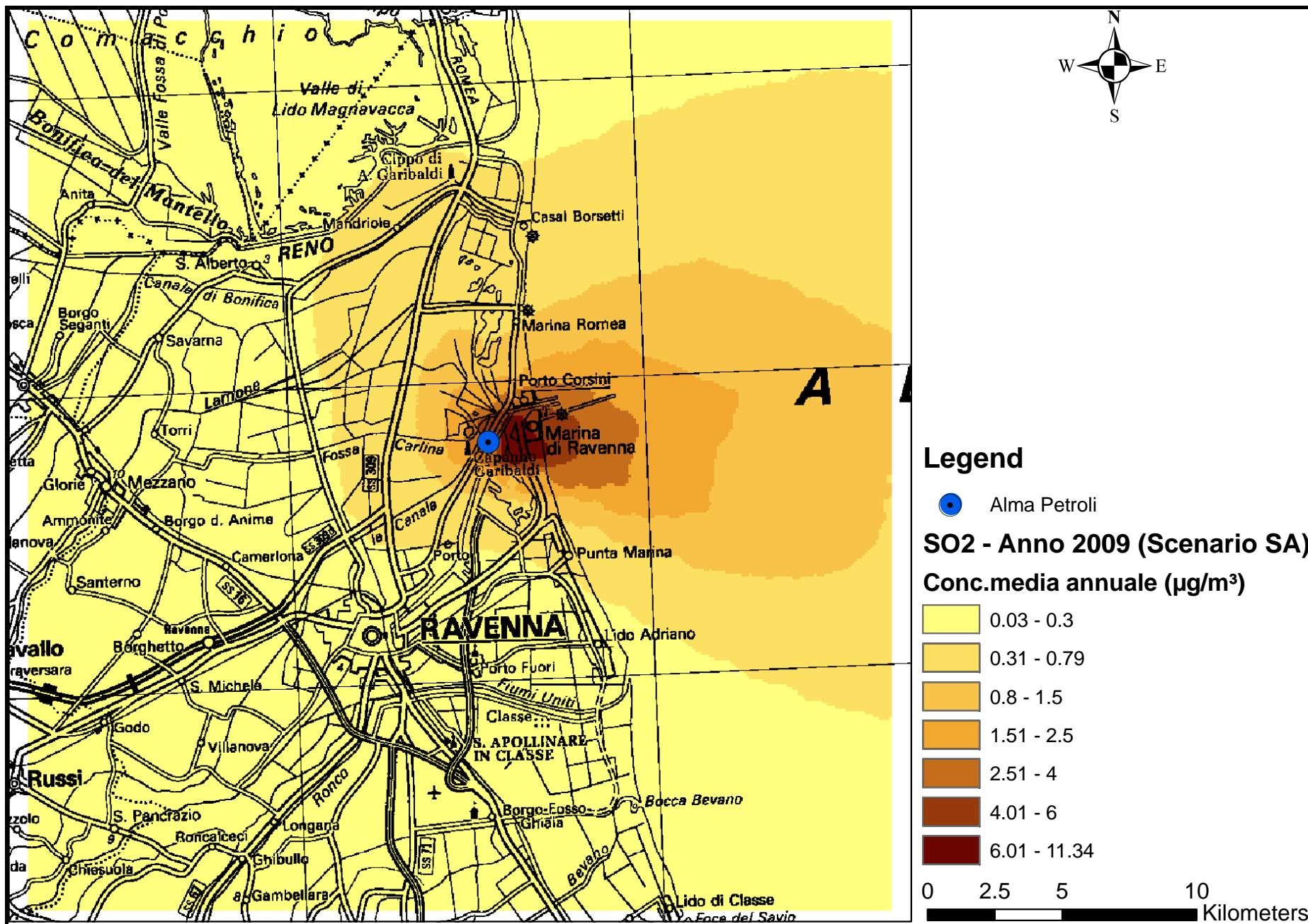
Mapa 24 - Concentrazione massima su media annua - CALPUFF - SO x - SCENARIO AUTORIZZATO - Anno 2009
