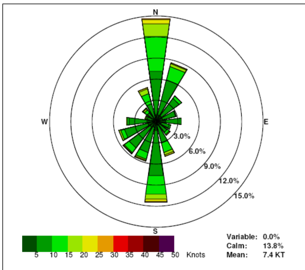
Figura 4: Rosa dei venti. Stazione n. 163240 (Periodo 1995÷2005). (Fonte dei dati NCDC).
