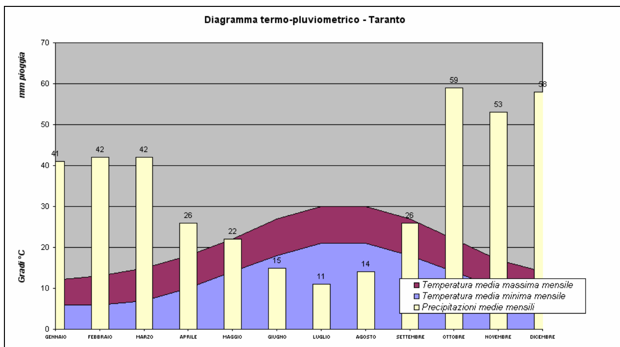
Figura 3- Diagramma termo-pluviometrico periodo 1995-2005 (Fonte: National Climatic Data Center stazione Taranto Grottaglie (TA) (lat. 40.517° N, long 17.4° E, Quota s.l.m.: 69 m, n.ID staz 163240), Elaborazione ENSR Italia).
