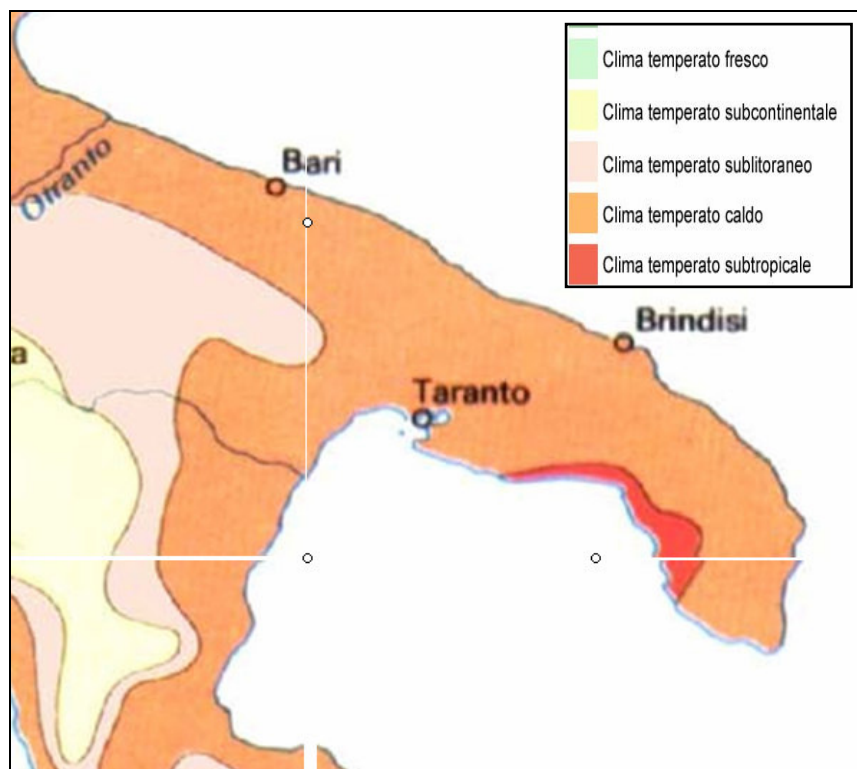
Figura 2- Classificazione climatica dell'area vasta d'interesse (Fonte: Stralcio dalla Carta Climatica elaborata da Wladimir Koppen, 1961)
