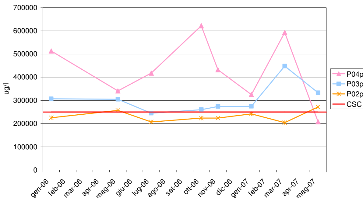
Solfati - falda profonda
