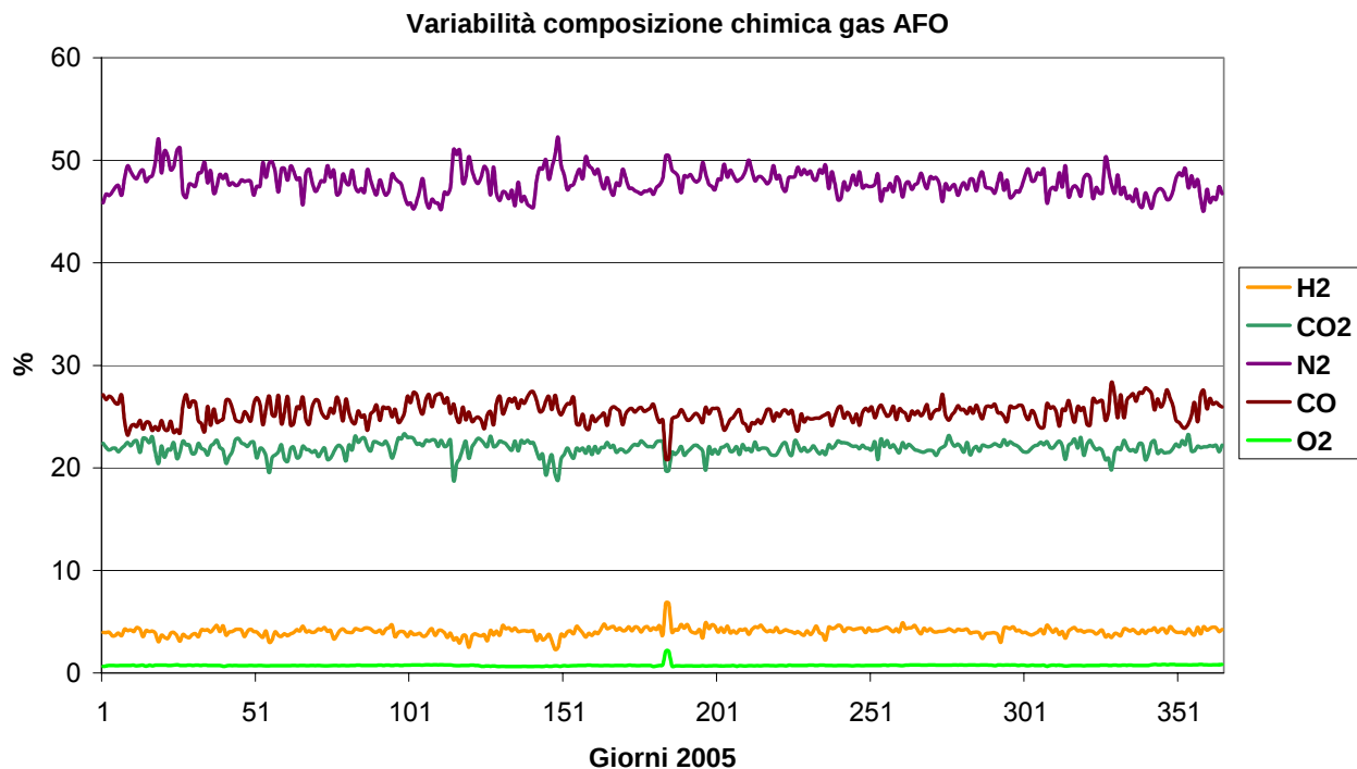
Figura 5 – Variabilità composizione chimica Gas AFO – anno 2005
