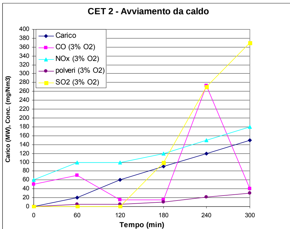
Figura 33 – CET2 – Avviamento da caldo
