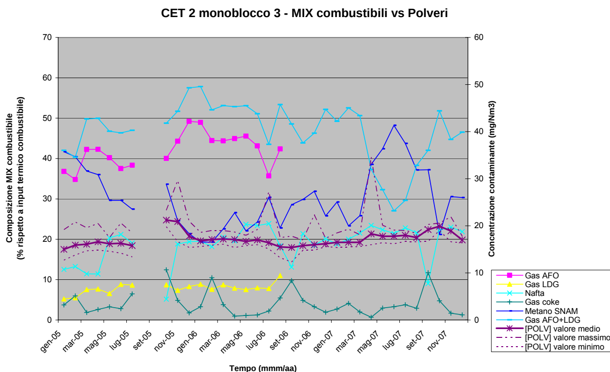
Figura 28 – CET2 – Monoblocco 3 – Mix combustibili Vs. emissioni Polveri
