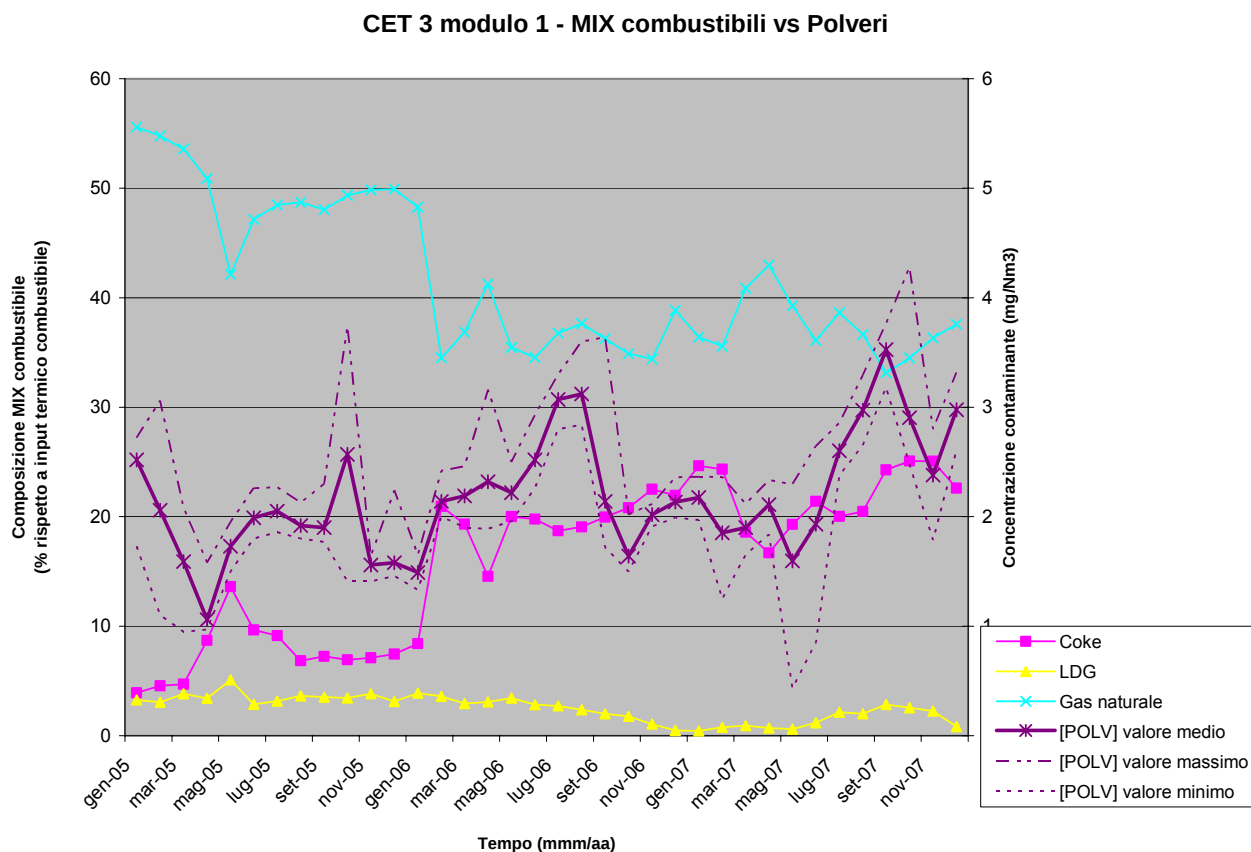
Figura 29 – CET3 – Modulo 1 – Mix combustibili Vs. emissioni Polveri
