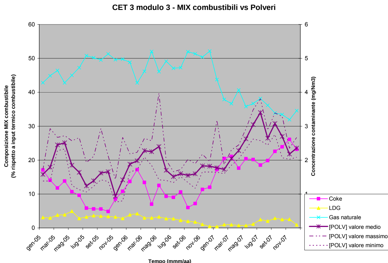
Figura 31 – CET3 – Modulo 3 – Mix combustibili Vs. emissioni Polveri
