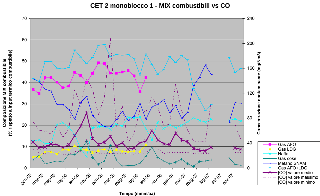
Figura 20 – CET2 – Monoblocco 1 – Mix combustibili Vs. emissioni CO
