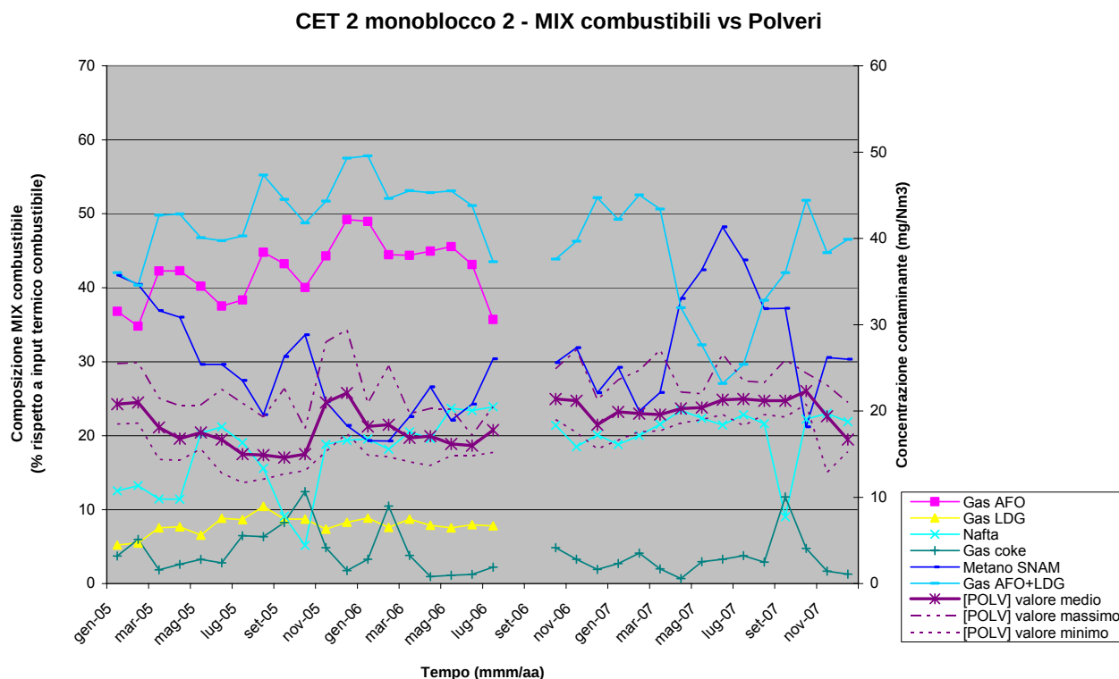
Figura 27 – CET2 – Monoblocco 2 – Mix combustibili Vs. emissioni Polveri
