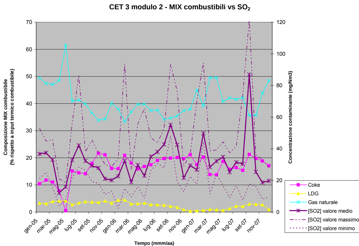
Figura 12 – CET3 – Modulo 2 – Mix combustibili Vs. emissioni SO 2
