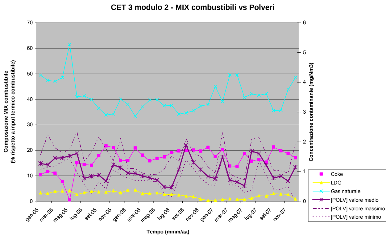
Figura 30 – CET3 – Modulo 2 – Mix combustibili Vs. emissioni Polveri
