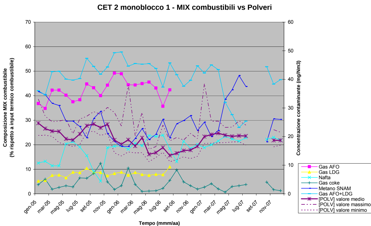
Figura 26 – CET2 – Monoblocco 1 – Mix combustibili Vs. emissioni Polveri
