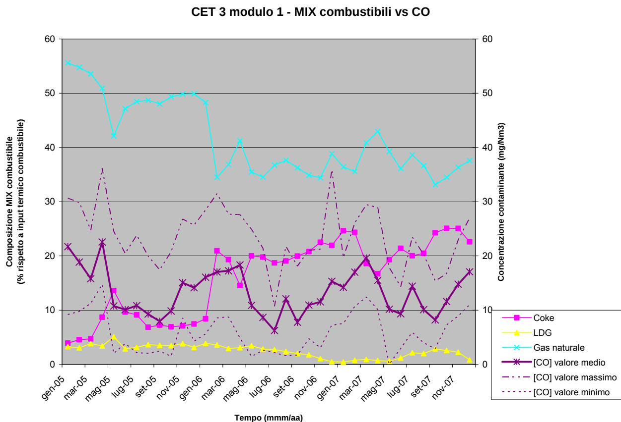
Figura 23 – CET3 – Modulo 1 – Mix combustibili Vs. emissioni CO
