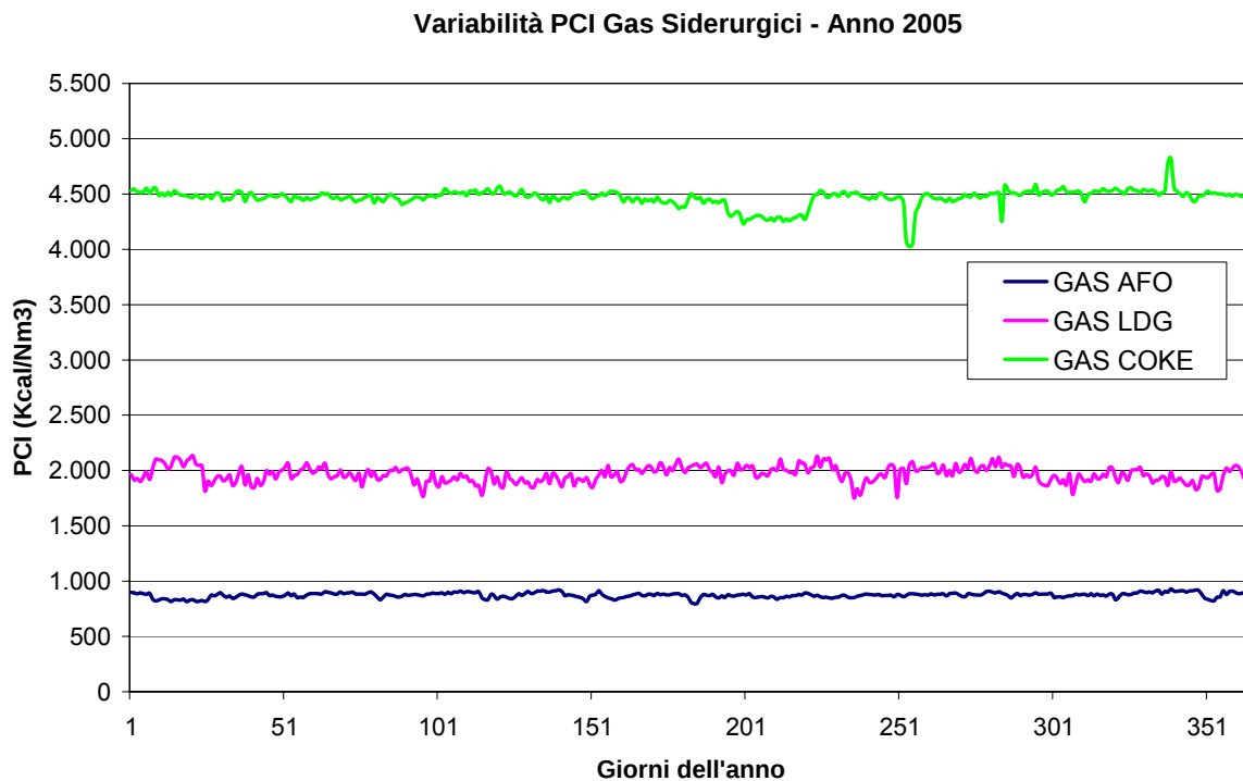
Figura 4 – Variabilità PCI Gas Siderurgici in ingresso – anno 2005
