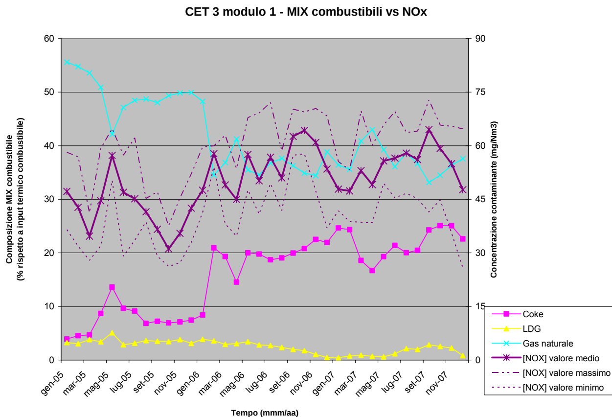
Figura 17 – CET3 – Modulo 1 – Mix combustibili Vs. emissioni NOx
