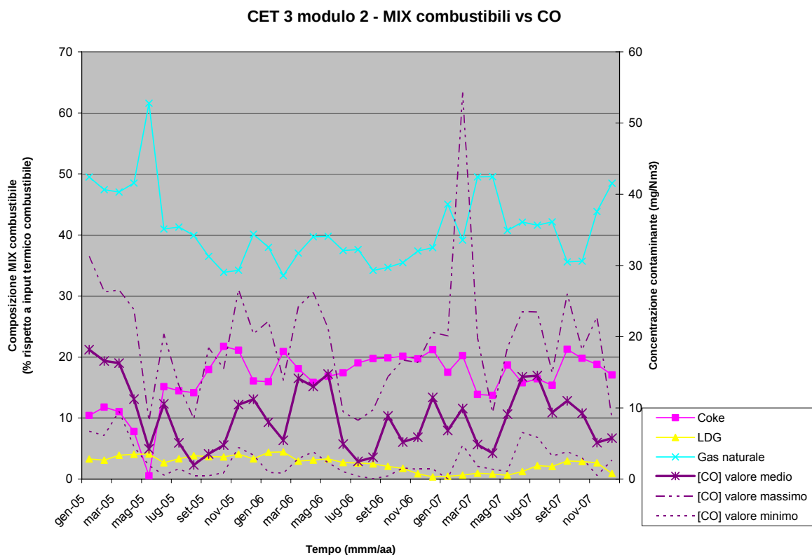
Figura 24 – CET3 – Modulo 2 – Mix combustibili Vs. emissioni CO
