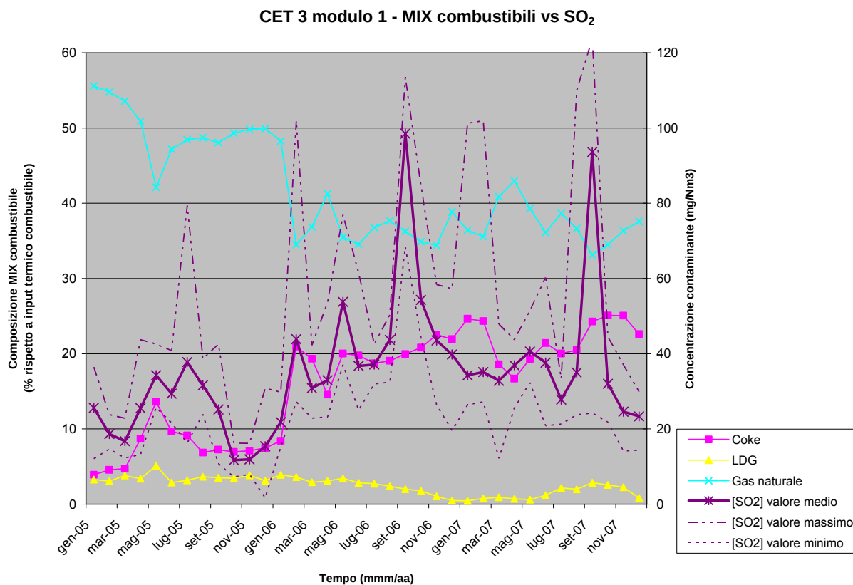
Figura 11 – CET3 – Modulo 1 – Mix combustibili Vs. emissioni SO 2
