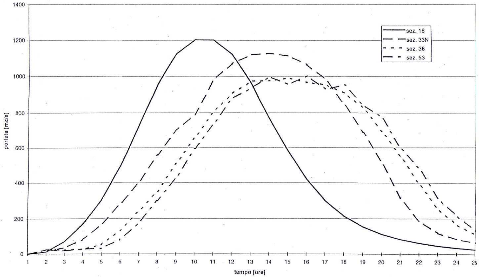
Fiume Cornia - Idrogrammi di progetto tempo di ritorno 200 anni
