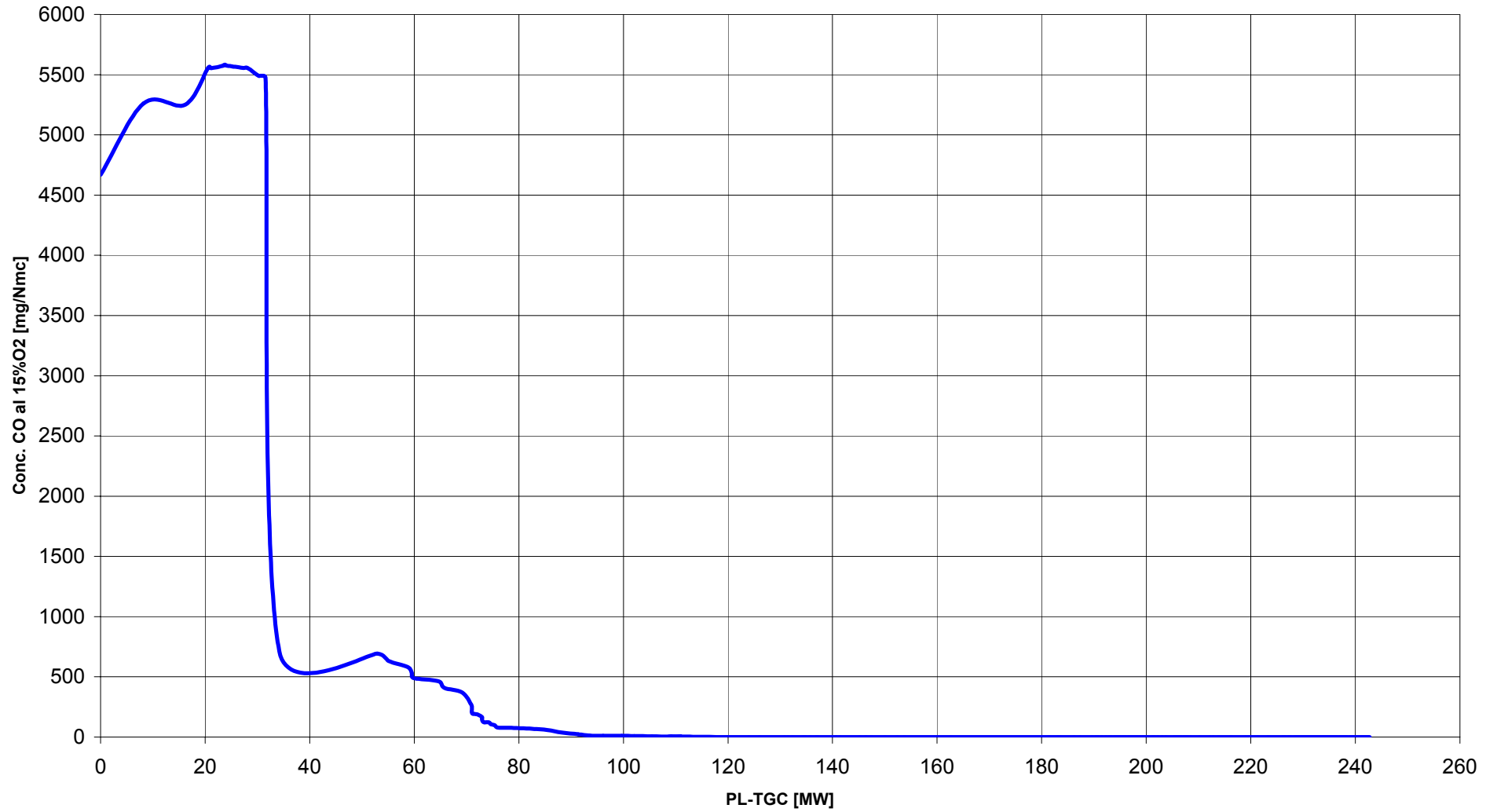
OS2 - Andamento Concentrazione CO al 15% O2 in funzione della potenza erogata TGC - D.L.N. 2.6
