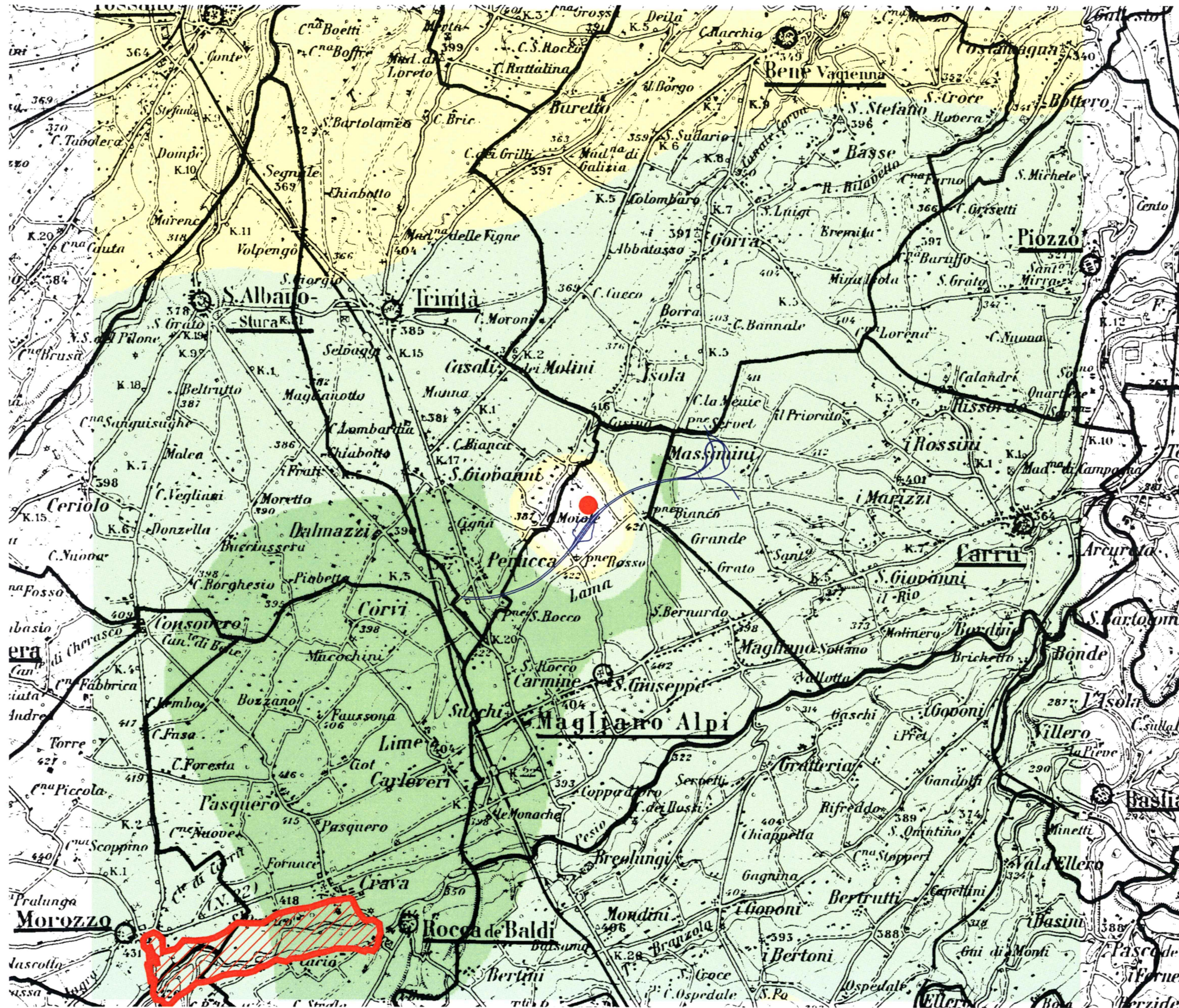
Figura D6.1.2b Concentrazioni Medie Annuie di NOx (15 x 15 km) - Scenario B - (Scala 1:60.000)
