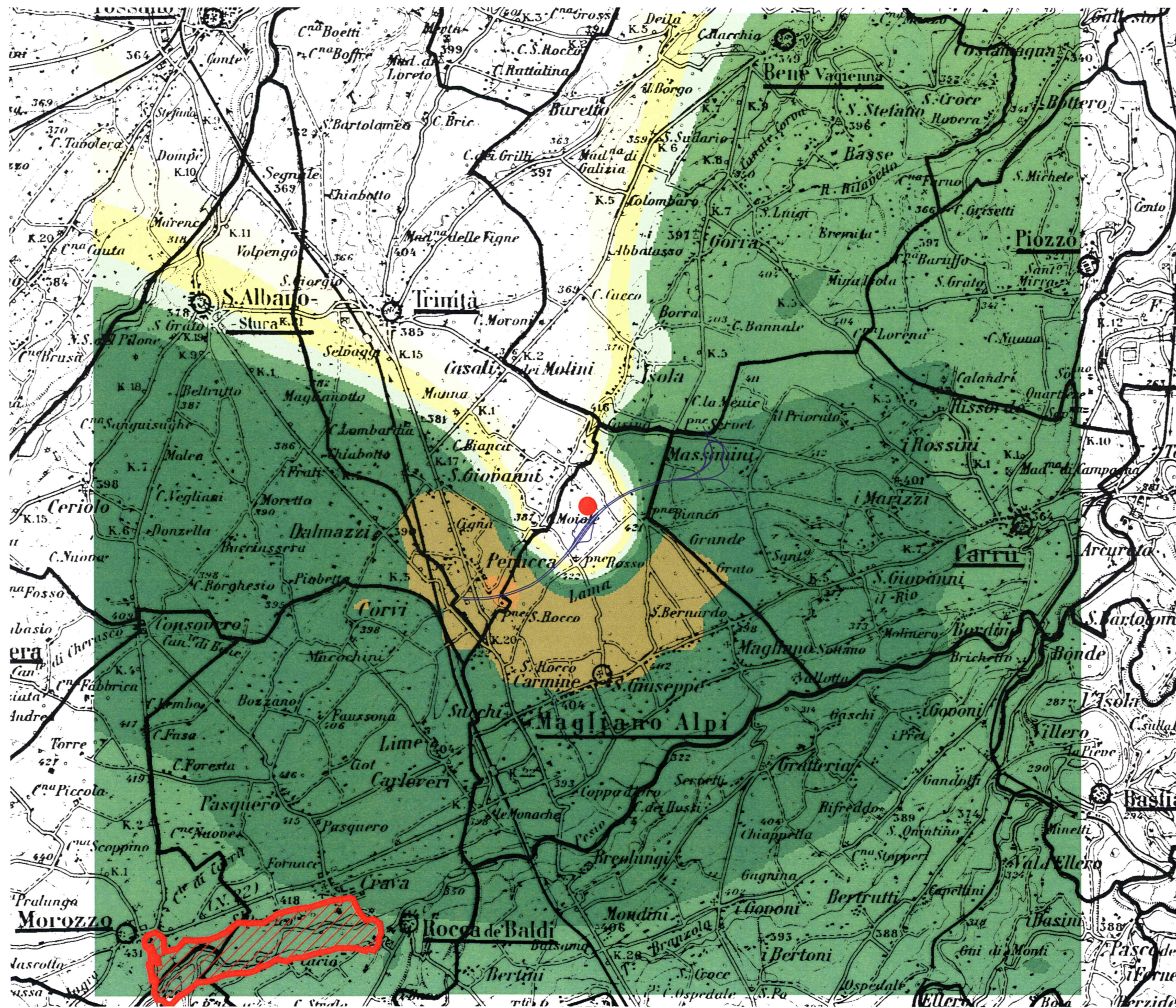
Figura D6.1.3c 99,8° Percentile delle Concentrazioni Medie Orarie di NOx (15 x 15 km) - Scenario B - (Scala 1:60.000)
