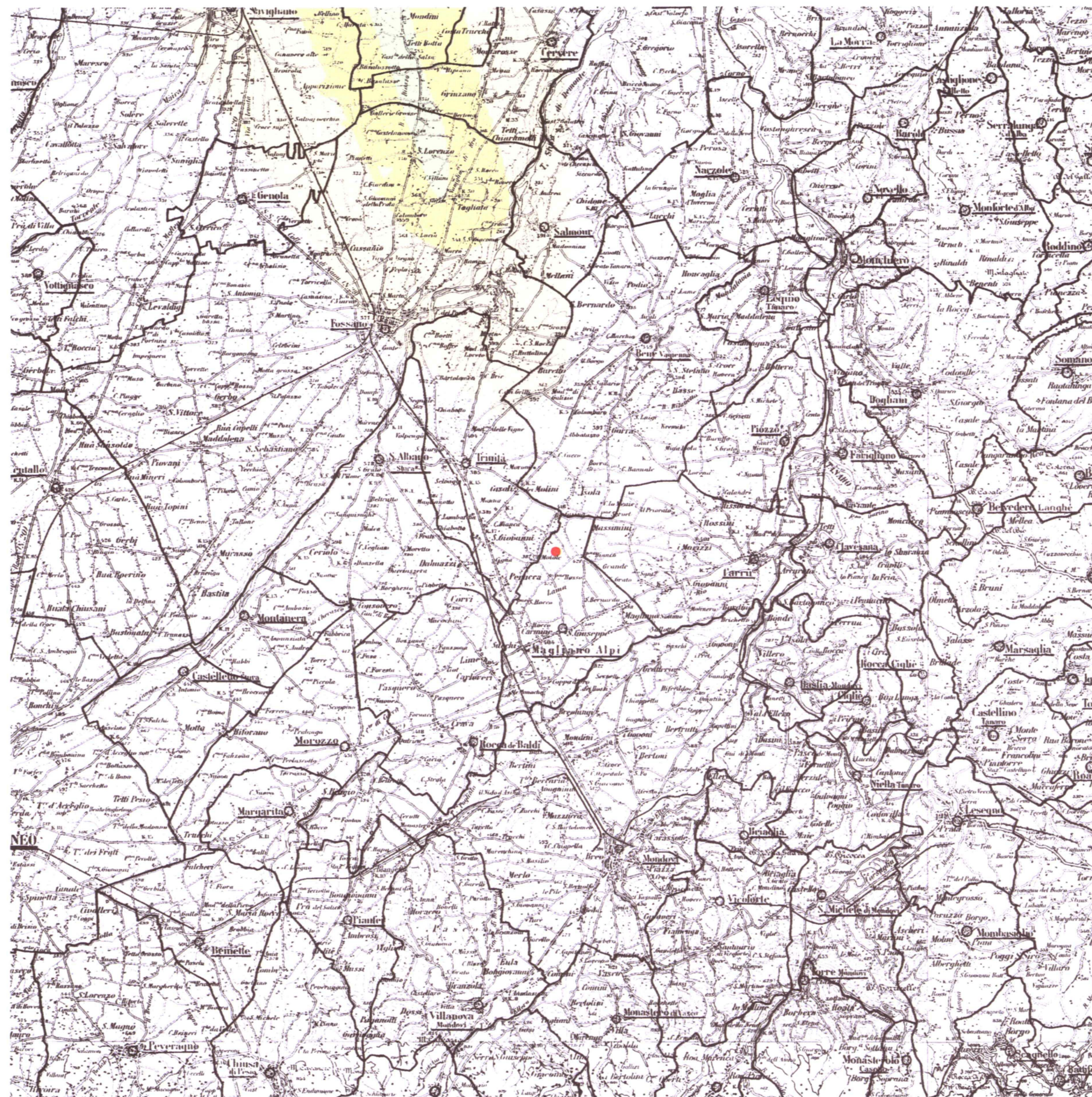
Figura D6.1.4d Concentrazione al Suolo di NOx a Mezzogiorno del 09/01/2002 (Scala 1:150.000) - (7 di 13)
