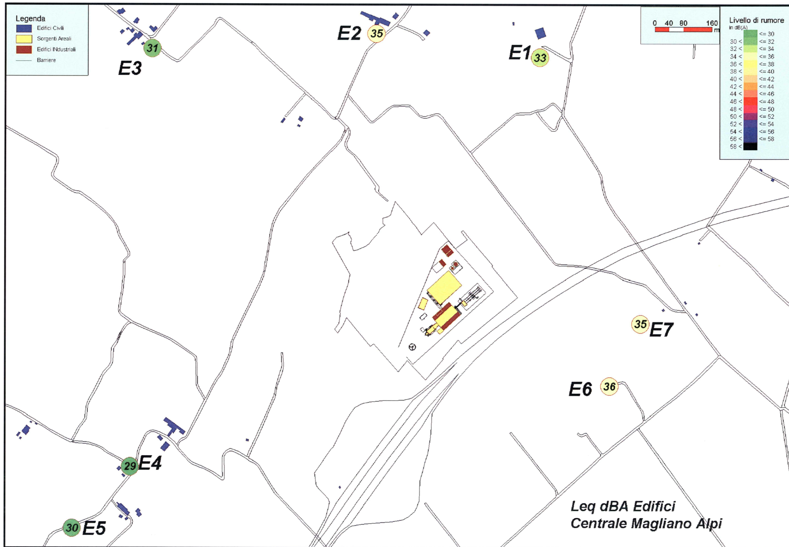
Figura B24.2a Livello Equivalente Massimo Indotto dall'Esercizio della Centrale Presso le Abitazioni Limitrofe all'Impianto
