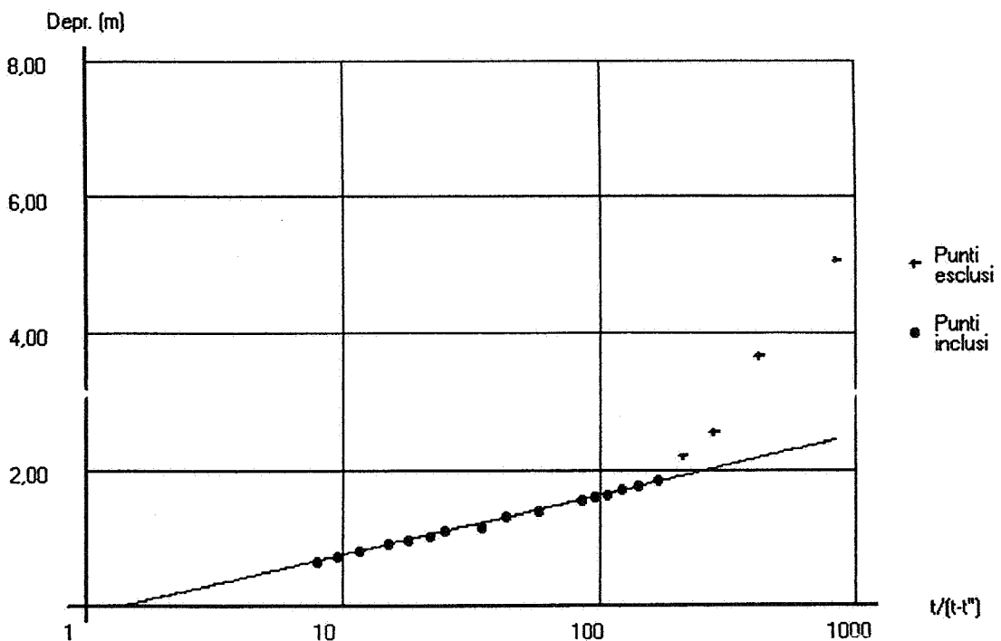
CALCOLO IN FASE DI RISALITA CON IL METODO DI COOPER - JACOB Nota Bene: S stimato considerando S" come ultimo dato in fase di discesa
