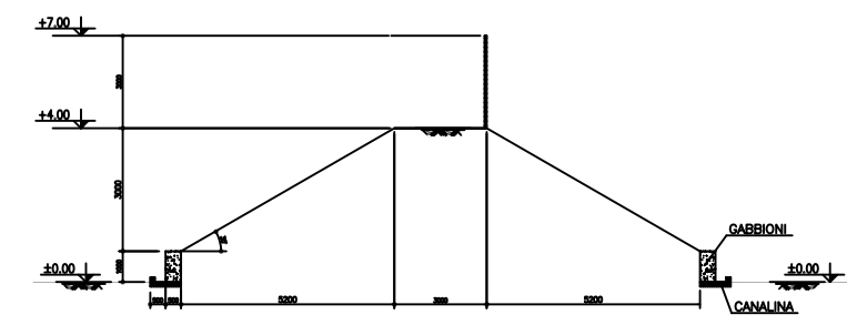
SEZIONE 1-1
