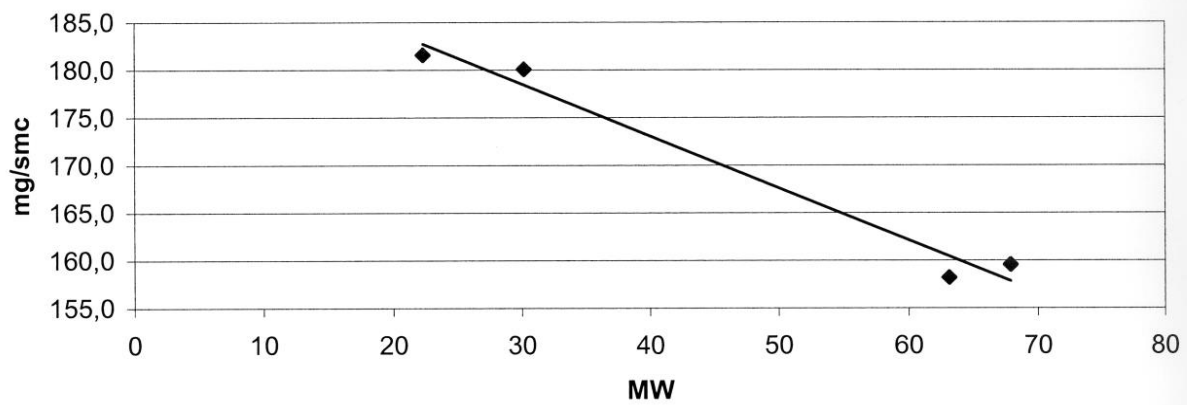
Fig. 2 - Andamento NOx in variazione di carico
