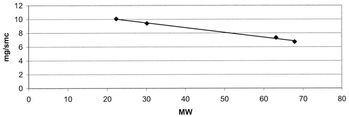
Fig. 1 - Andamento CO in variazione di carico
