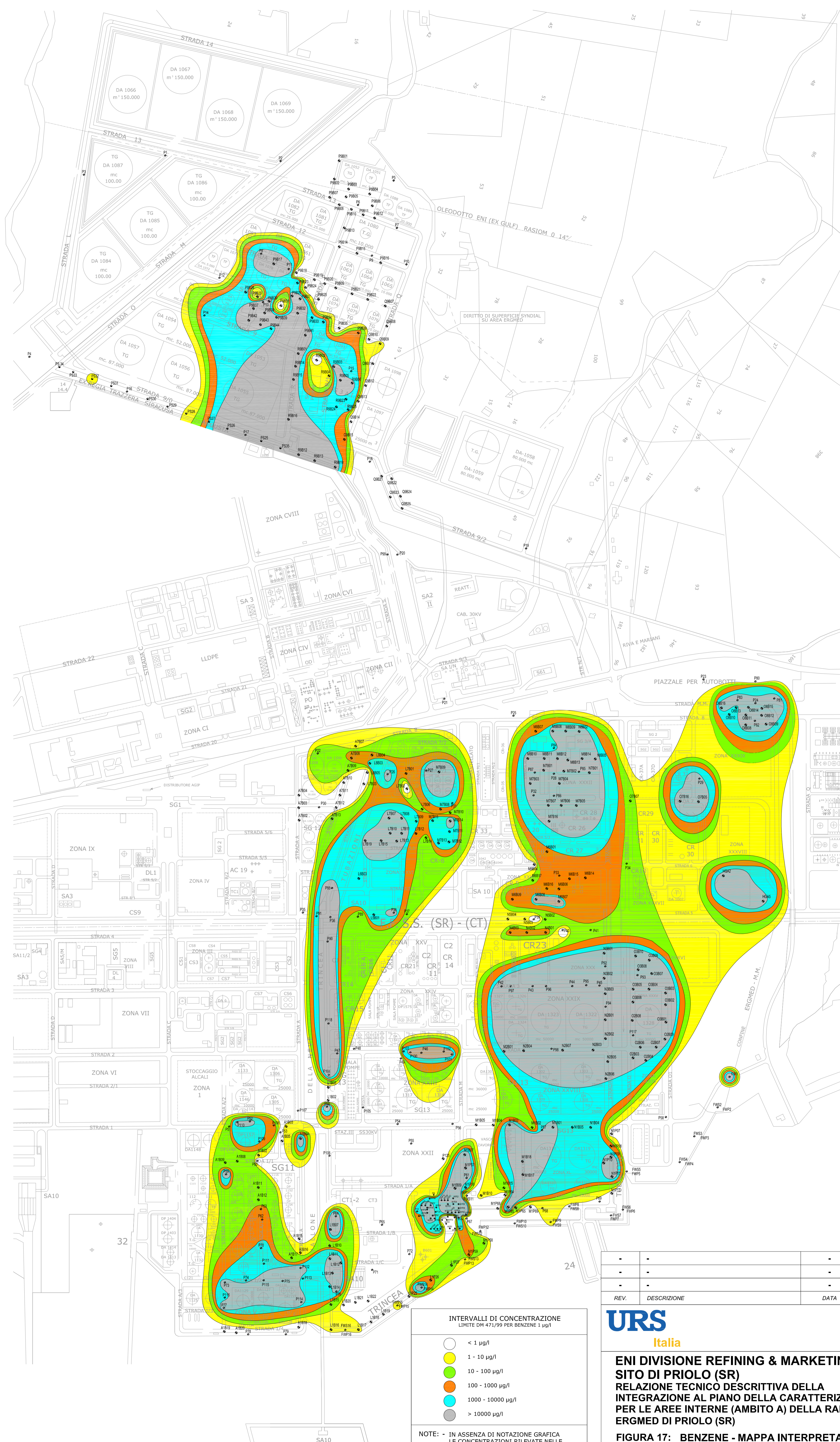
FIGURA 17: PRIOLO - MAPPA INTERPRETATIVA DELLA CONTAMINAZIONE DELLE ACQUE
