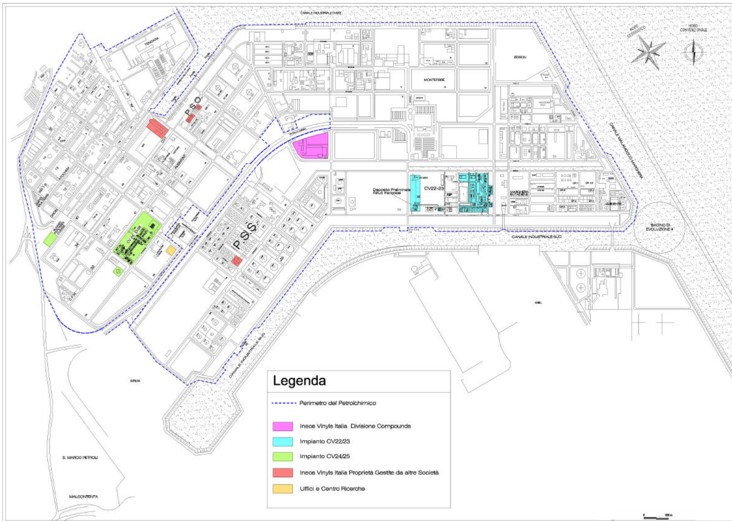
Figura 1 - Planimetria del sito petrolchimico di Porto Marghera con ubicazione degli impianti INEOS Vinyls
