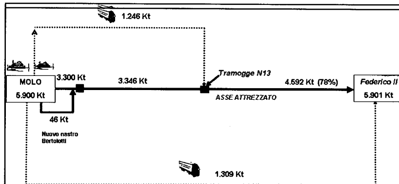
Figura 5.5 – Flussi carbone da molo a centrale Federico II - anno 2006
