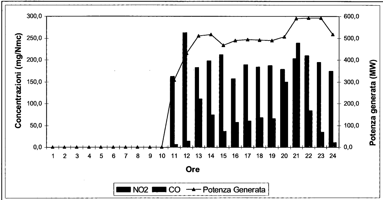
Figura 5-a – Indicazione delle variazioni della concentrazione di \text{NO}_{2\text{equivalente}} e CO al variare del carico
