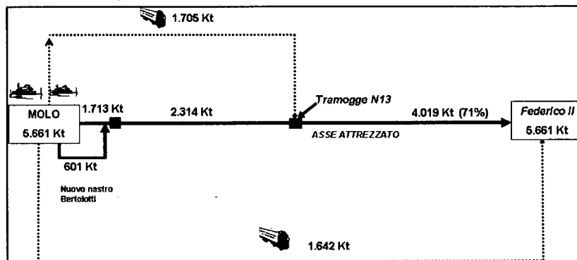
Figura 5.6 – Flussi carbone da molo a centrale Federico II - anno 2007
