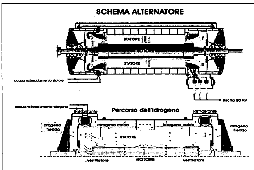
Figura 3.7 – Sezioni longitudinale dell'alternatore
