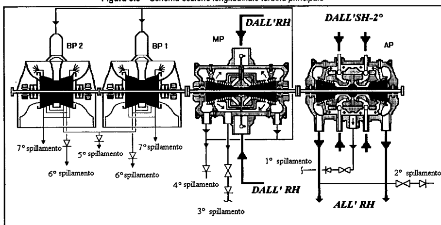
Figura 3.5 – Schema sezione longitudinale turbina principale
