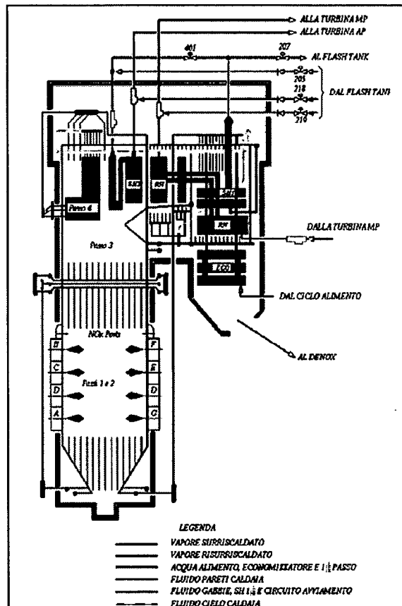
Figura 3.4 – Schema sezione longitudinale del GV
