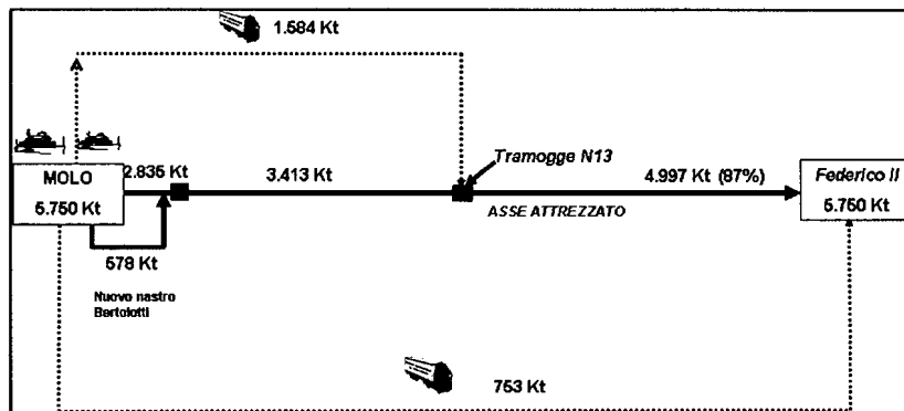
Figura 5.5 – Flussi carbone da molo a centrale Federico II - anno 2006
