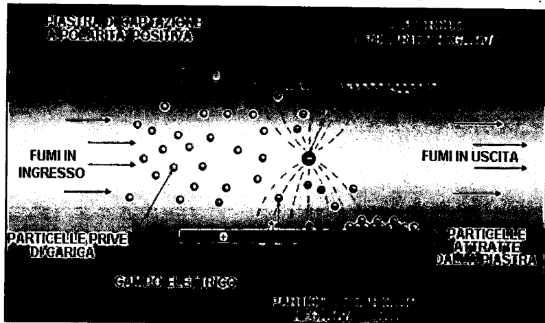
Figura 4.D.1 – Schema principio di funzionamento degli elettrofiltri
