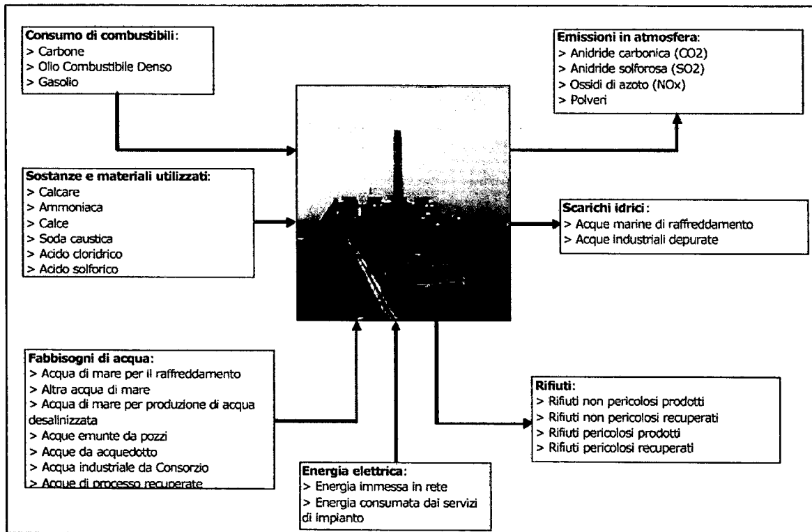
Figura 5.1 – Schema per i bilanci di centrale
