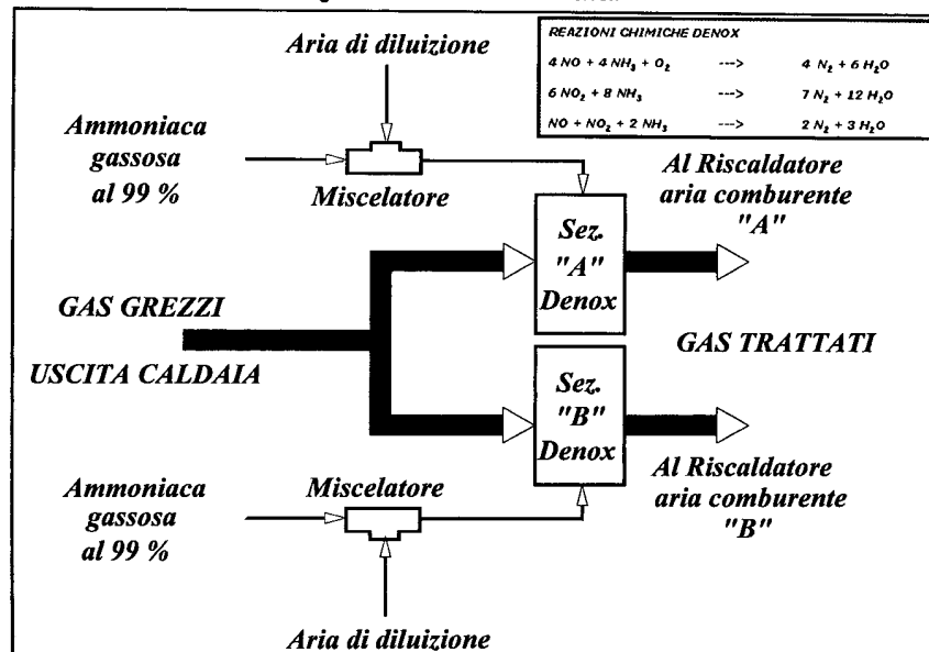
Figura 4.C.1 – Schema reattori DeNOx
