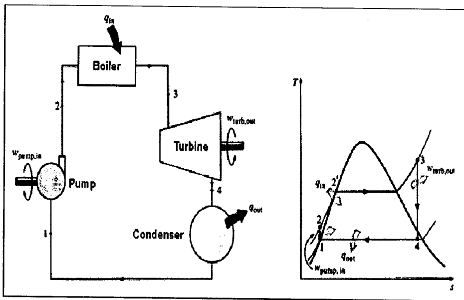
Figura 3.1 – Schema impianto a vapore e ciclo termodinamico
