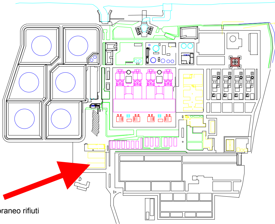
Planimetria generale
